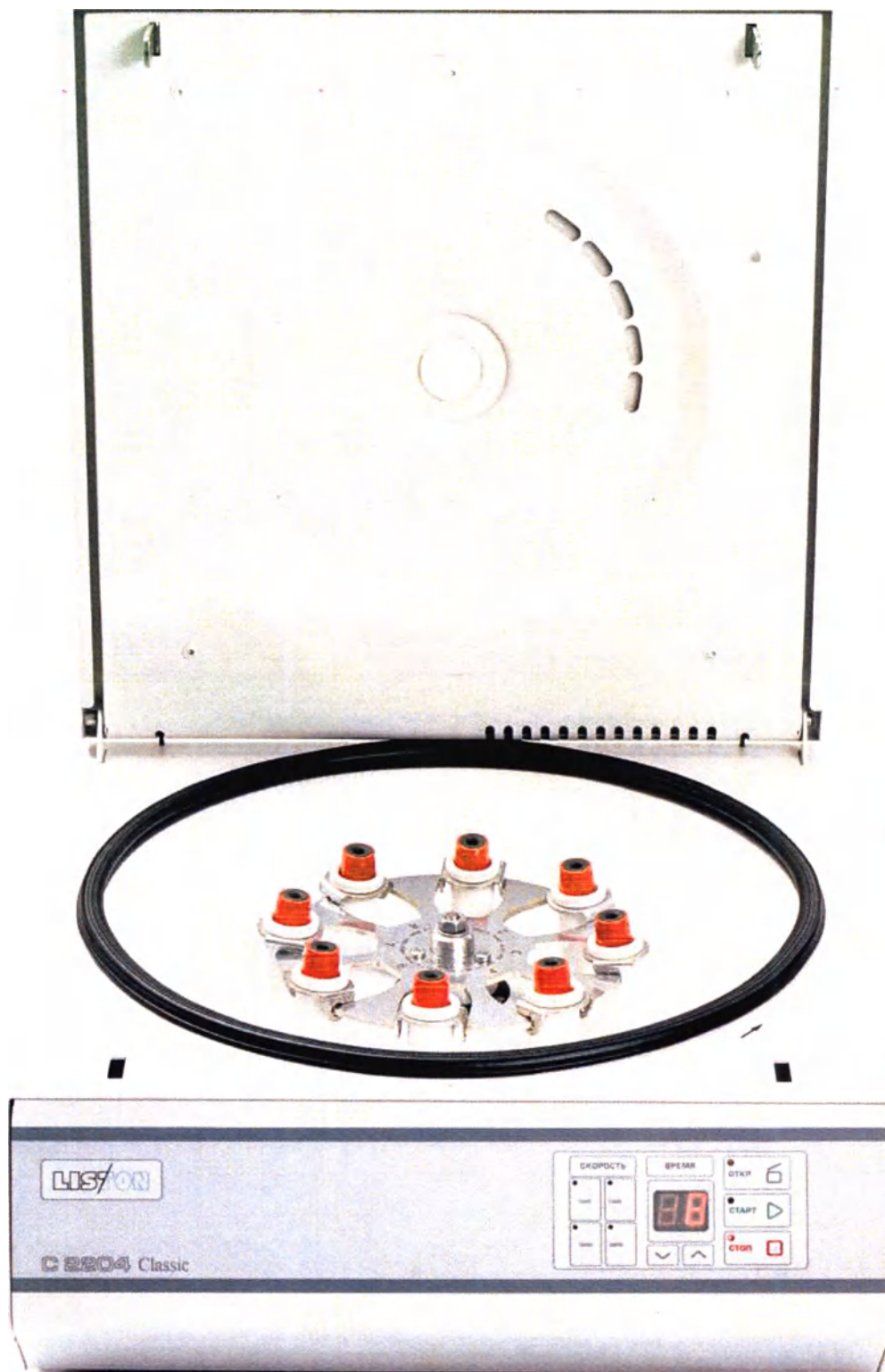
Центрифуга Liston C 2204 Classic. Вид с открытой крышкой.
