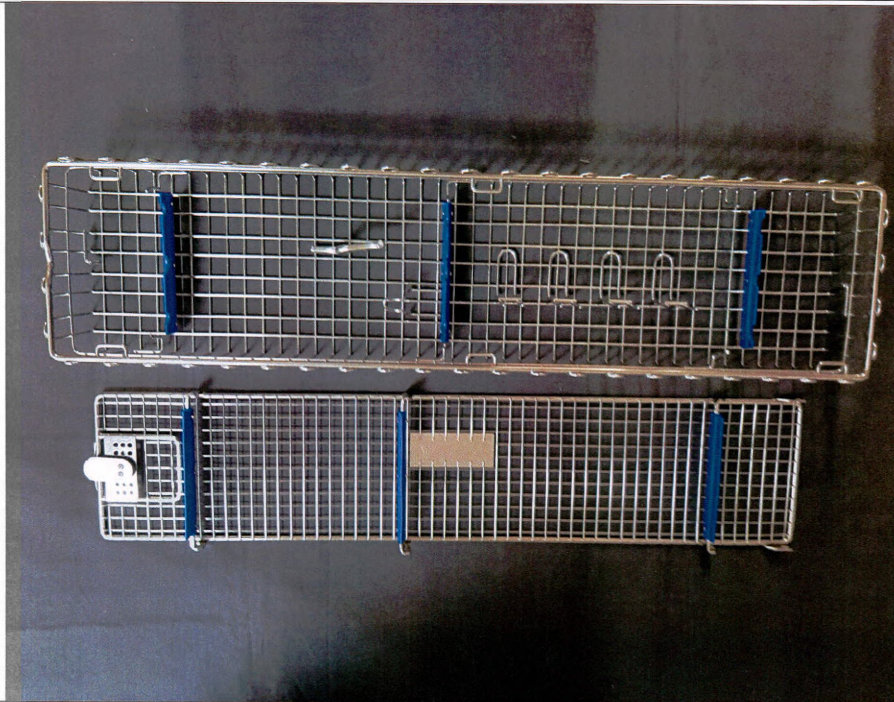
Рис. 41. Контейнер проволочный для дезинфекции/стерилизации/хранения, размеры: 622 x 150 x 78 мм.
