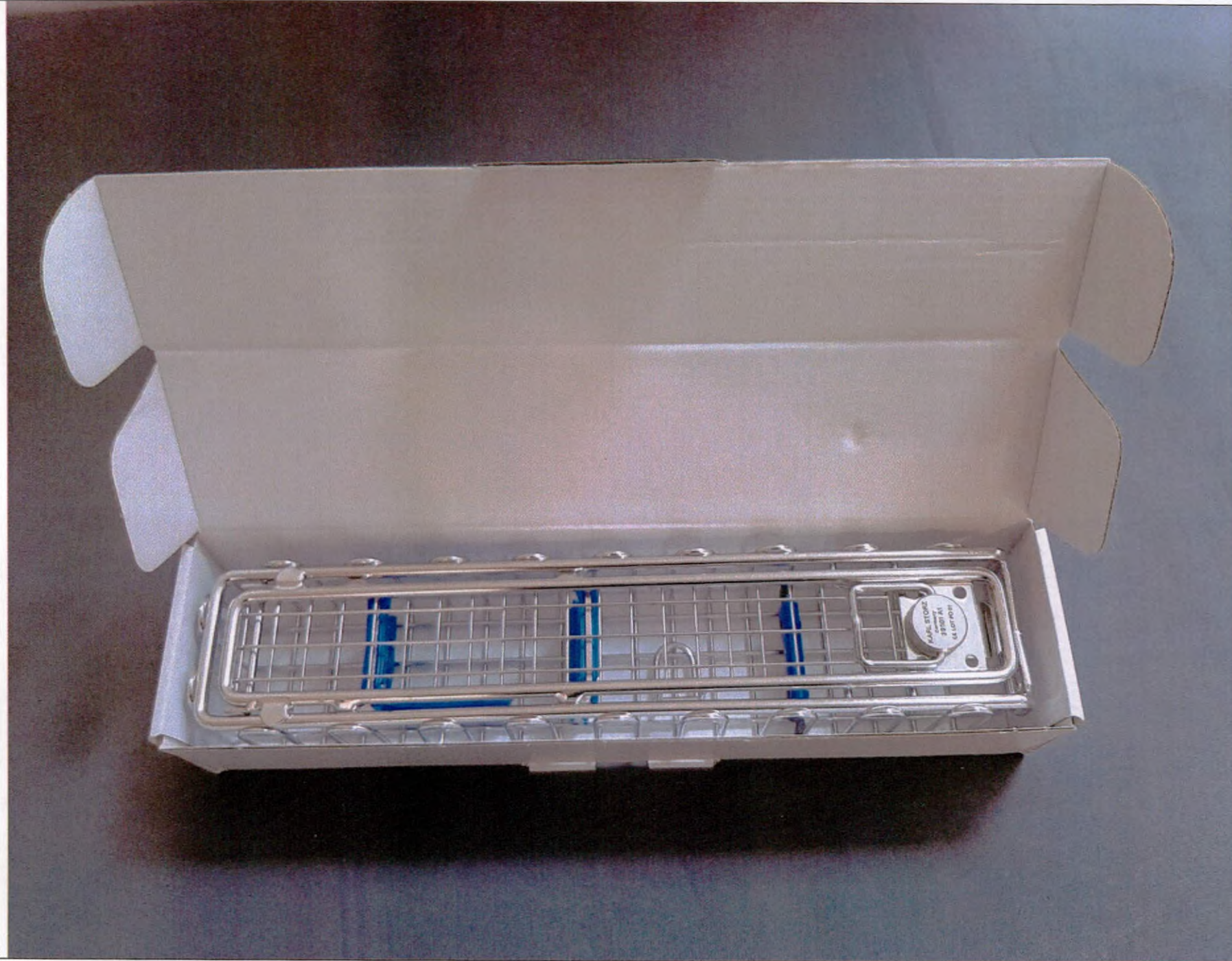
Рис. 19. Контейнер проволочный для дезинфекции/стерилизации/хранения, размеры: 290 x 60 x 52 мм.
