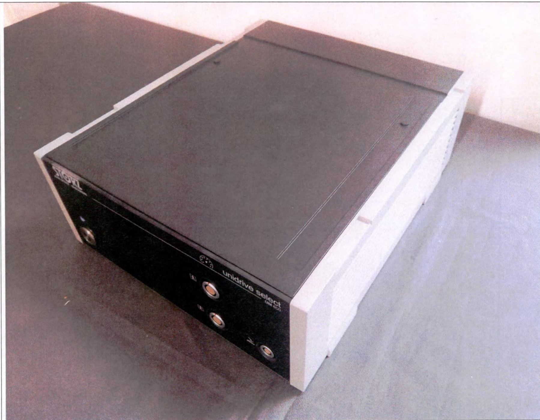
Рис. 5. Аппарат UNIDRIVE SELECT
