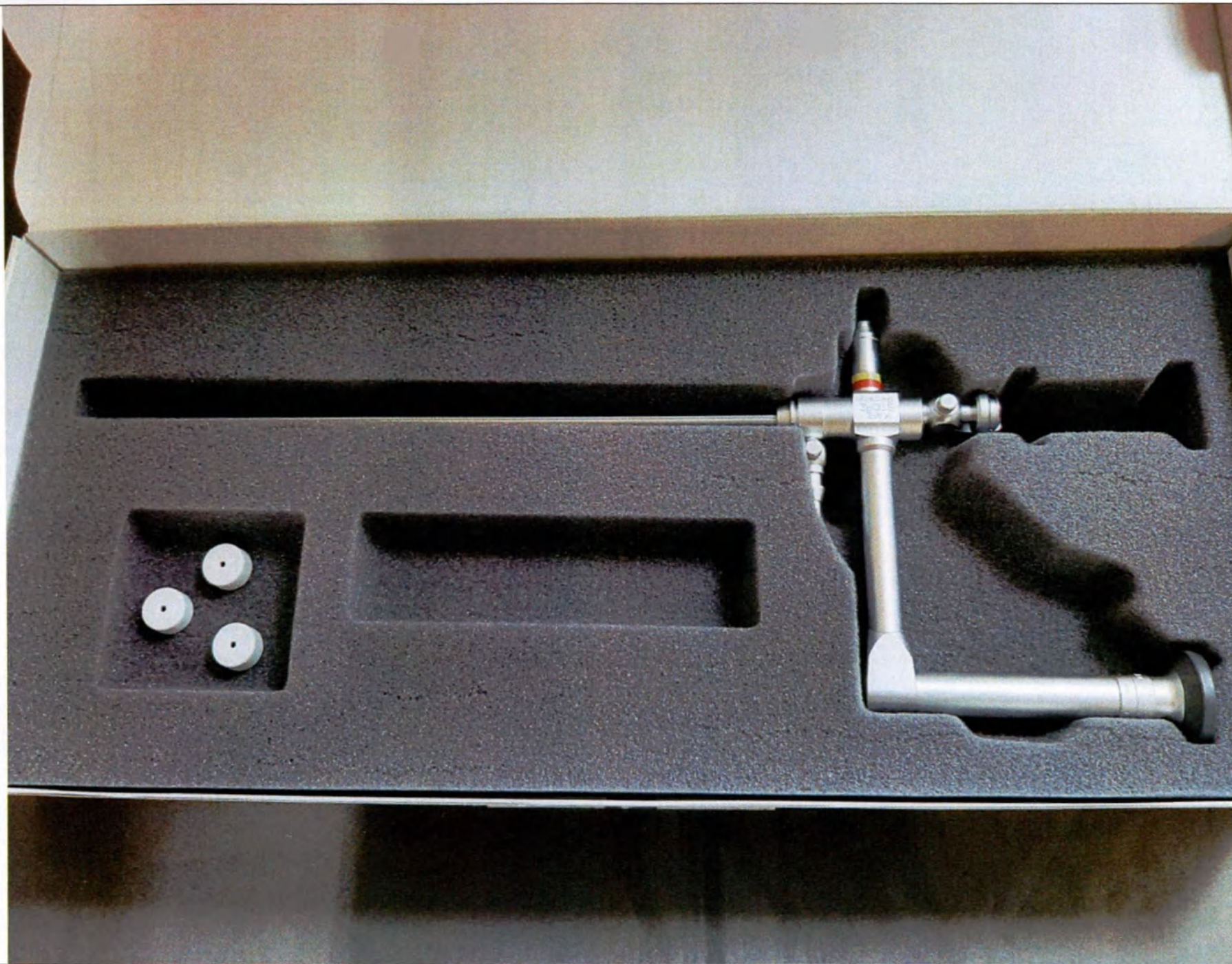
Рис. 5. Нефроскоп жесткий HOPKINS с параллельным окуляром, с инструментальным каналом, типоразмер: направление наблюдения 6°, длина 25 см.
