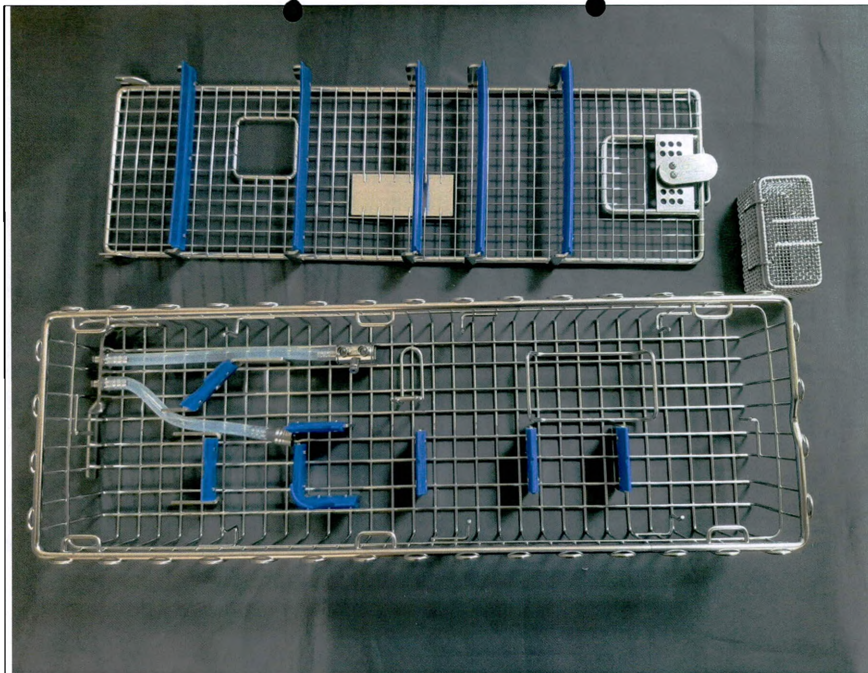
Рис. 73. Контейнер проволочный для дезинфекции/стерилизации/хранения с ячейкой для мелких деталей, размеры: 460 x 150 x 80 мм.
