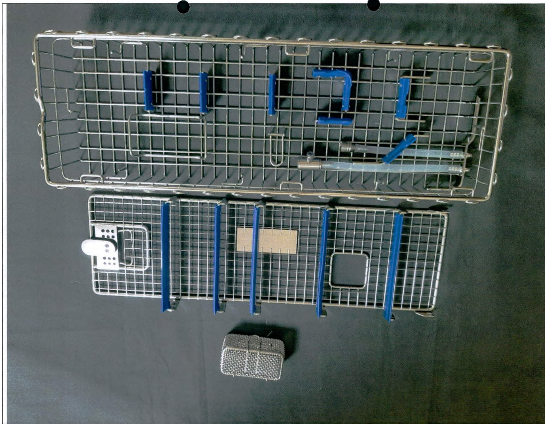
Рис. 78. Контейнер проволочный для дезинфекции/стерилизации/хранения, размеры: 460 x 150 x 87 мм.
