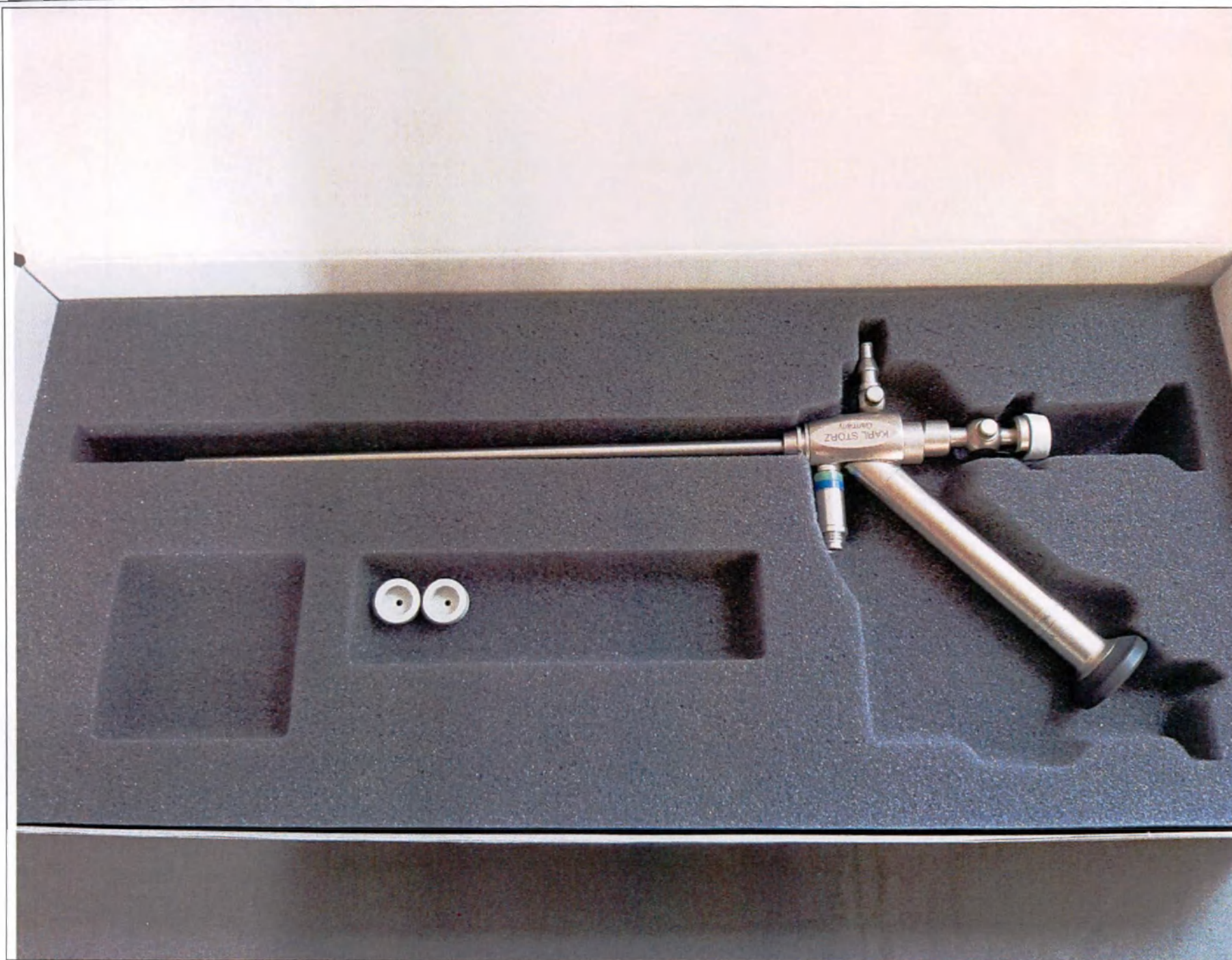
Рис. 31. Нефроскоп жесткий HOPKINS с угловым окуляром, с инструментальным каналом, типоразмер: направление наблюдения 6°, размер 18 Шр.
