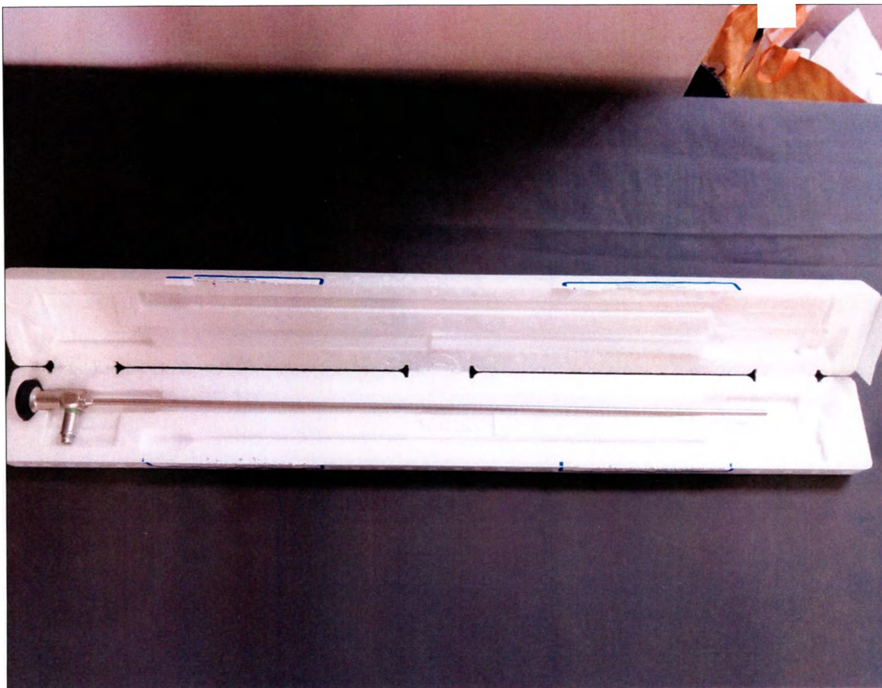
Рис. 5. Эзофагоскоп жесткий НОРКИНС (вид 144970), направление наблюдения 0^\circ , диаметр 5,5 мм, длина 53 см.
