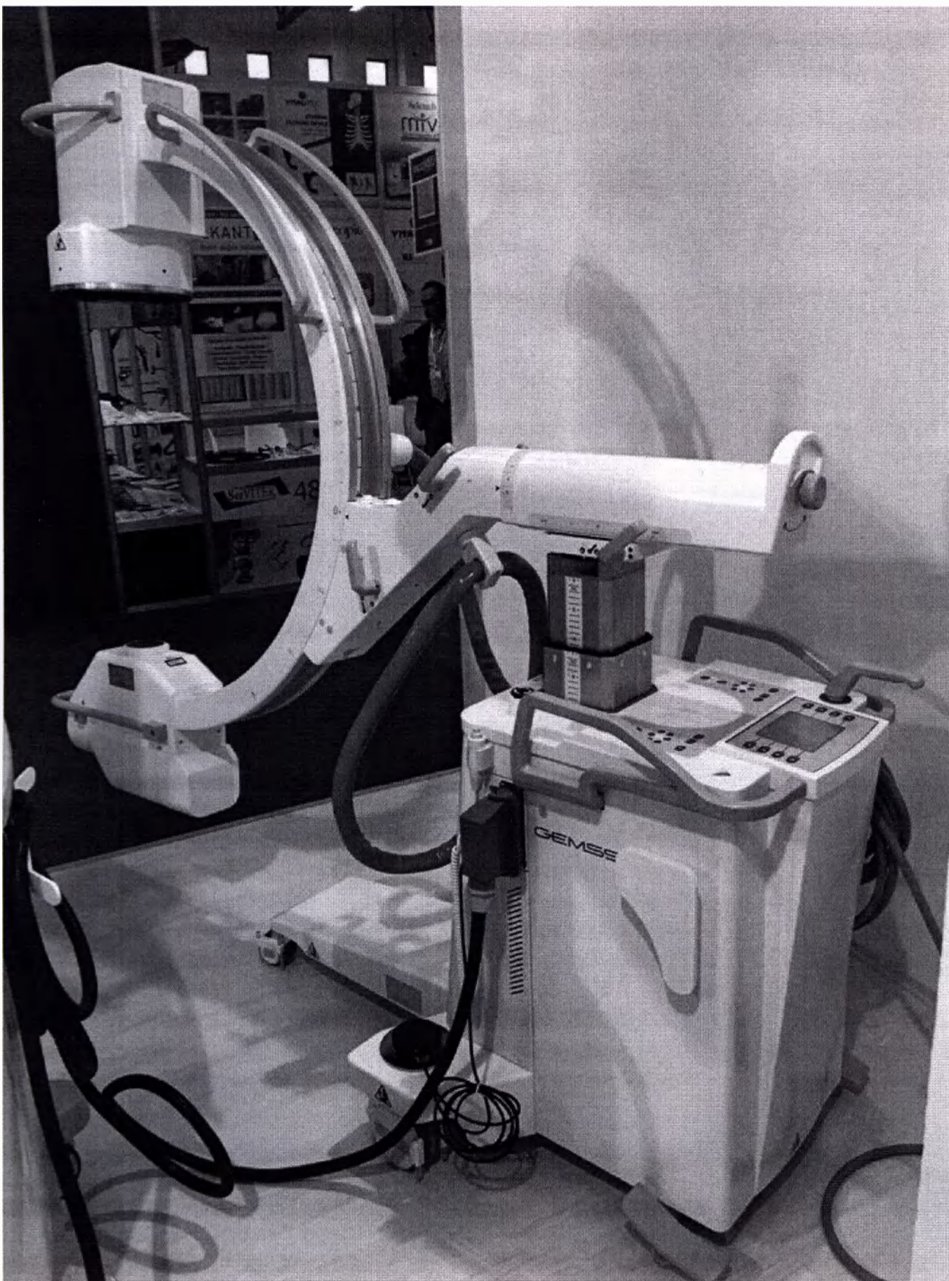
Рис. 1 - Штатив типа С-ДУГА на тележке с пультом управления, рентгеновским генератором и коллиматором
