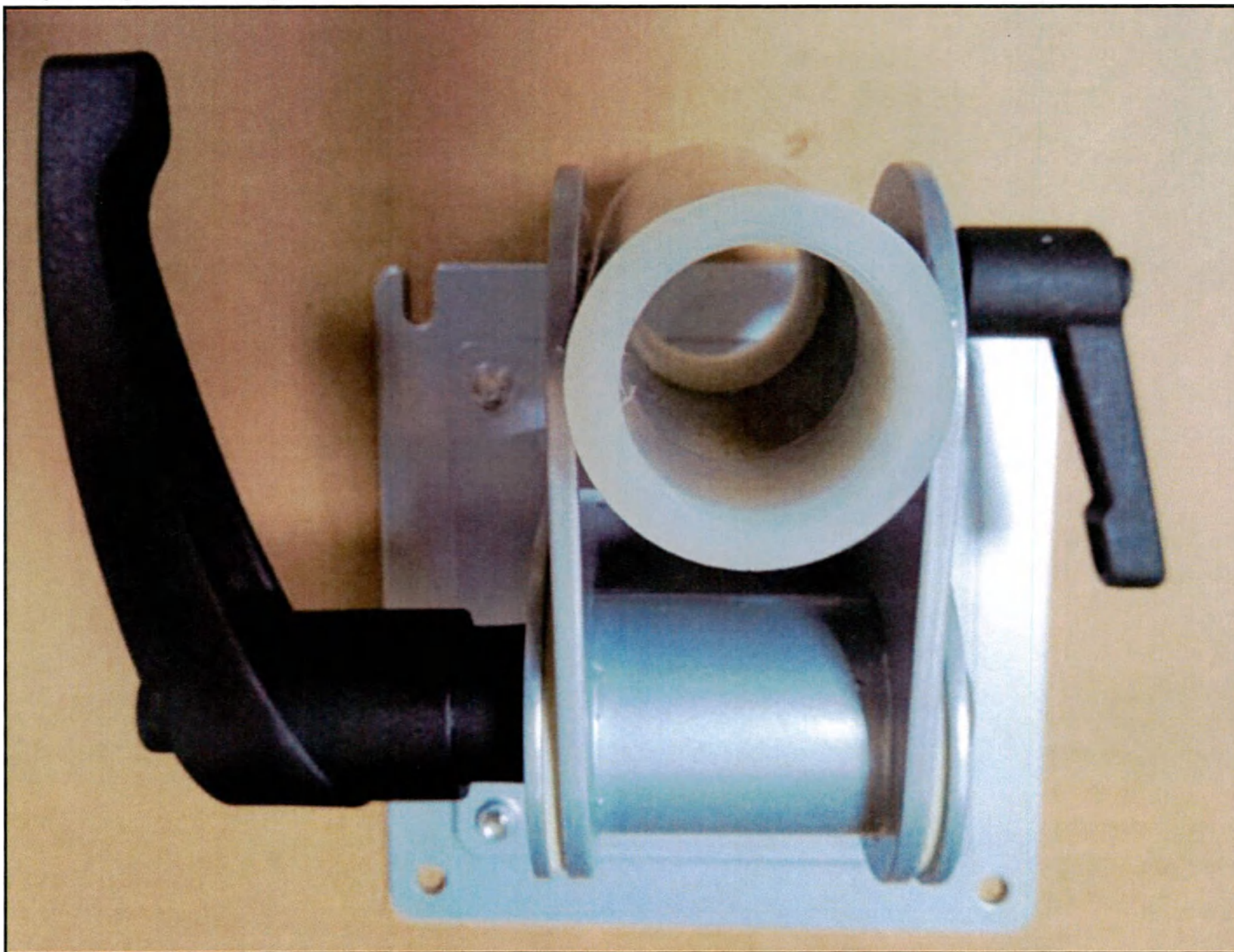
Модуль для крепления монитора, для стойки мобильной COR
