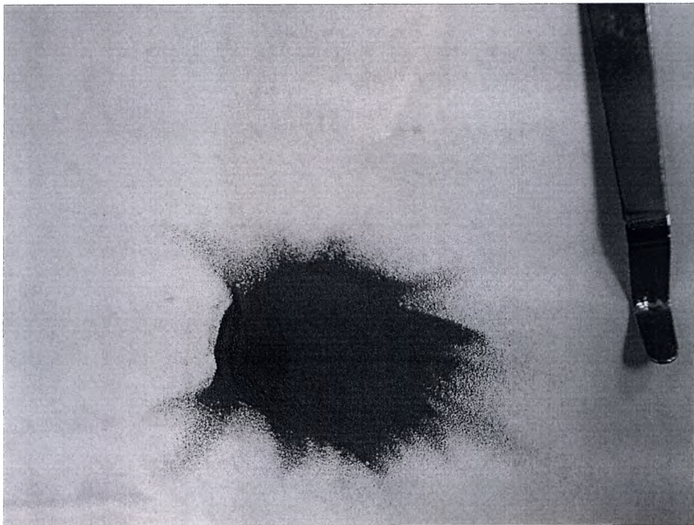
Внешний вид сплава титанового стоматологического в форме порошка для производства стоматологических протезов методом селективного лазерного плавления по ТУ 32.50.11-007-31072128-2018
