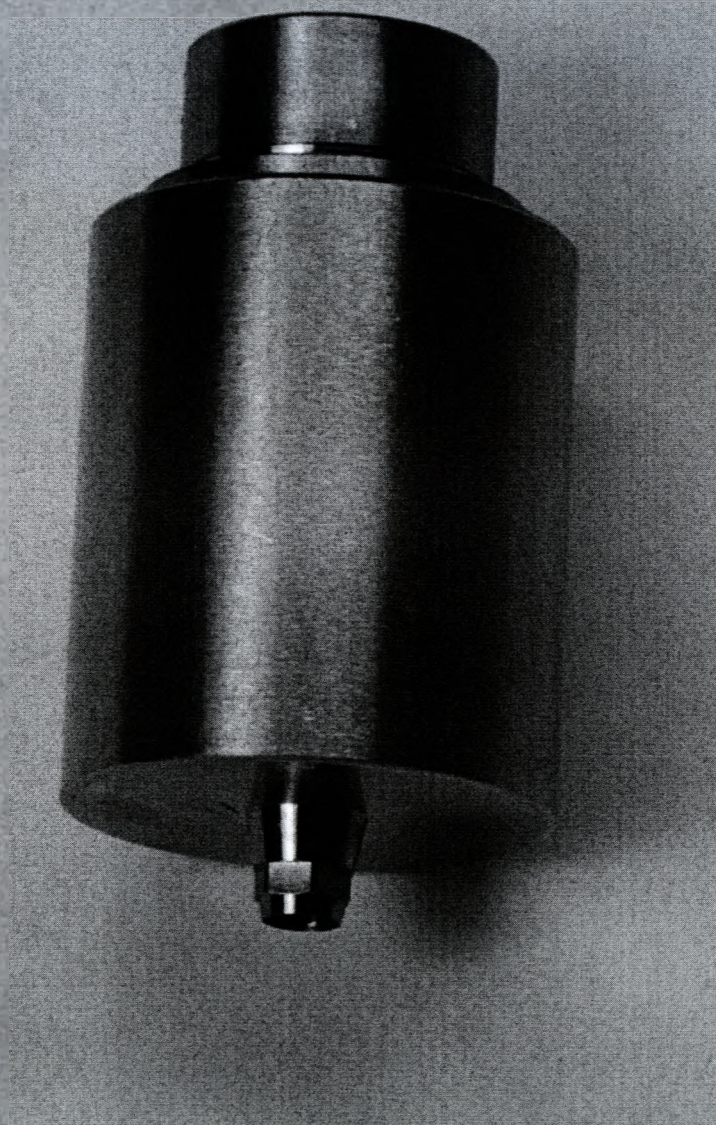
Заготовка для индивидуального абатмента Impro45Z14
