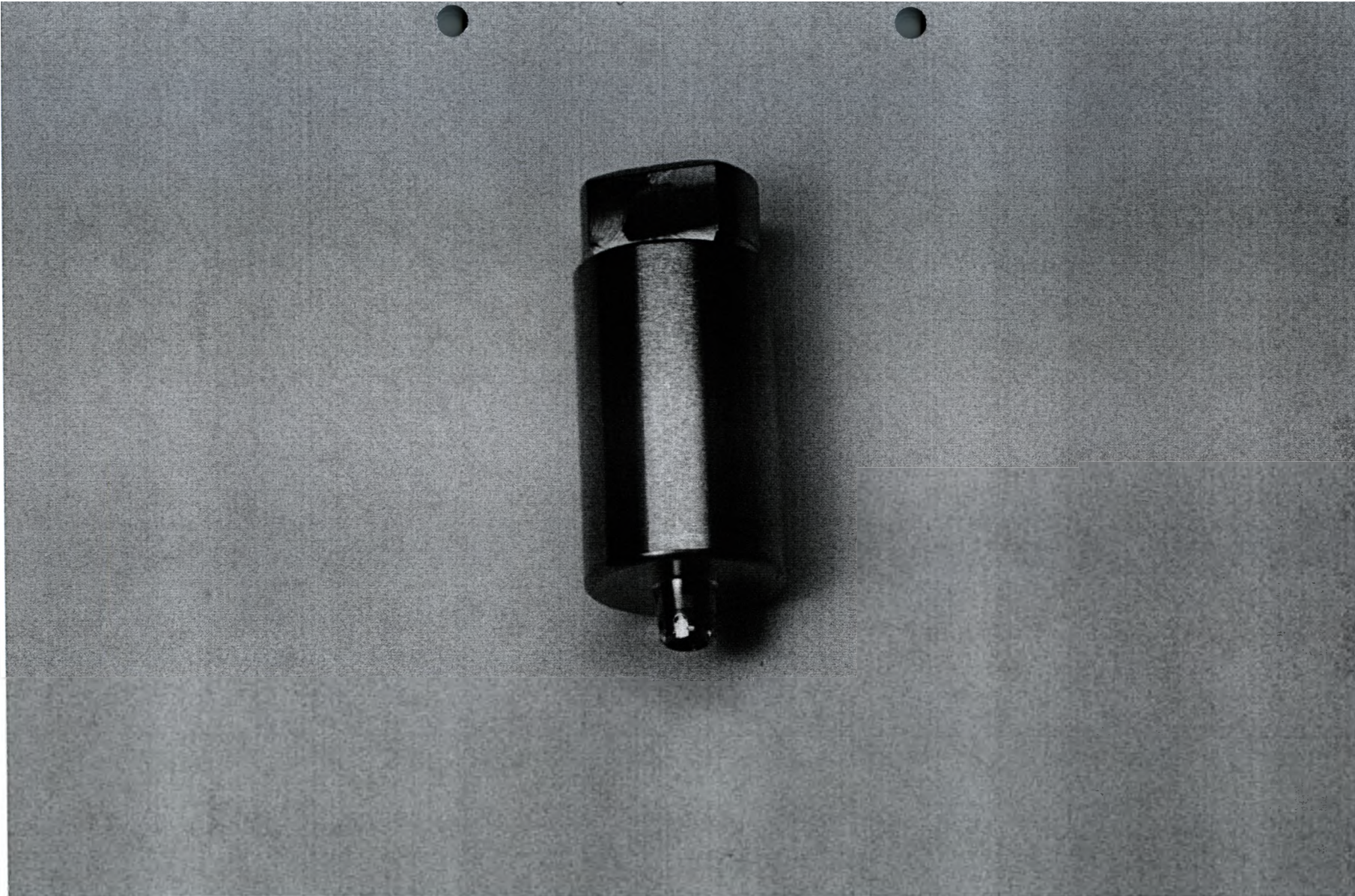
Заготовка для индивидуального абатмента MC1SPZ10
