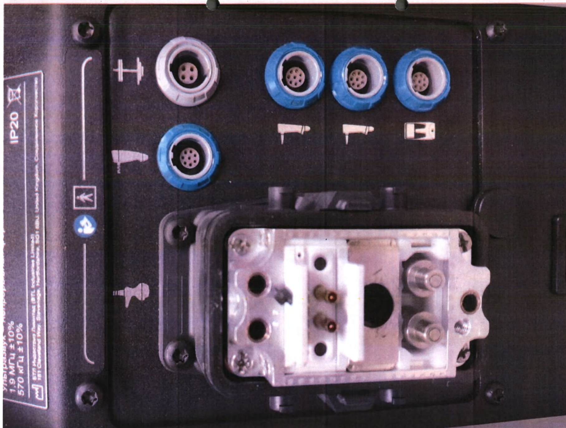
Разъем подключения аппликаторов
