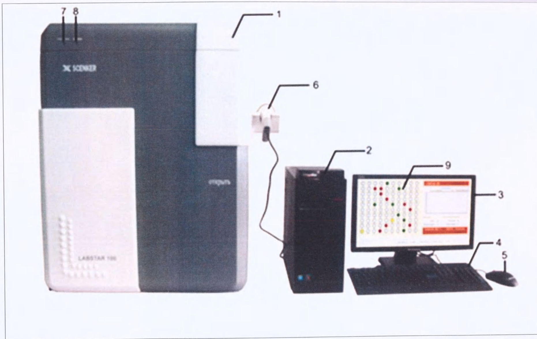
Анализатор бактериологический автоматический ЮНОНА® LABSTAR 100 (общий вид с принадлежностями) 1 – основной модуль, 2 – компьютер, 3 – монитор, 4 – клавиатура, 5 – мышь, 6 – сканер, 7 – индикатор питания, 8 – индикатор температуры, 9 – программное обеспечение
