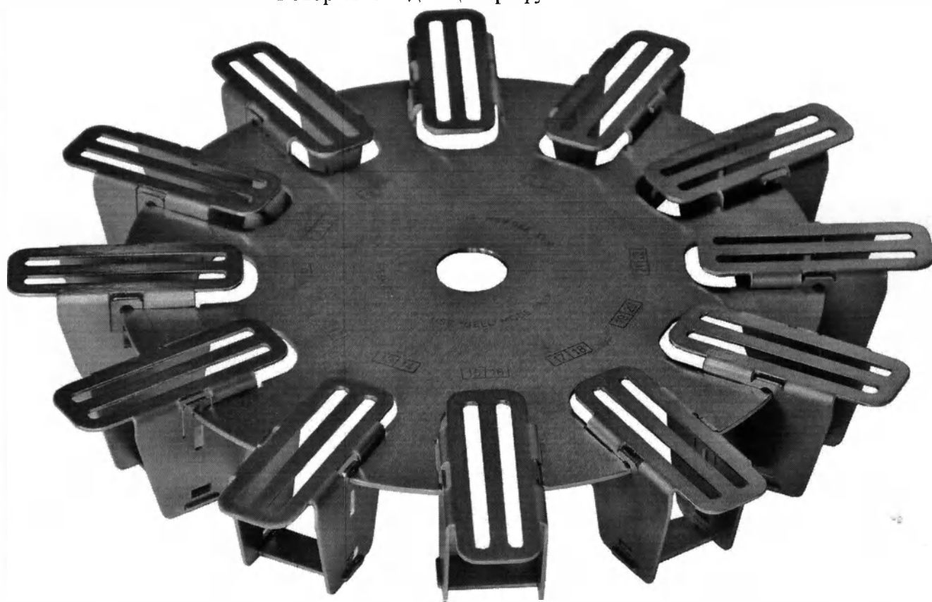
Ротор 6М.03 для центрифуги СМ-6МТ
