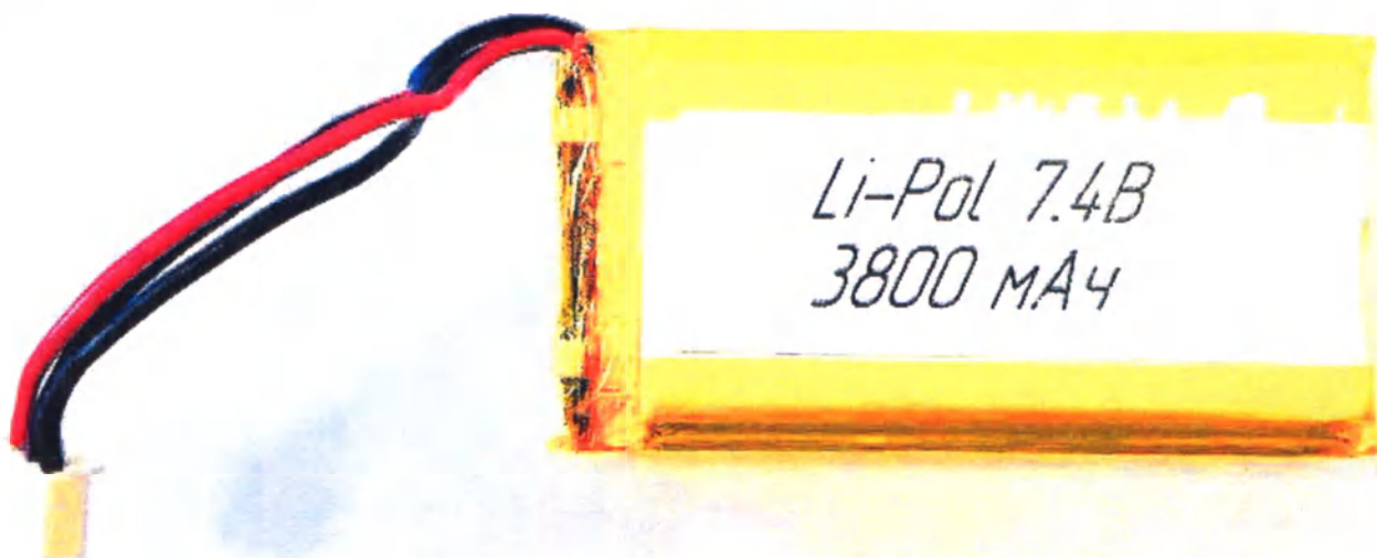
Фотографическое изображение батареи повышенной емкости для инфузионных насосов НК-100II, hawk-i1.
