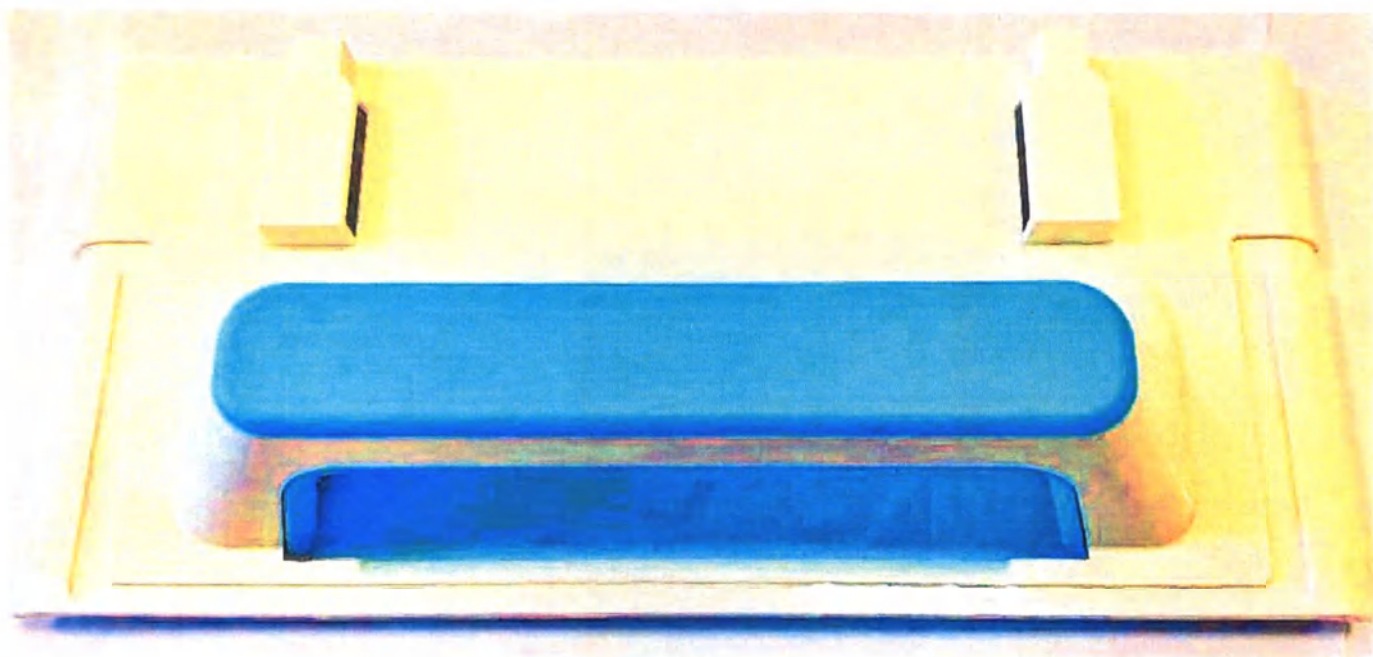
Фотографическое изображение батареи повышенной емкости для инфузионных насосов НК-100II, hawk-i1.
