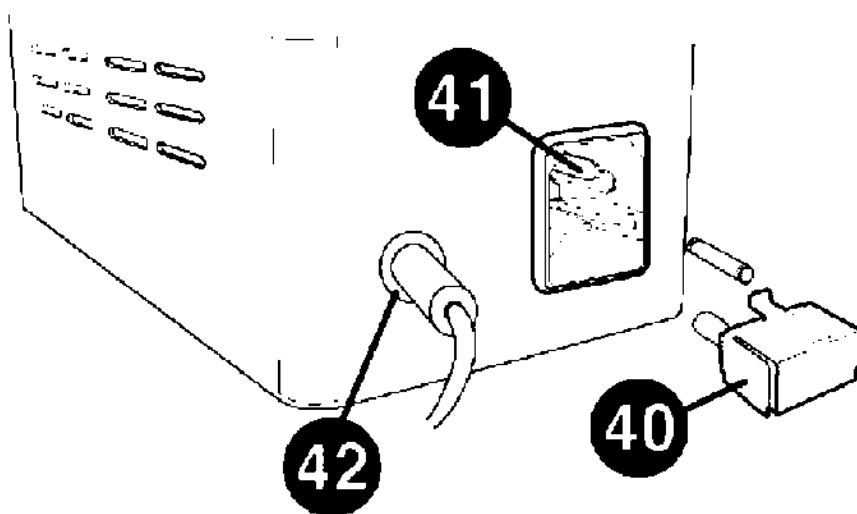
Рис. 9. Замена предохранителей
