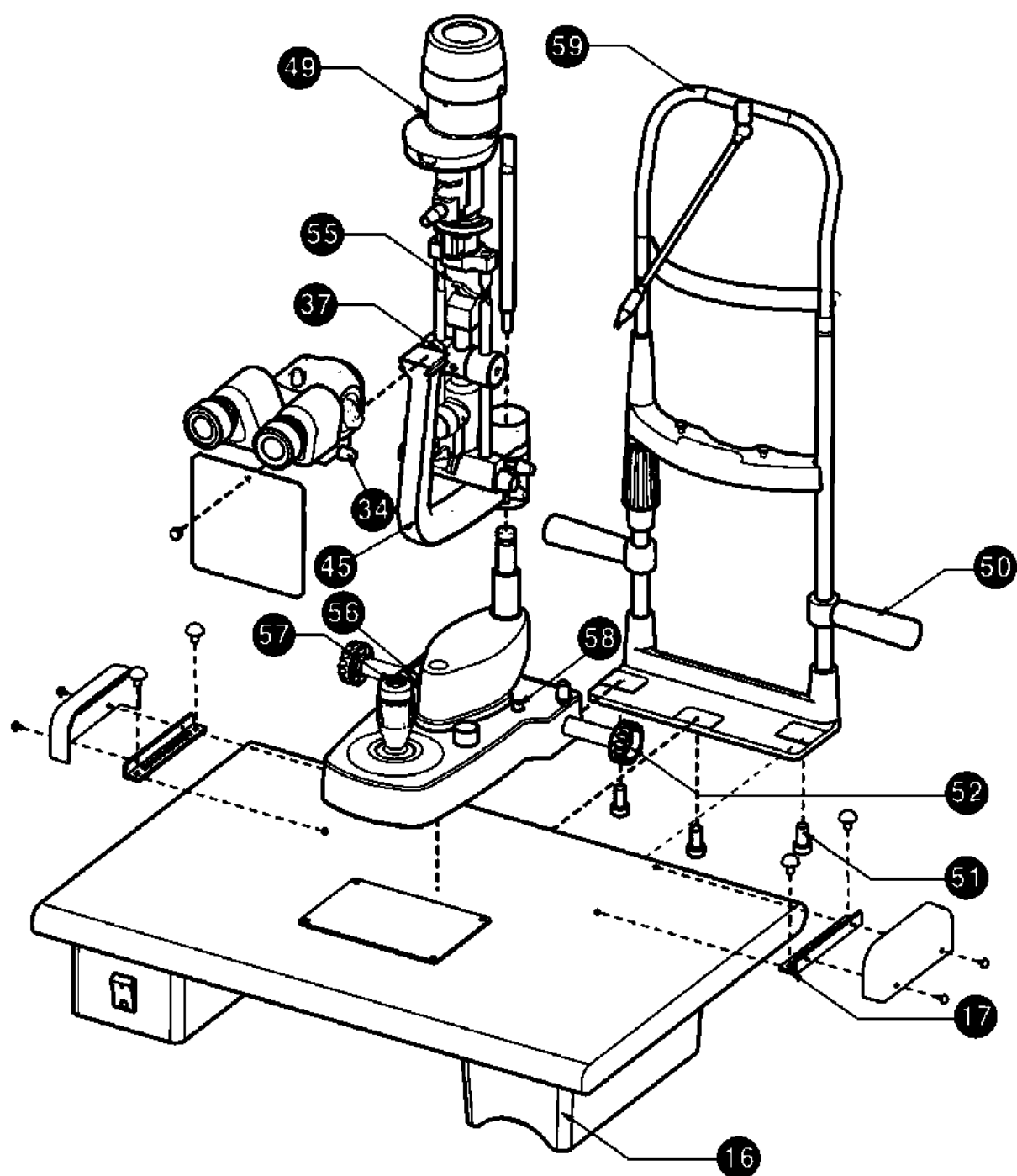
Рис.3 Сборка-II
