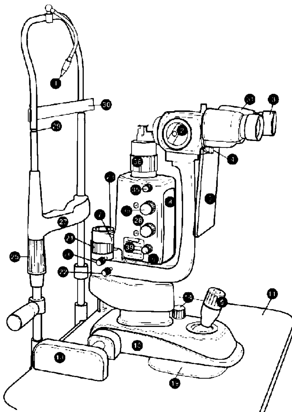
Рис. 2. Сборка-I
