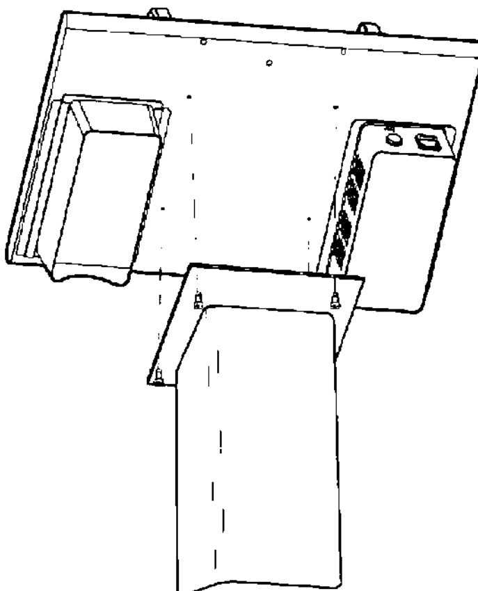
Рис. 4 Сборка стола
