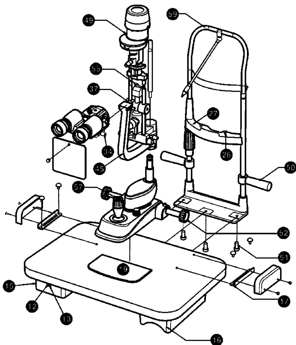
Рис.3 Сборка-II
