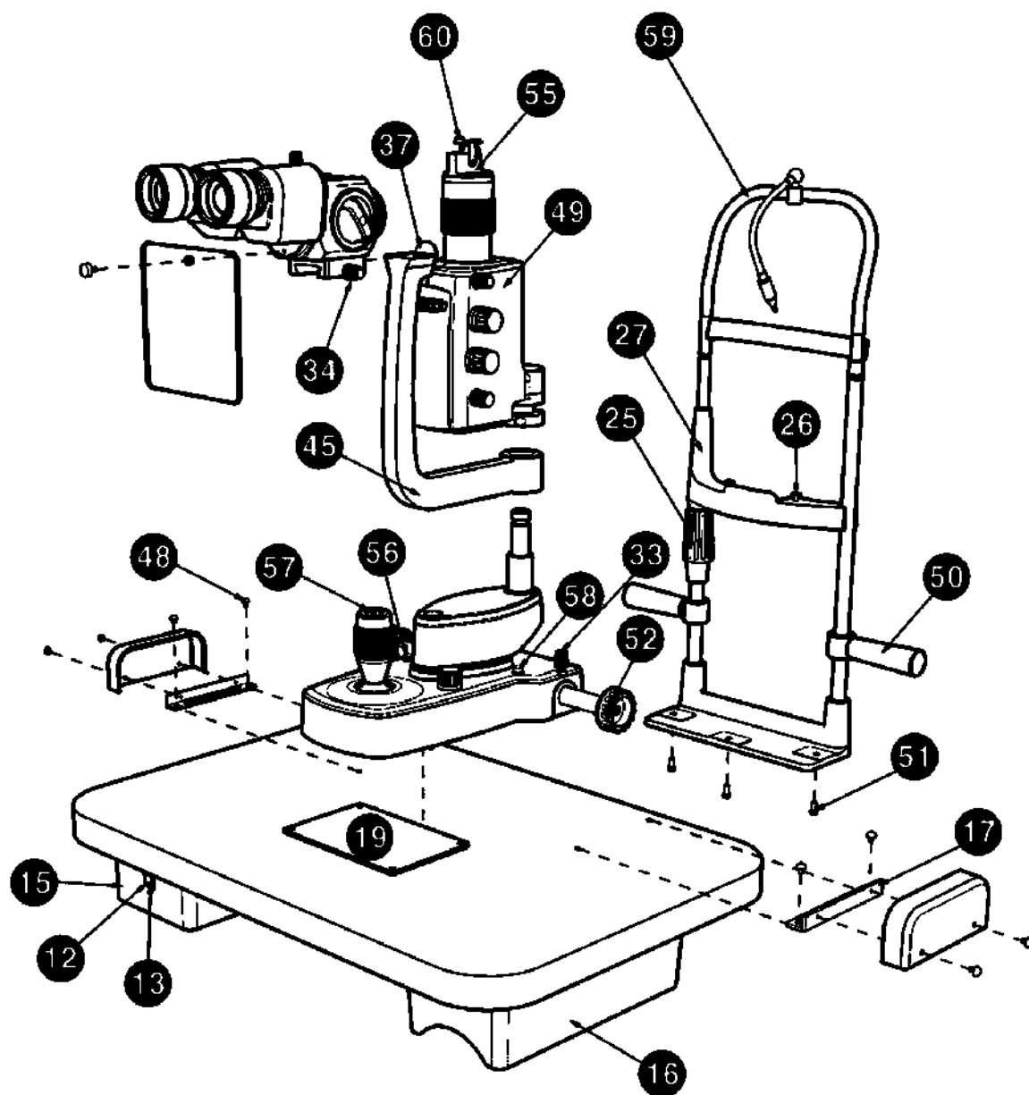
Рис.3 Сборка-II
