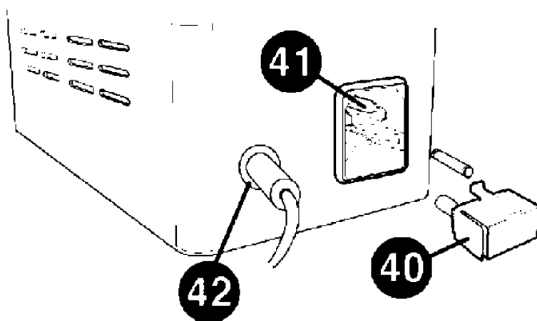
Рис. 8 Замена предохранителей
