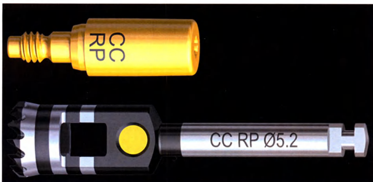
4. Костная мельница с направляющей Bone Mill with Guide Conical Connection RP Ø5,2
