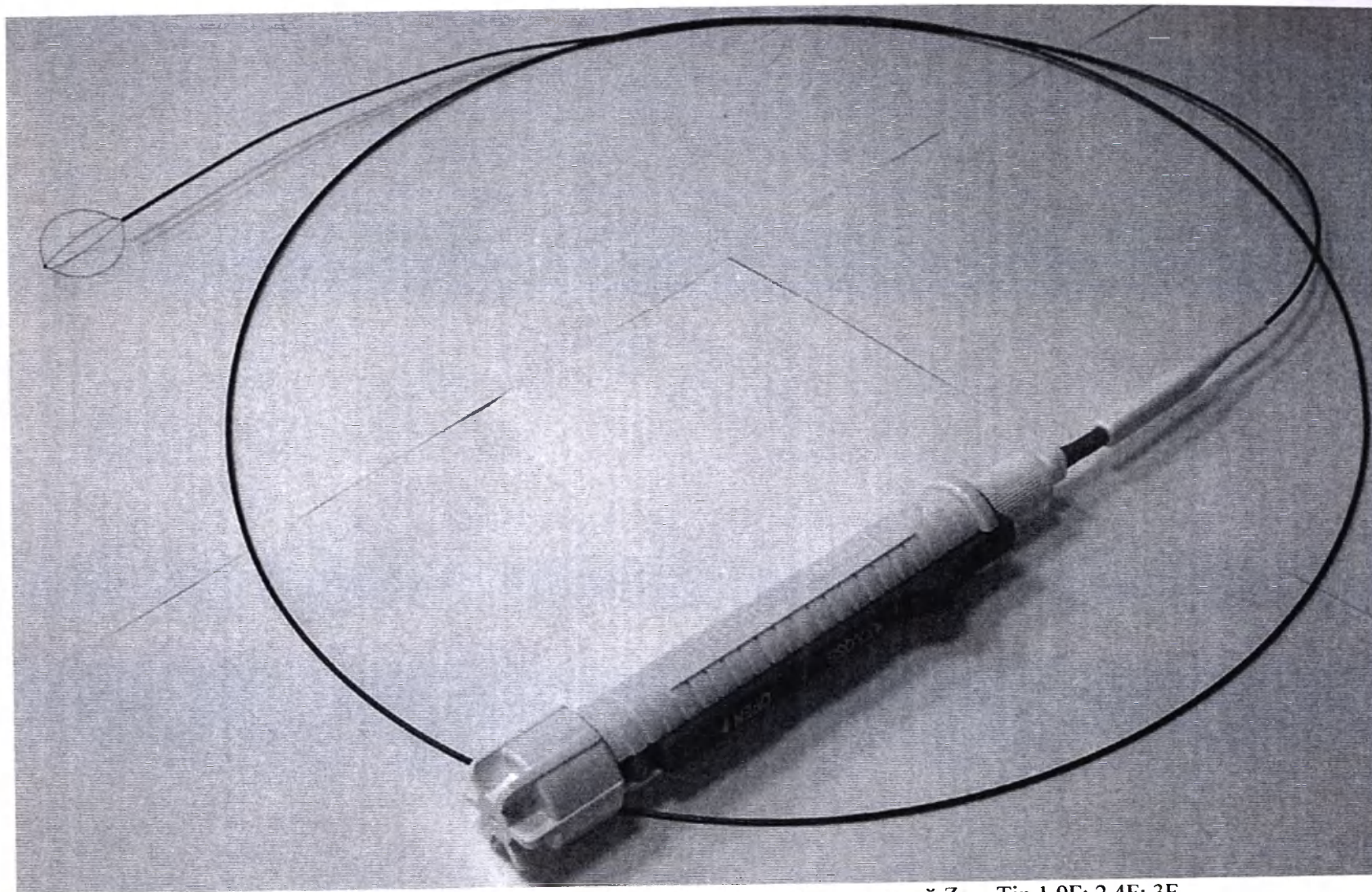
Рис. 10 Захваты типа «корзинка» нитиноловые для удаления камней Zero Tip 1,9F; 2,4F; 3F
