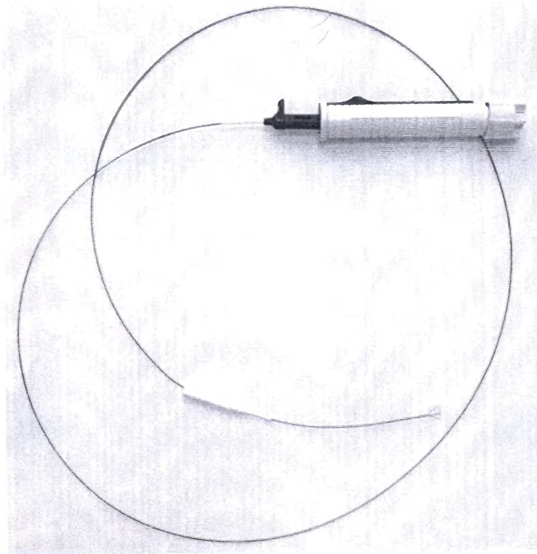
Рис. 20 Захваты типа «корзинка» нитиновые для удаления камней Dakota 1,9F, диаметр раскрытия корзинки 8 мм
