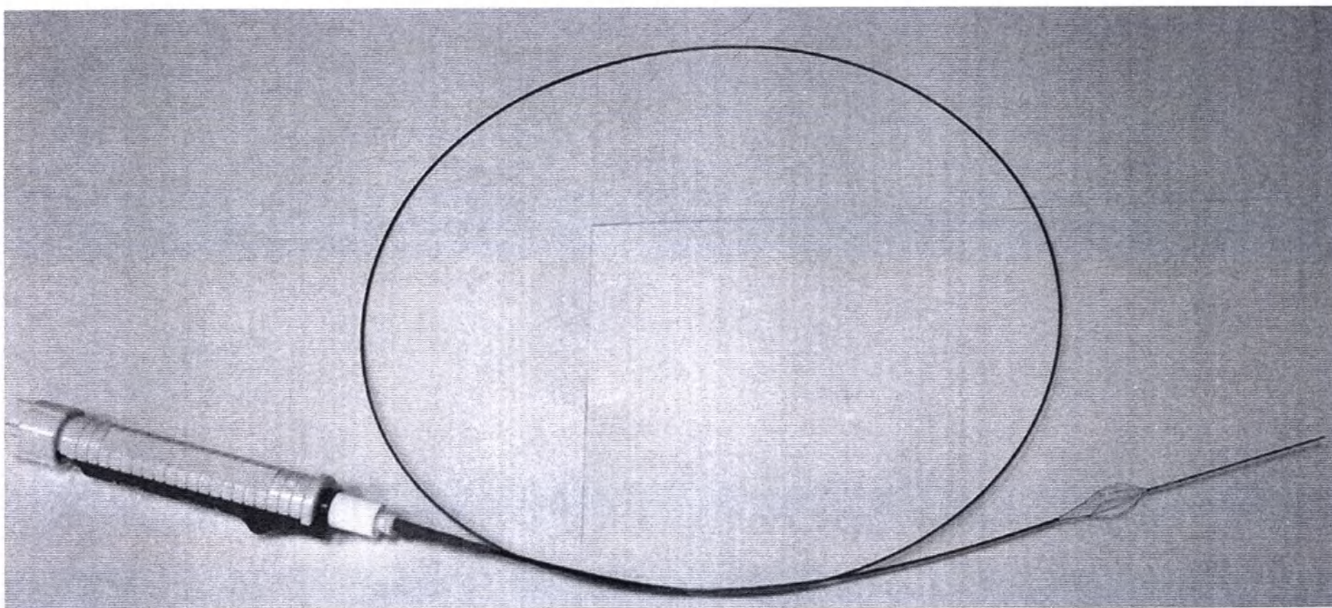
Рис. 7 Захваты типа «корзинка» для удаления камней Leslie Parachute многопроволочные (нитевидный наконечник 5 см) 3,1F
