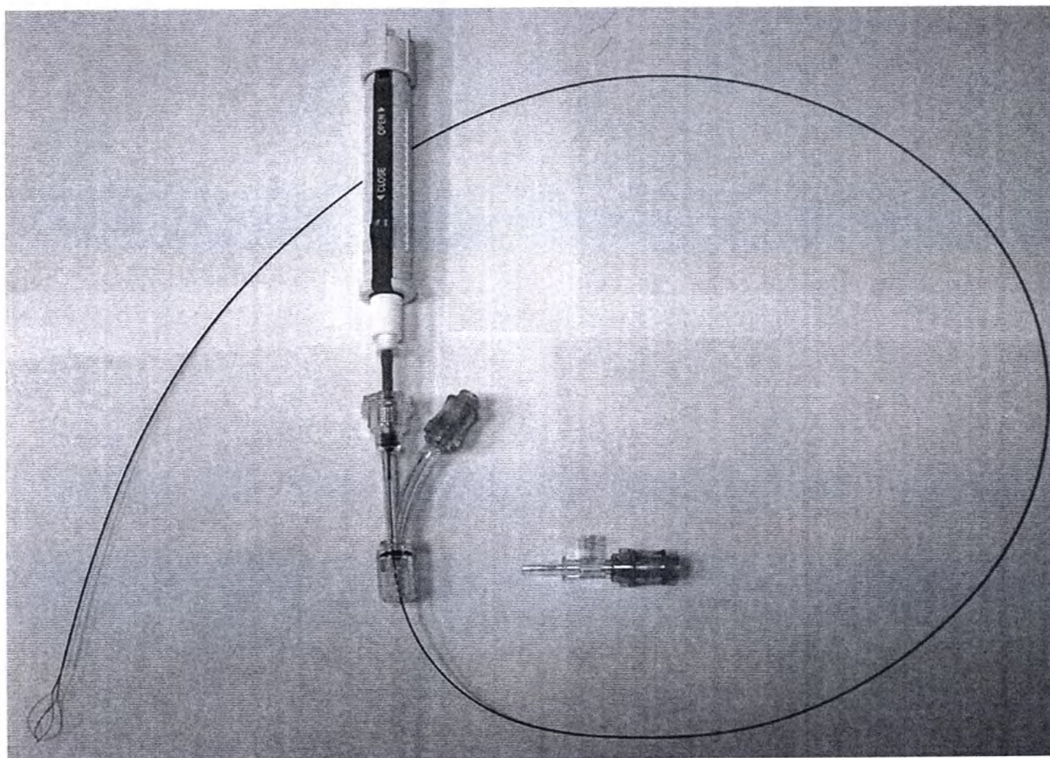
Рис. 8 Захваты типа «корзинка» нитиновые для удаления камней Escape 1,9F
