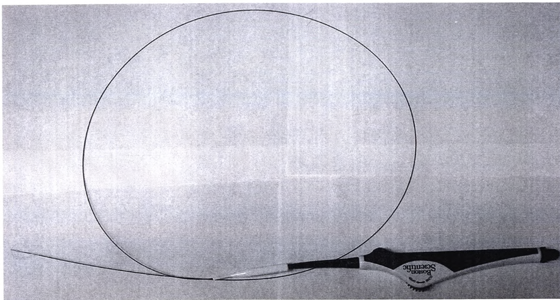
Рис. 9 Захваты типа «корзинка» нитиновые для удаления камней OptiFlex 1,3F
