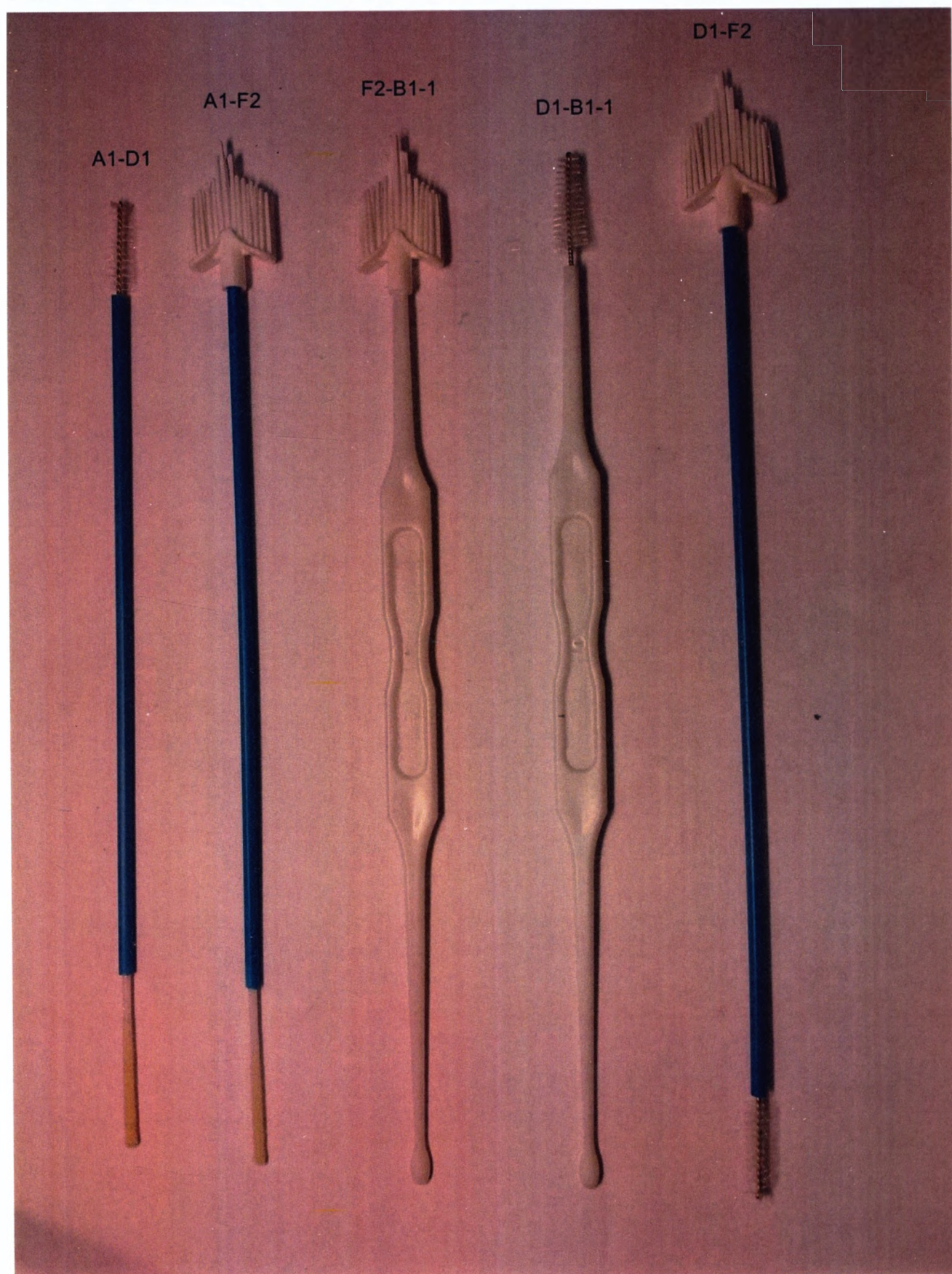
Фото 10. Зонд двухсторонний типов А-Д, А-Ф, F-B, D-B, D-F (на примере изображения зондов типов А1-Д1, А1-Ф2, F2-B1-1, D1-B1-1, D1-Ф2).
