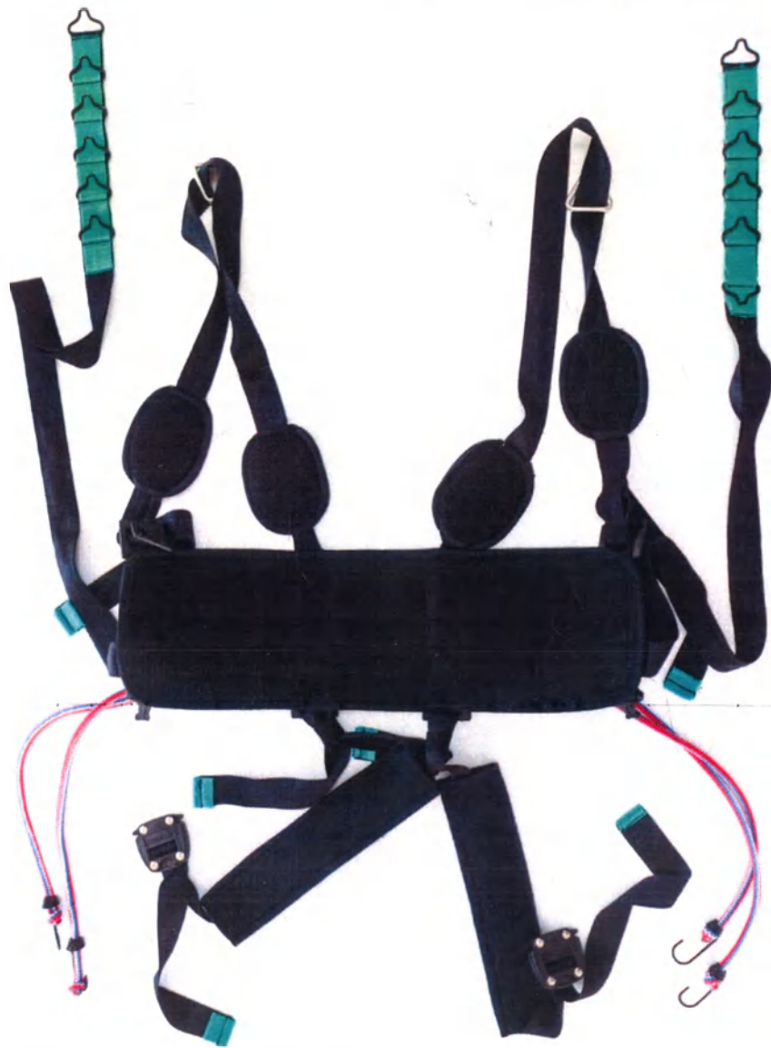
ФОТО 22. ПРИНАДЛЕЖНОСТИ. Удерживающее приспособление «Стандарт» мод.01.00
