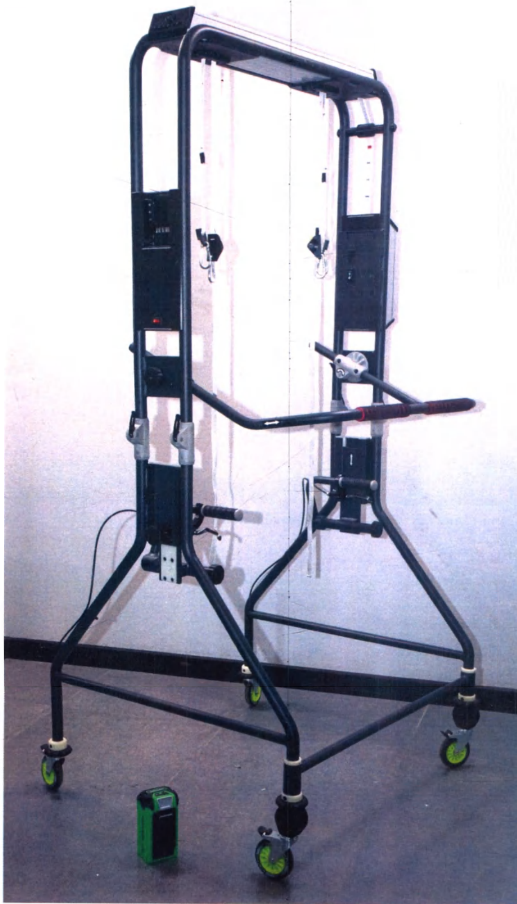
ФОТО 2. МОБИЛЬНАЯ РАМА ДЛЯ РАЗГРУЗКИ ВЕСА ПРИ ХОДЬБЕ (МОБИЛЬНАЯ СЛИНГ-СИСТЕМА – ВЕРТИКАЛИЗАТОР) МССЭ. Мобильная рама (в сборе) со съёмным аккумулятором
