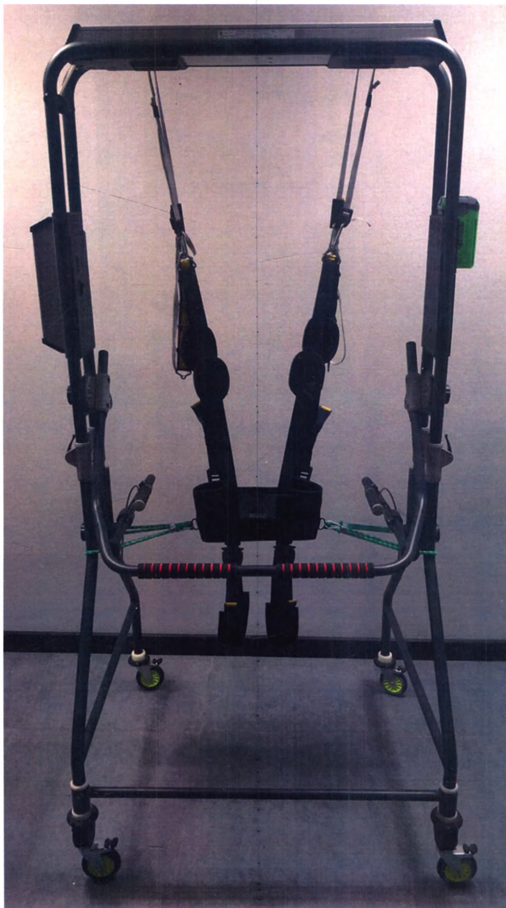
ФОТО 1. МОБИЛЬНАЯ РАМА ДЛЯ РАЗГРУЗКИ ВЕСА ПРИ ХОДЬБЕ (МОБИЛЬНАЯ СЛИНГ-СИСТЕМА – ВЕРТИКАЛИЗАТОР) МССЭ
