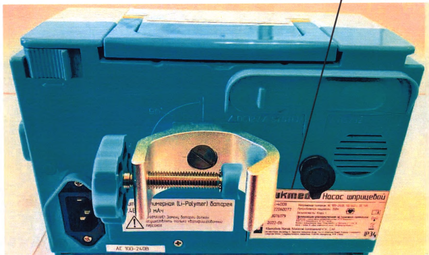
Фотографическое изображение насоса шприцевого НК-400III: основной блок с батареей и зажимом для крепления к стойке (вид сзади).
