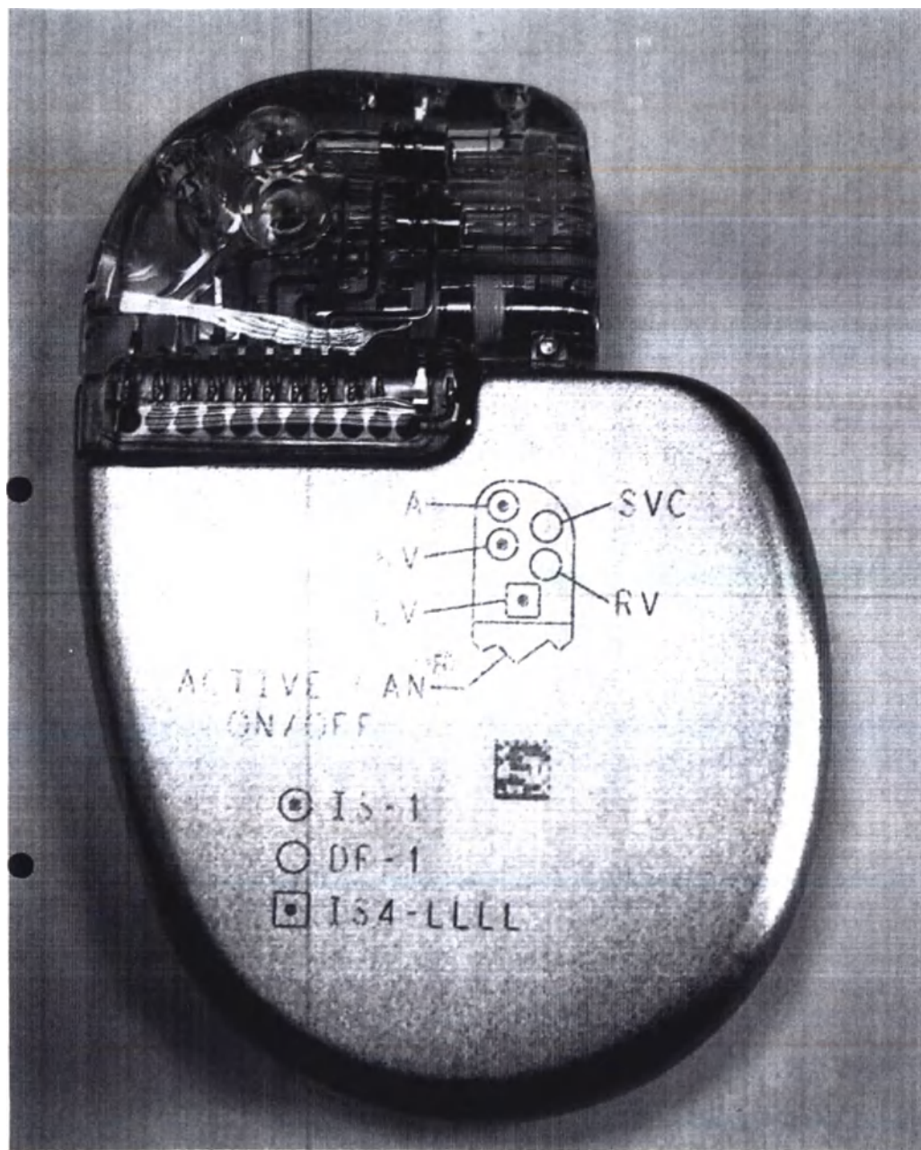
Задняя часть Цифрового имплантируемого кардиовертера-дефибриллятора с функцией сердечной ресинхронизирующей терапии и технологией SureScan AMPLIA MRI Quad CRT-D SureScan, модель DTMB2Q1
