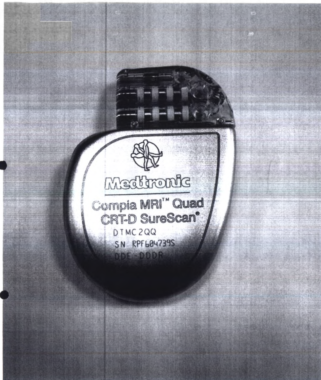
Фронтальная часть Цифрового имплантируемого кардиовертера-дефибриллятора с функцией сердечной ресинхронизирующей терапии и технологией SureScan COMPIA MRI Quad CRT-D SureScan , модель DTMC2QQ
