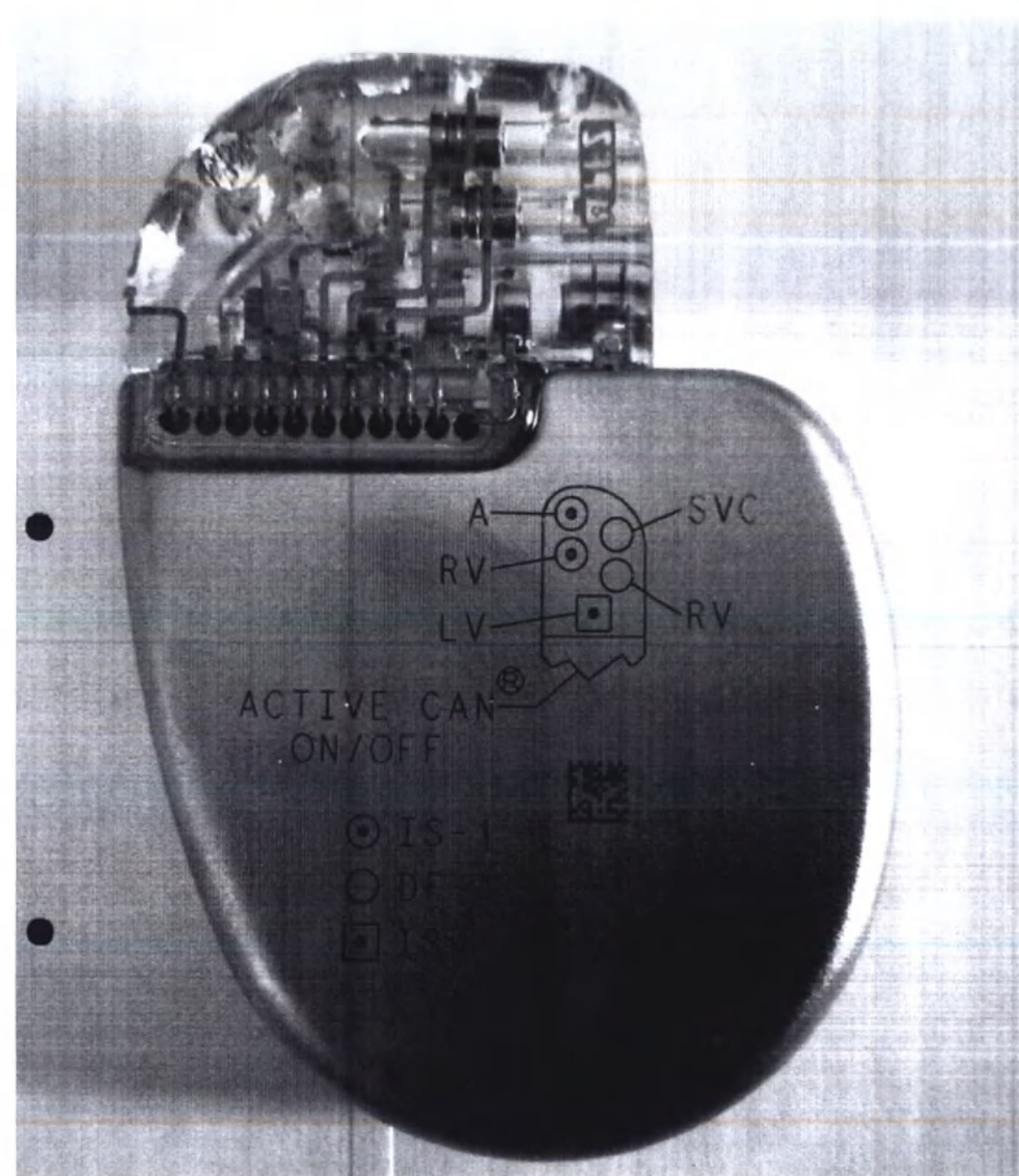
Задняя часть Цифрового имплантируемого кардиовертера-дефибриллятора с функцией сердечной ресинхронизирующей терапии и технологией SureScan CLARIA MRI Quad CRT-D SureScan, модель DTMA2Q1
