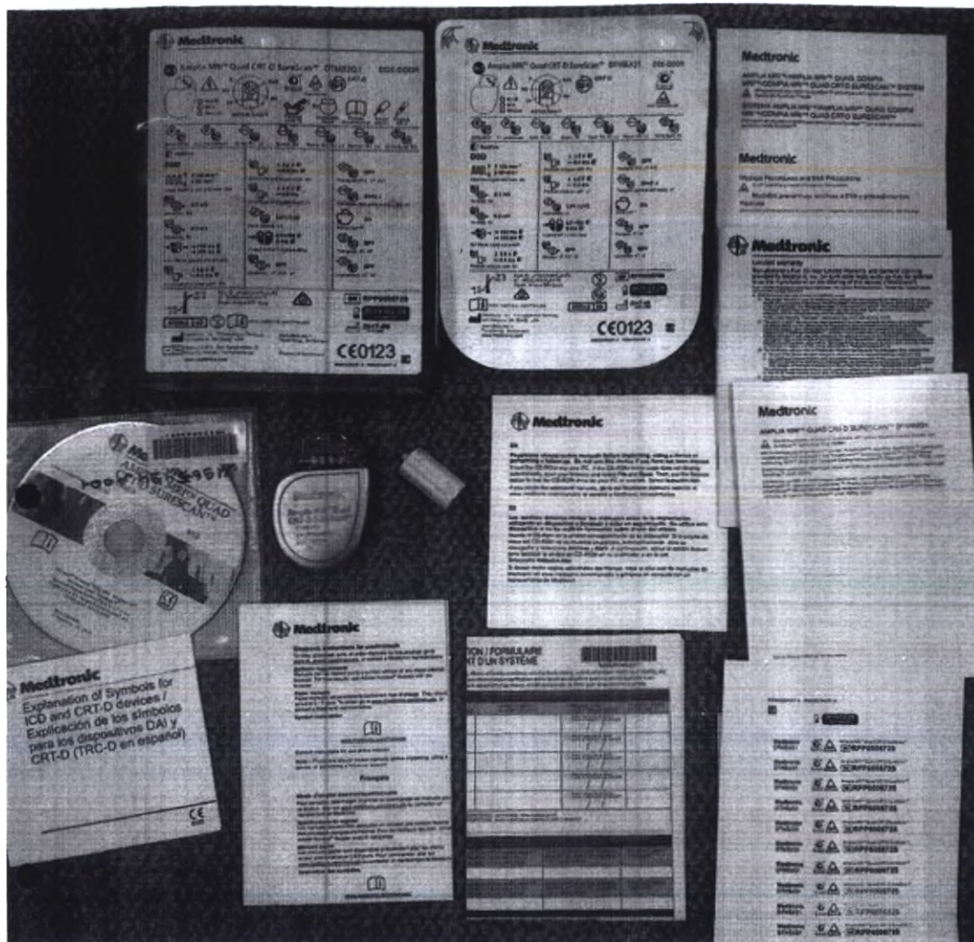
Цифровой имплантируемый кардиовертер-дефибриллятор с функцией сердечной ресинхронизирующей терапии и технологией SureScan AMPLIA MRI Quad CRT-D SureScan, модель DTMB2Q1 – комплект поставки
