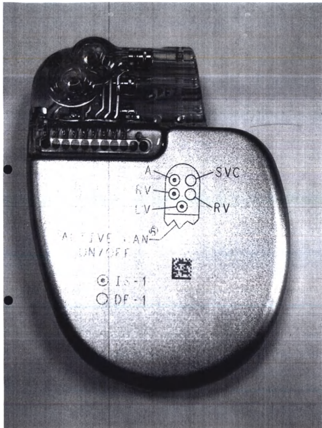
Задняя часть Цифрового имплантируемого кардиовертера-дефибриллятора с функцией сердечной ресинхронизирующей терапии и технологией SureScan COMPIA MRI CRT-D SureScan, модель DTMC2D1
