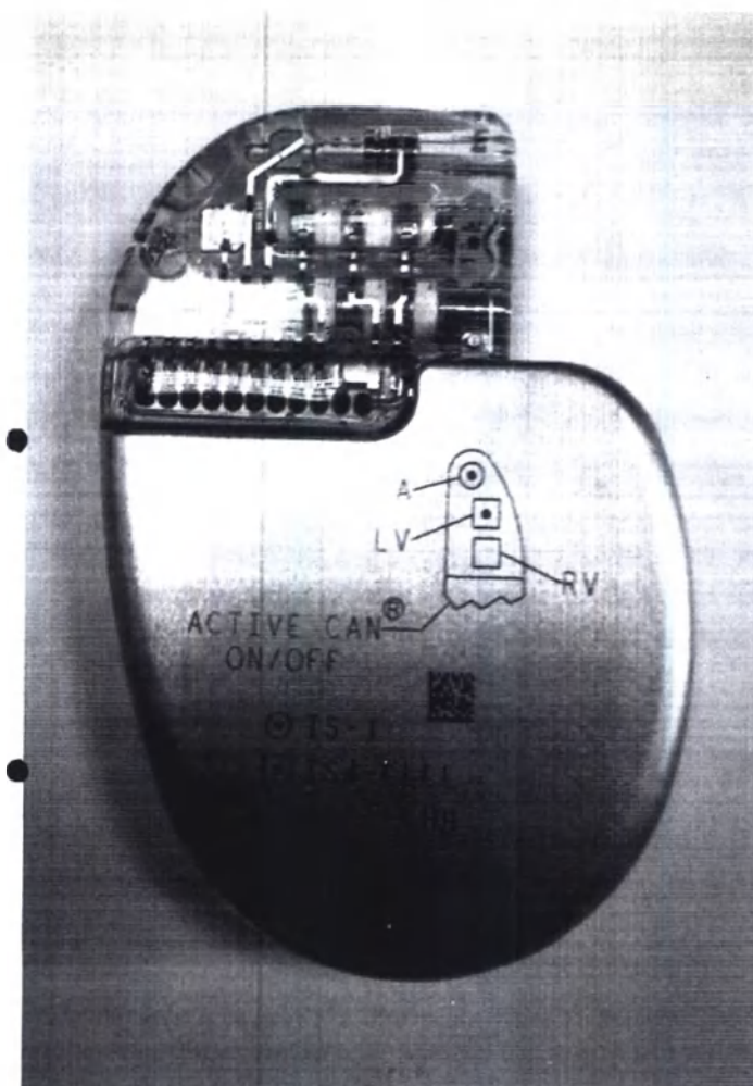
Задняя часть Цифрового имплантируемого кардиовертера-дефибриллятора с функцией сердечной ресинхронизирующей терапии и технологией SureScan AMPLIA MRI Quad CRT-D SureScan, модель DTMB2QQ
