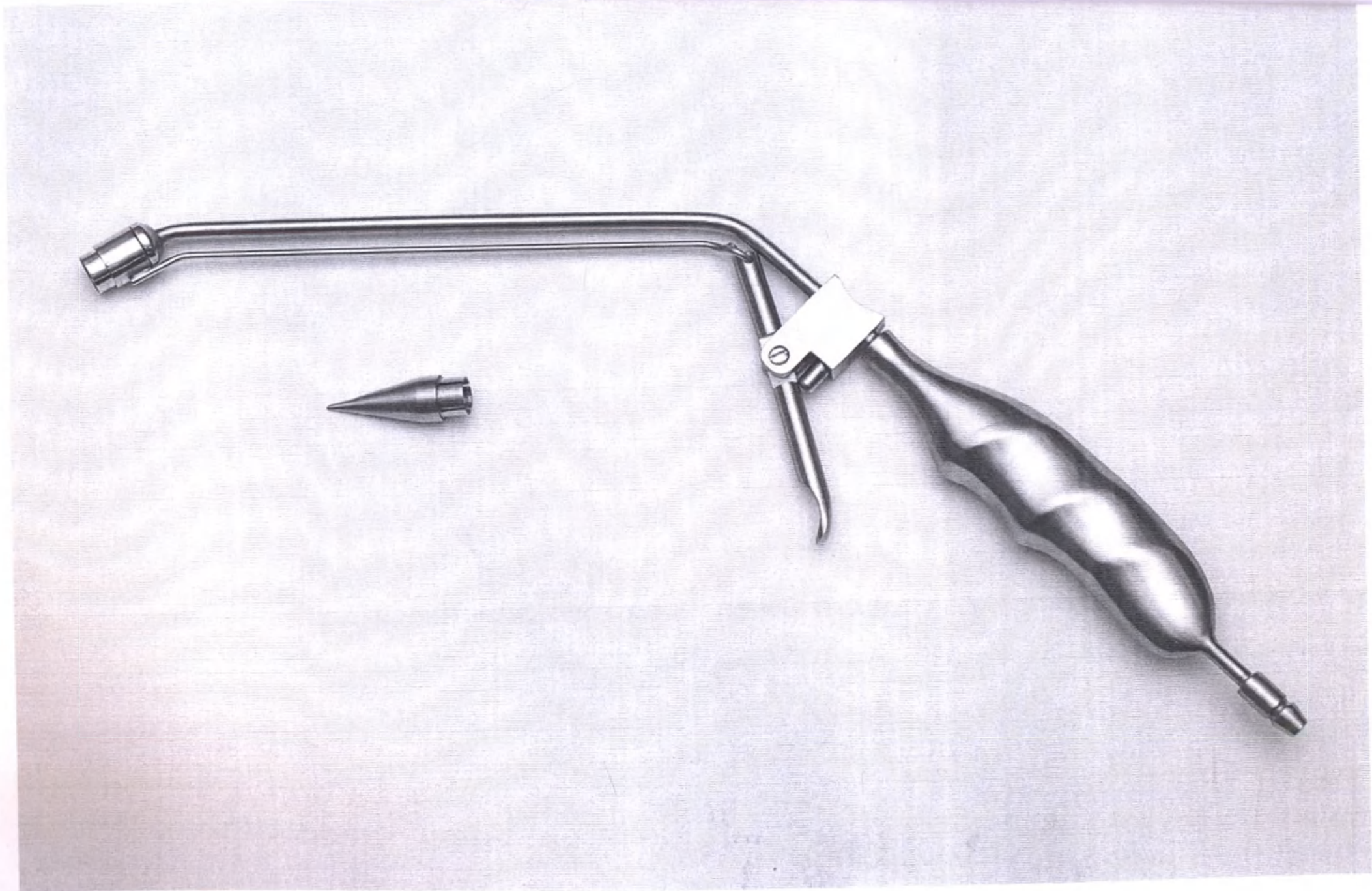
Рис. 18 – Аппликатор для наложения колец
