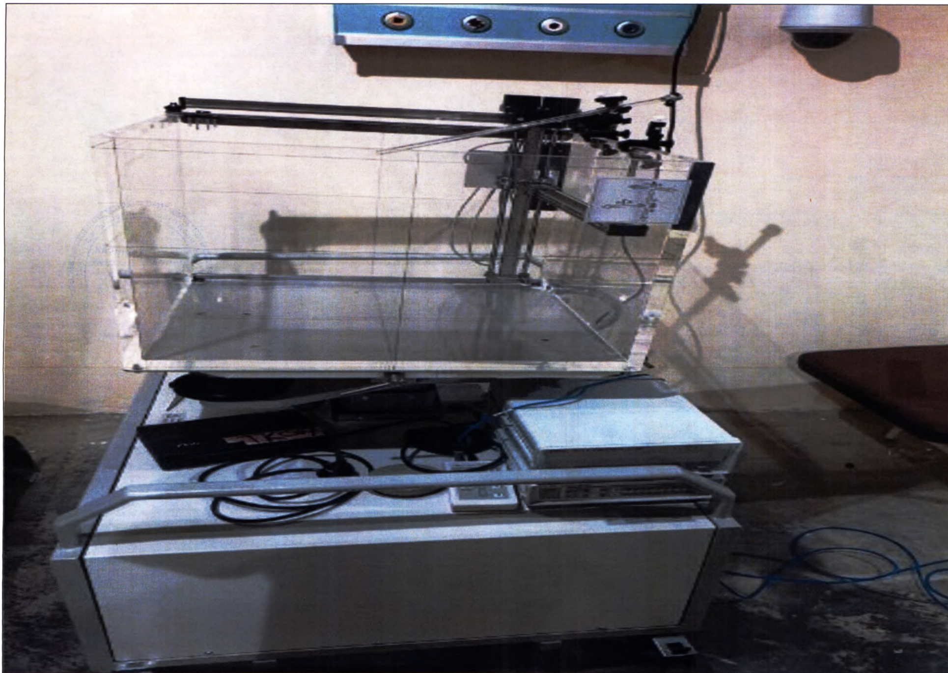
2. Набор стандартный для дозиметрии, в составе: - стандартные фантомы, не более 10 шт.; - водный фантом.
