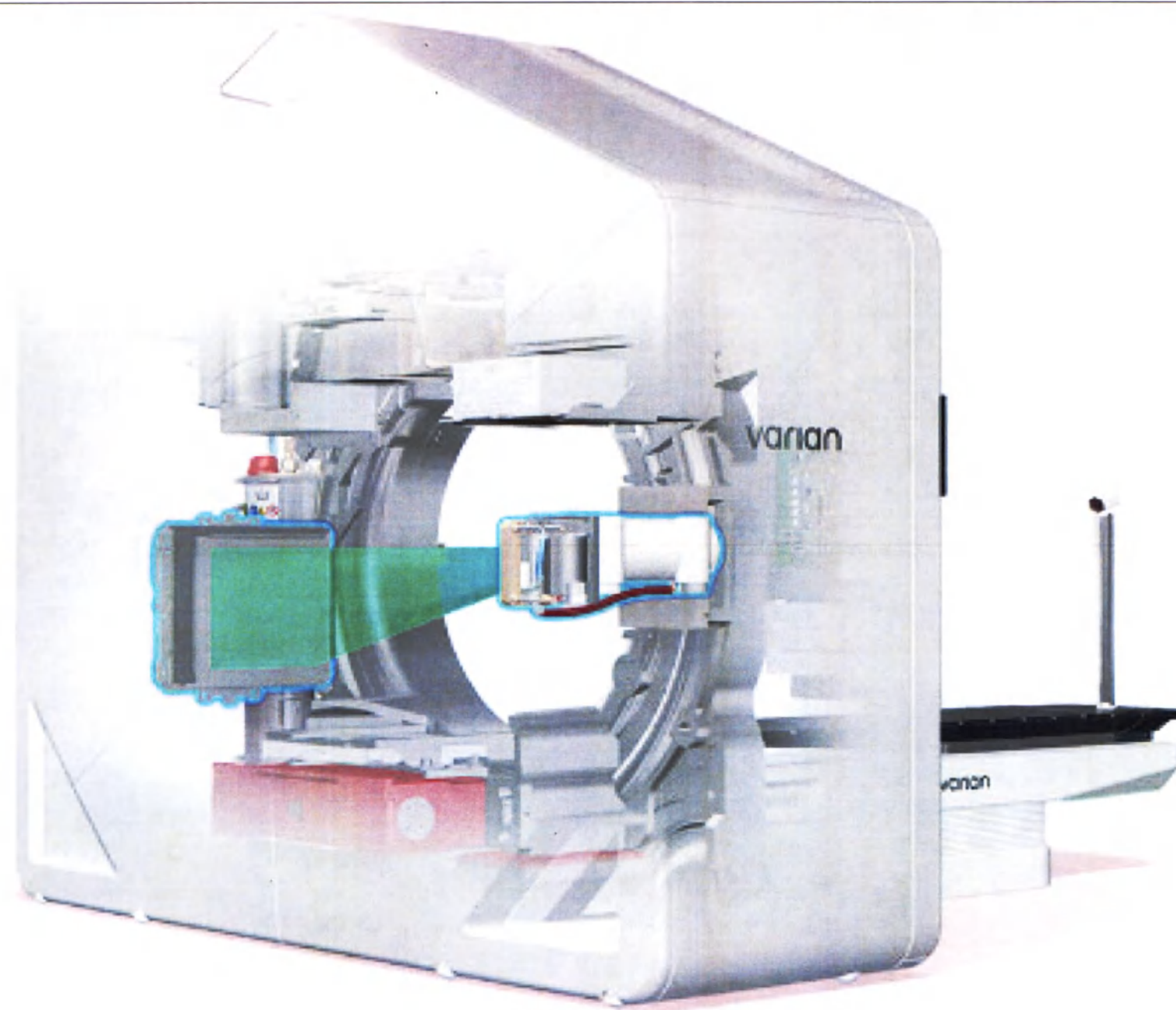
1.4. Система киловольтажной визуализации с функцией получения изображений СТ в коническом пучке (СВСТ)
