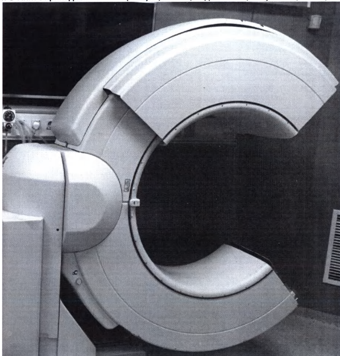
Гентри О-ARM с принадлежностями (кожухи, колеса, подшипники, излучатели, блоки, желобы).
