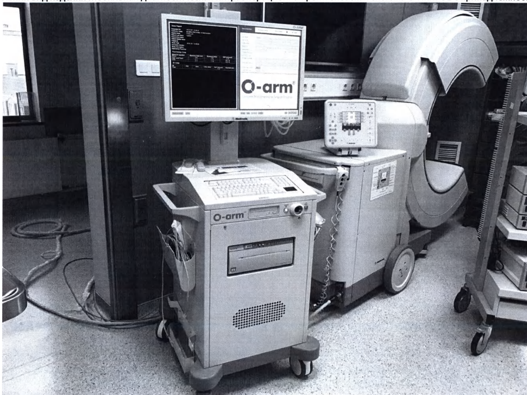
Внешний вид изделия Мобильная диагностическая интраоперационная рентгеновская система O-ARM O2 с принадлежностями
