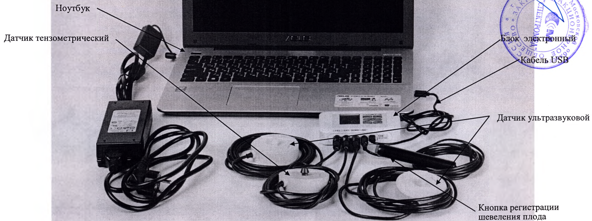
Общий вид - Монитор фетальный «СОНОМЕД 200» исполнение «-В»
