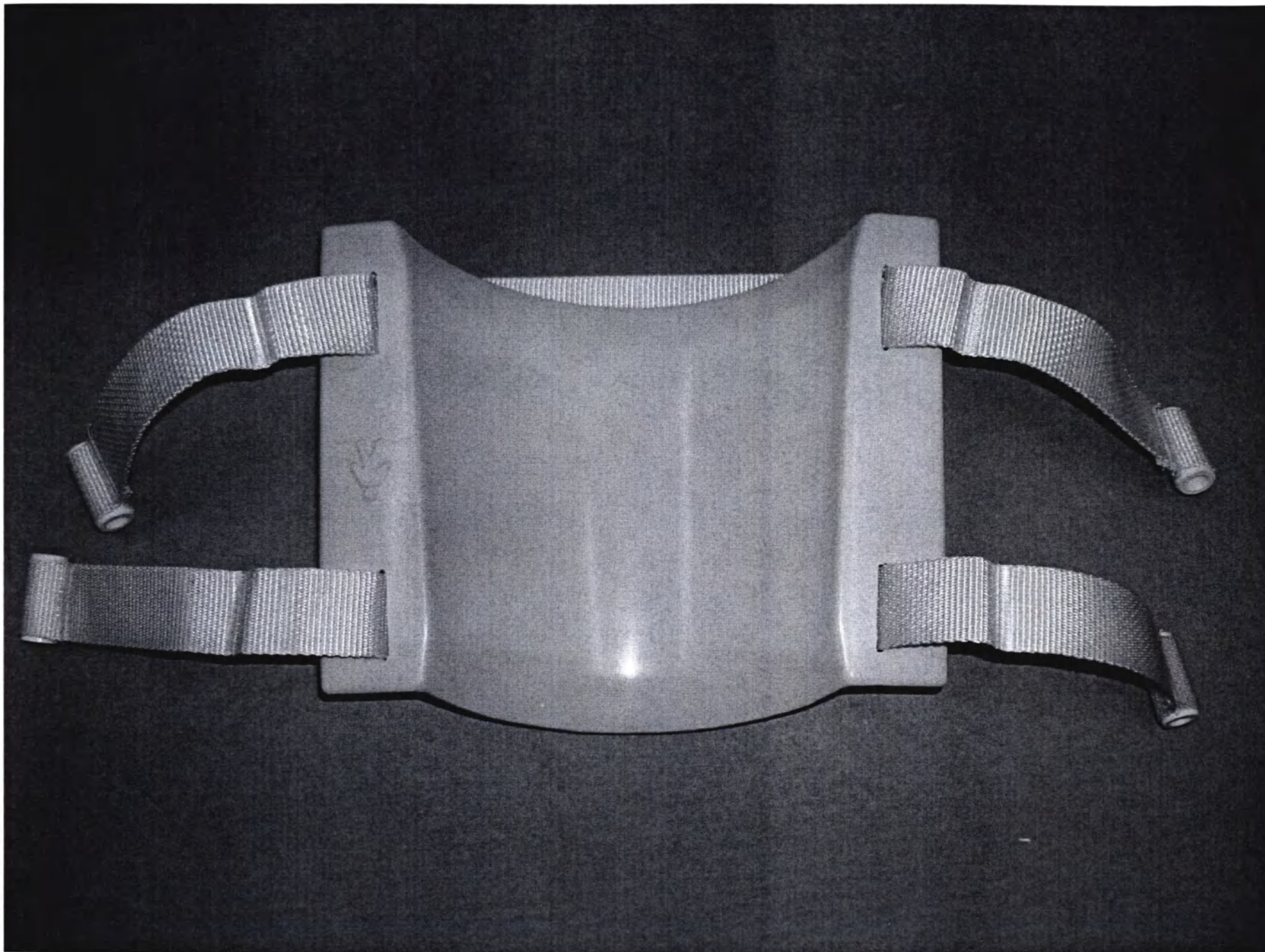
Подкладка под голень
