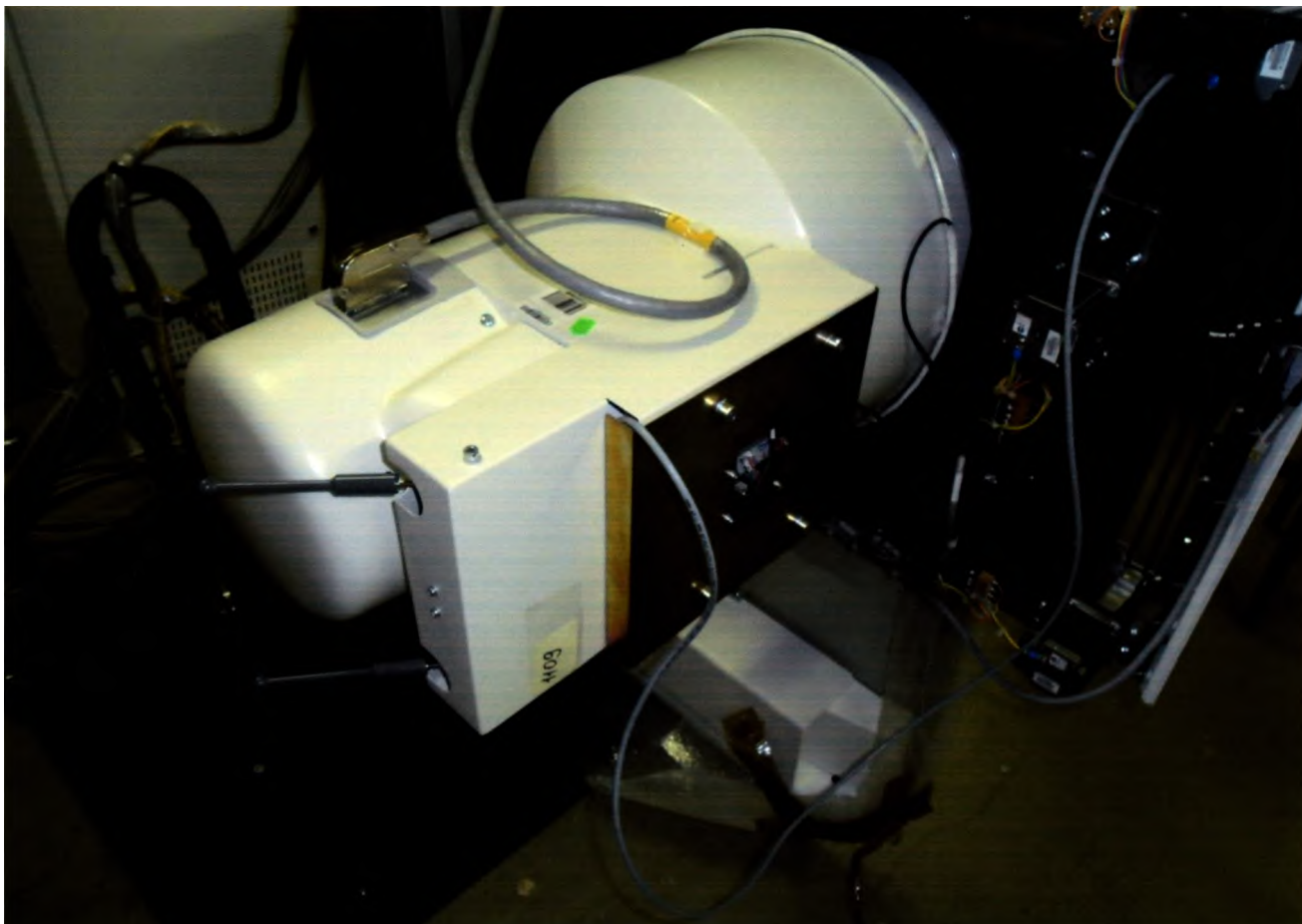
Усилитель рентгеновского изображения УРИ (установлен в систему)
