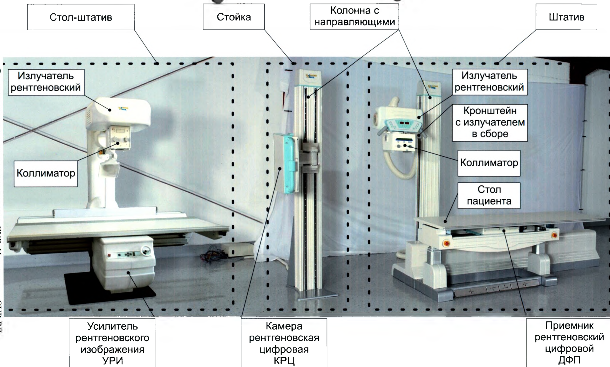
Система универсальная рентгеновская СУР-РД
