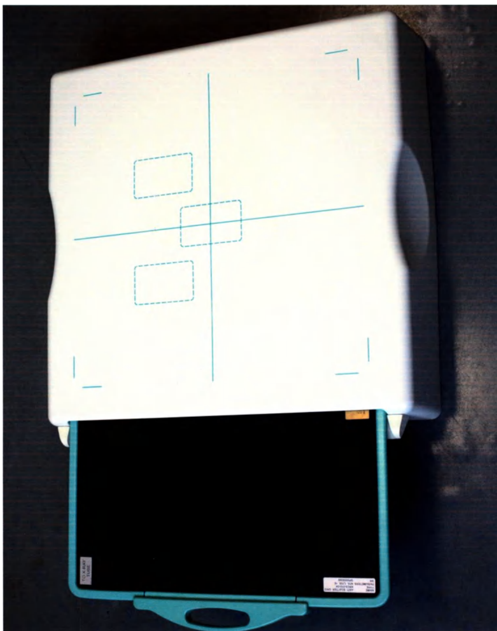
Приемник рентгеновский цифровой ДФП и решетка фокусирующая (растр рентгеновский)
