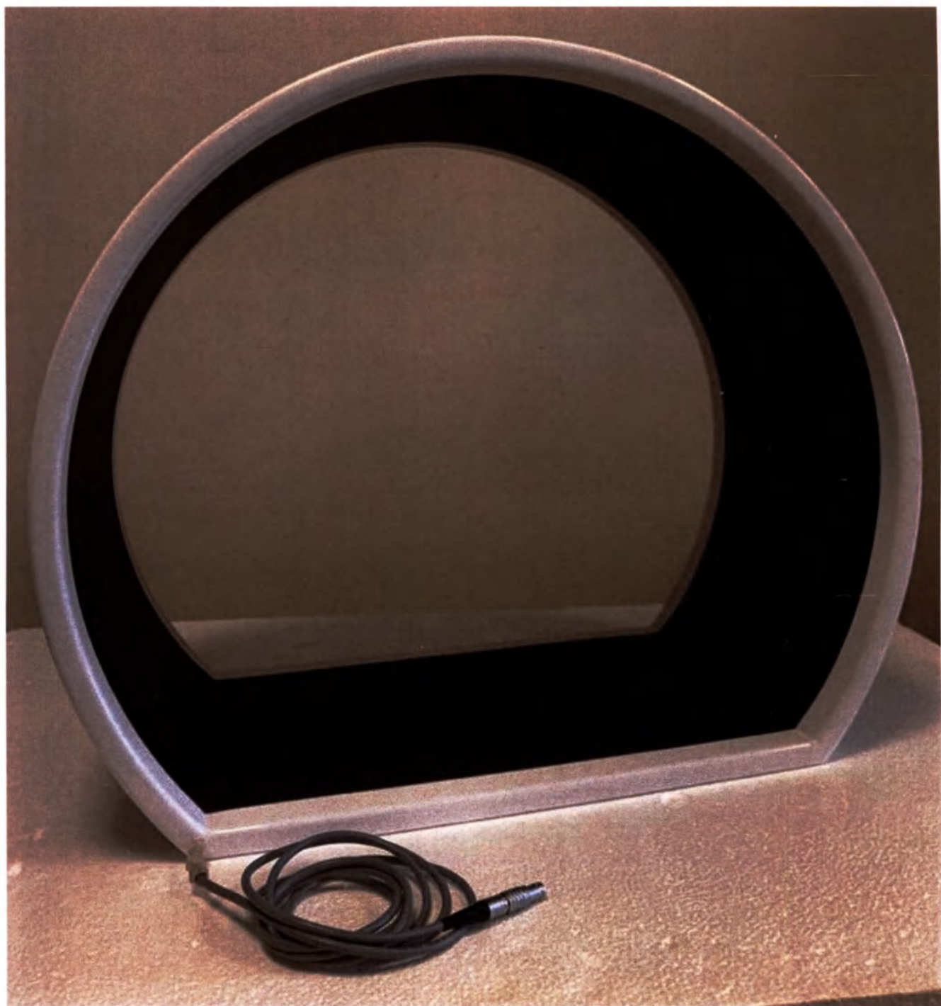
Индуктор №6 (соленоид большой)
