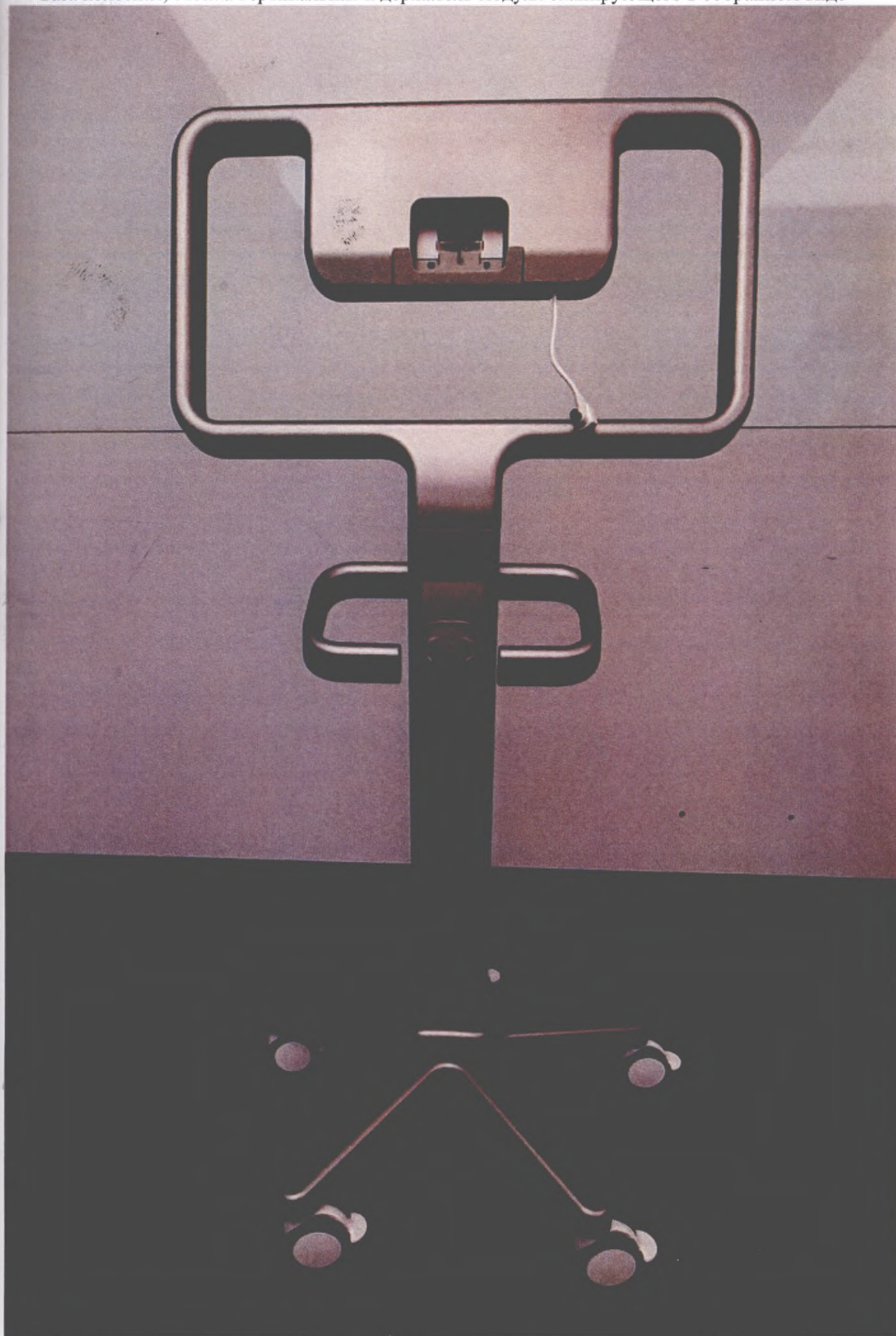
База колёсная, стойка вертикальная и держатель модуля сканирующего в собранном виде
