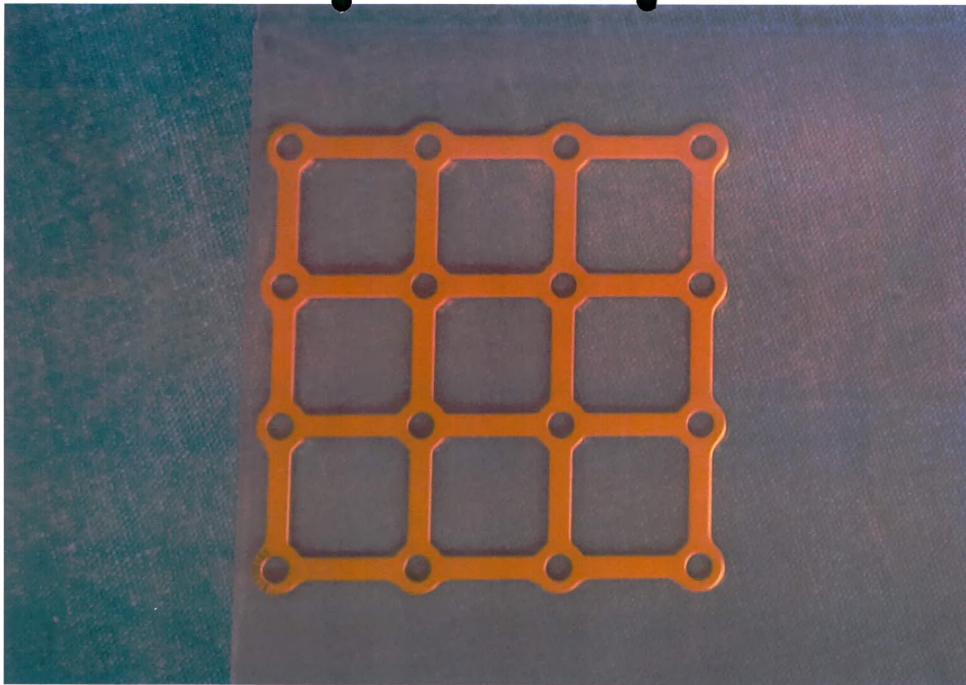
Мини-пластина прямоугольная, симметричная, 16 отверстий (4x4), 1,0 мм x 2,0 мм
