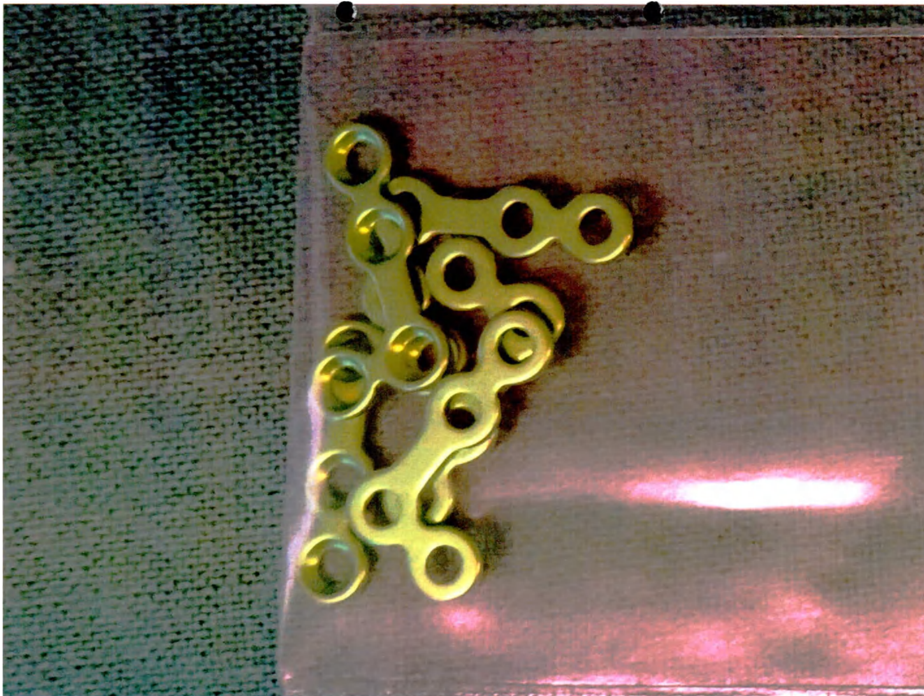
Медиум-пластина L-образная левая, 4 отверстия, планка 6 мм, 0,6 мм x 1,6 мм. Изображена упаковка с 5 изделиями
