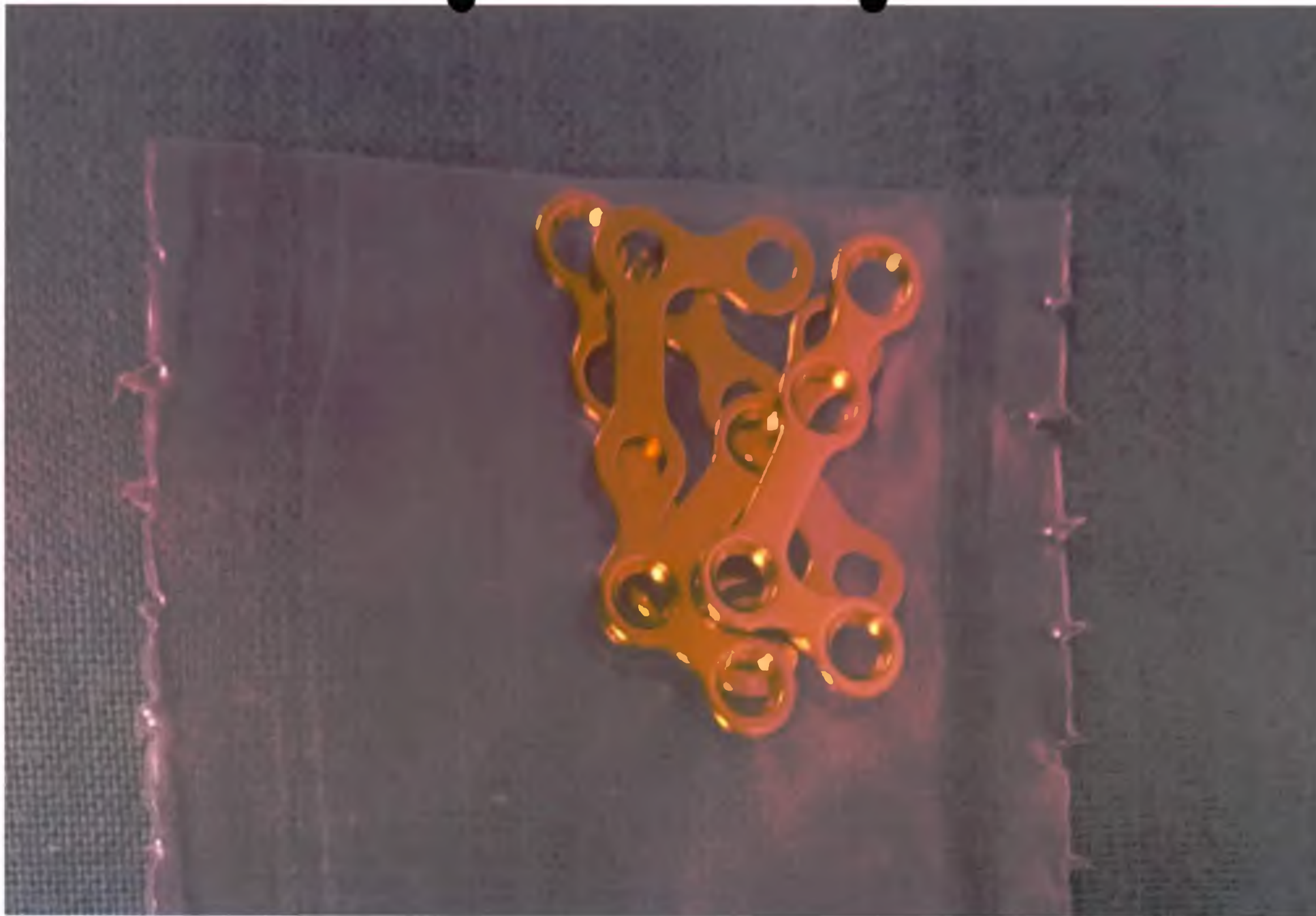
Мини-пластина L-образная правая, 4 отверстия, планка 9 мм, 0,6 мм x 2,0 мм. Представлена упаковка с 5 изделиями внутри
