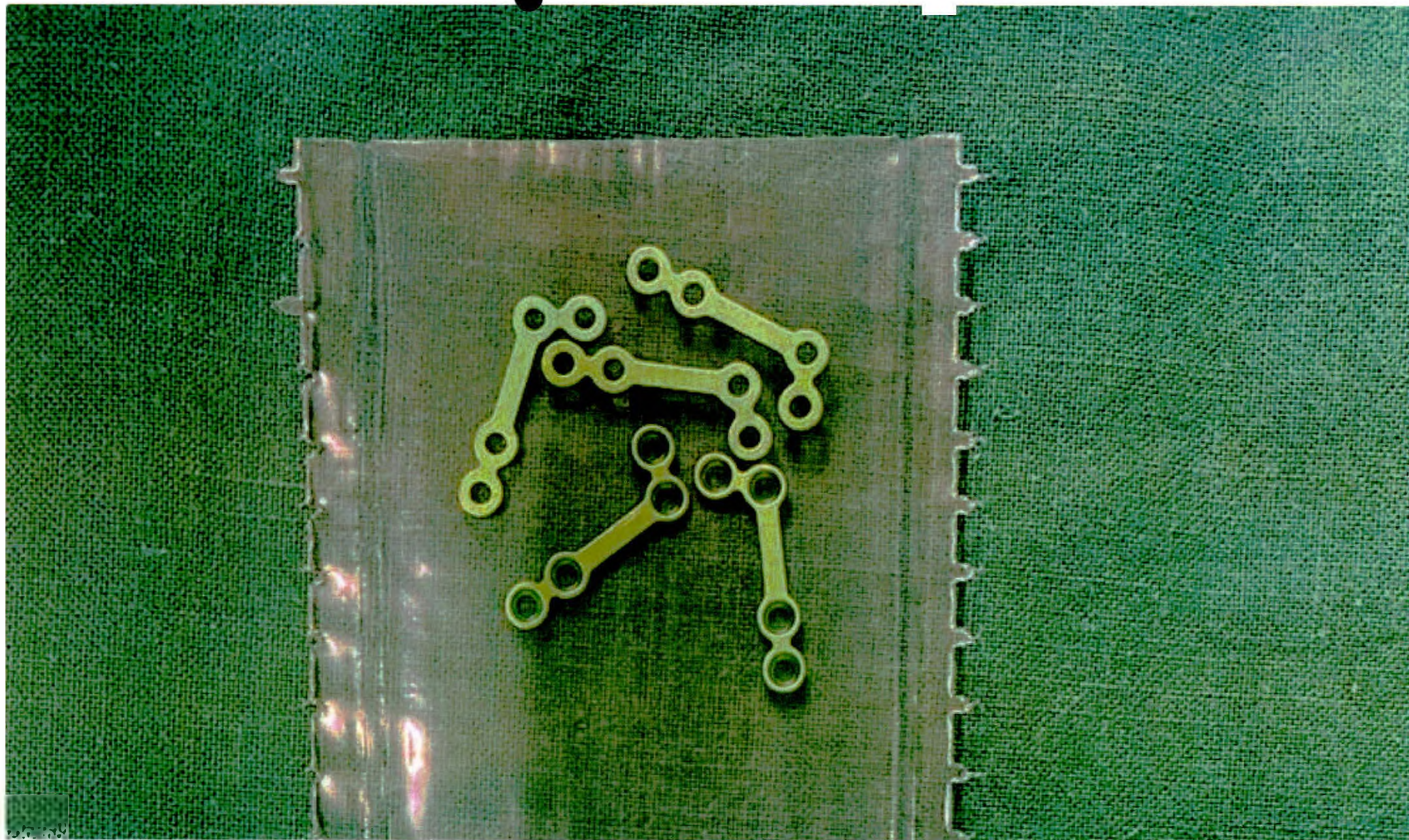
Медиум-пластина L-образная правая, под углом 110^\circ , 4 отверстия, планка 10 мм, 0,6 мм x 1,6 мм . На фотографии представлена упаковка с 5 пластинами внутри.
