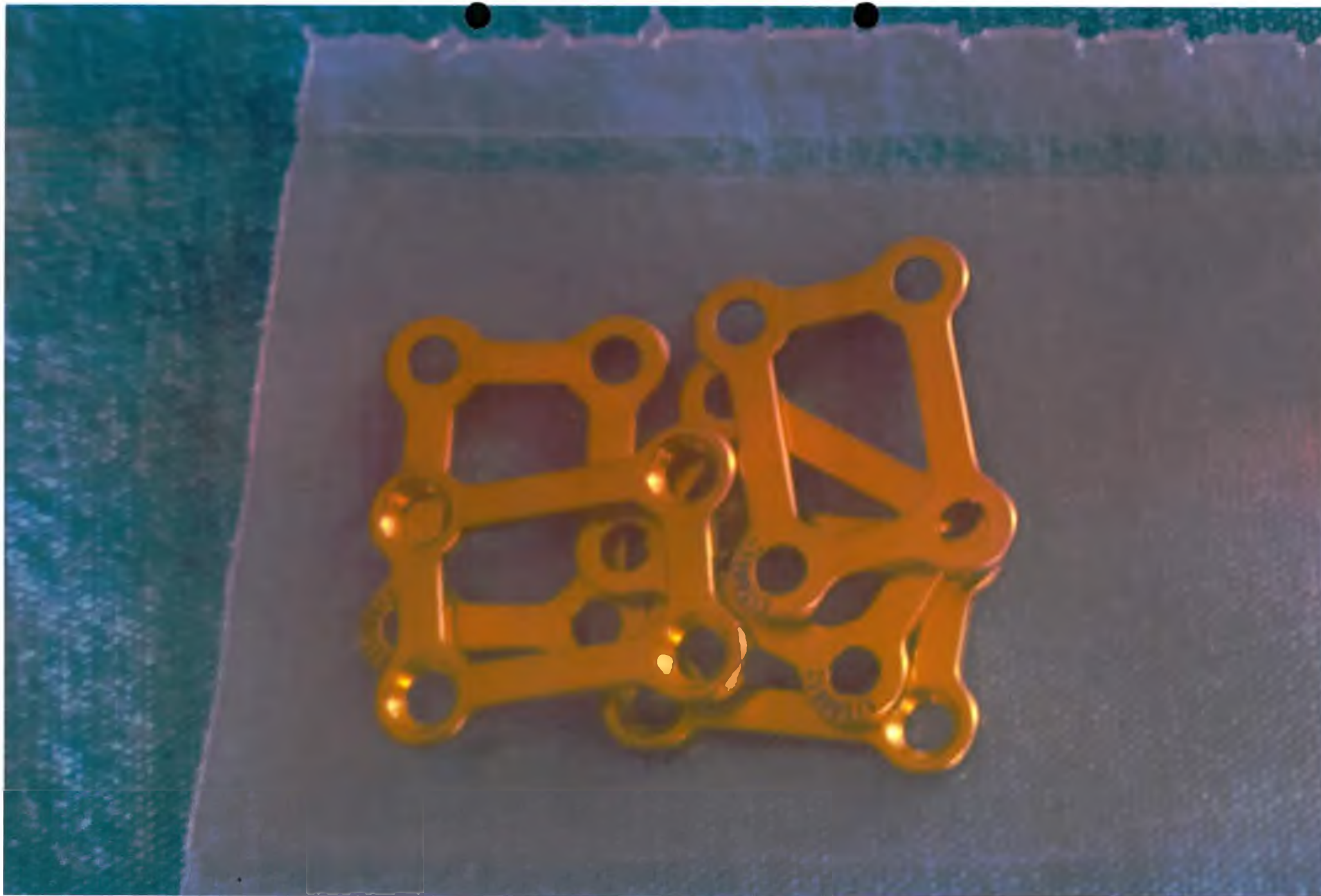
Мини-пластина прямоугольная, асимметричная, 4 отверстия (2x2), 1,0 мм x 2,0 мм. Представлена упаковка с 5 одинаковыми пластинами
