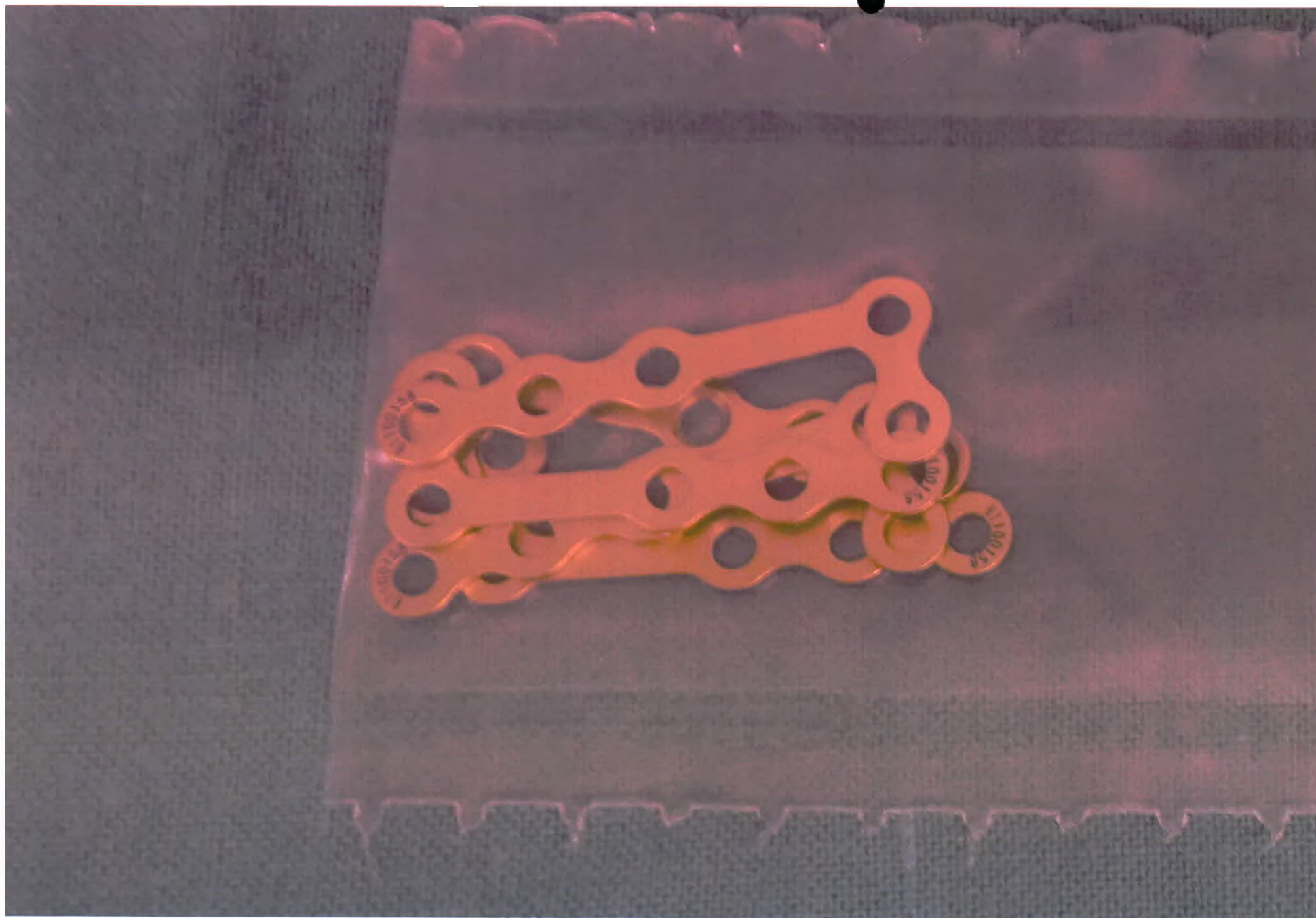
Мини-пластина L-образная правая, 5 отверстий, планка 12 мм, 0,6 мм х 2,0 мм. Представлена упаковка с 5 изделиями внутри
