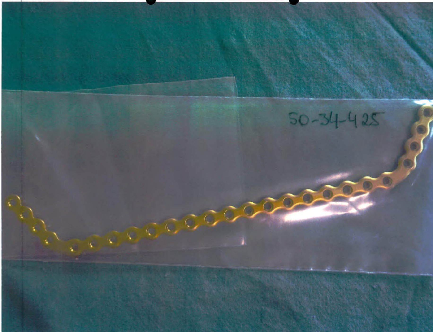
Пластина полная нижнечелюстная 4/17/4 отверстий, 2,7 мм
