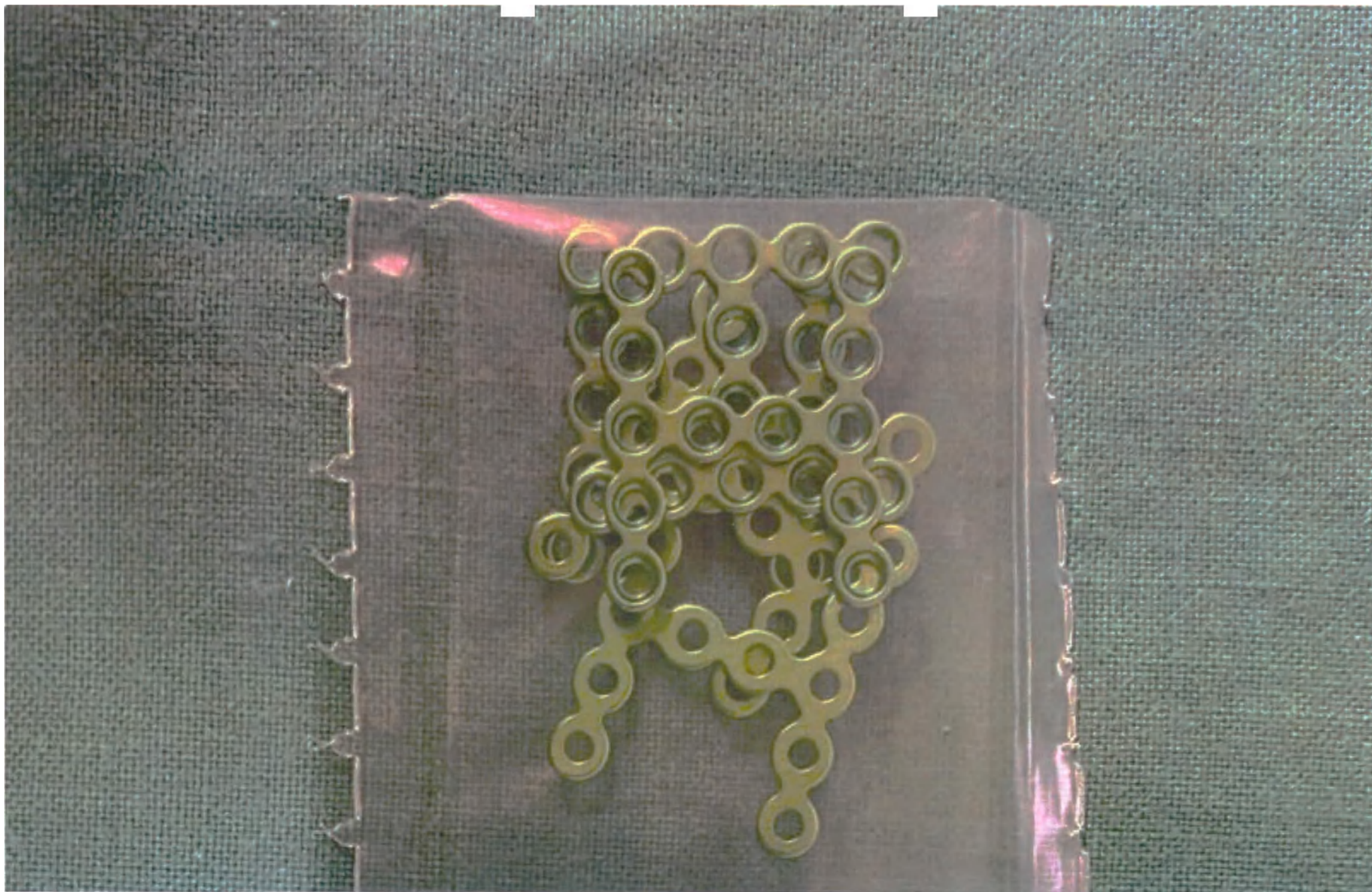
Медиум-пластина Т-образная двойная, 12 отверстий, 0,6 мм х 1,6 мм. На фотографии представлена упаковка с 5 пластинами внутри.
