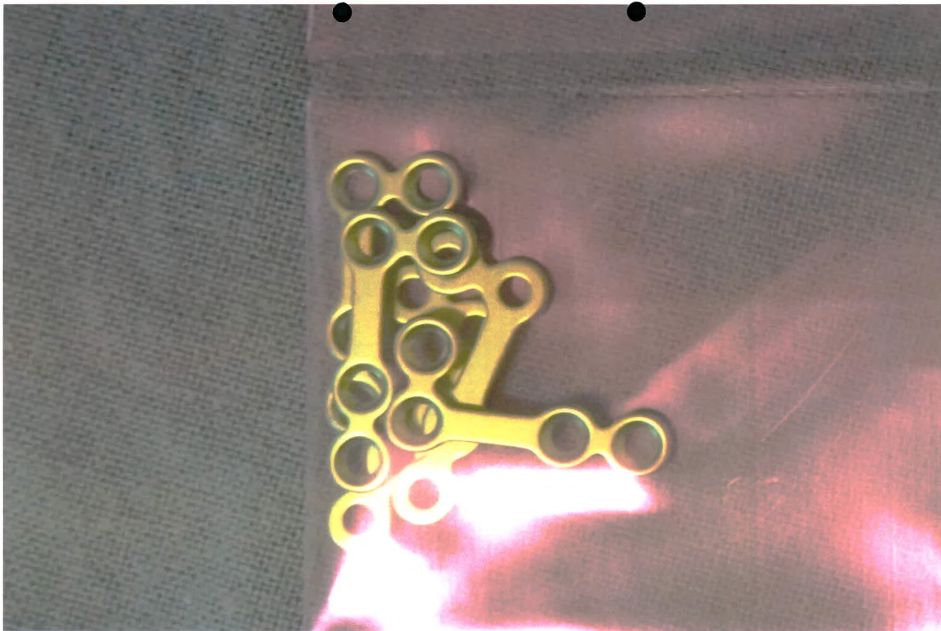
Медиум-пластина L-образная левая, 4 отверстия, планка 8 мм, 0,6 мм x 1,6 мм. Изображена упаковка с 5 изделиями
