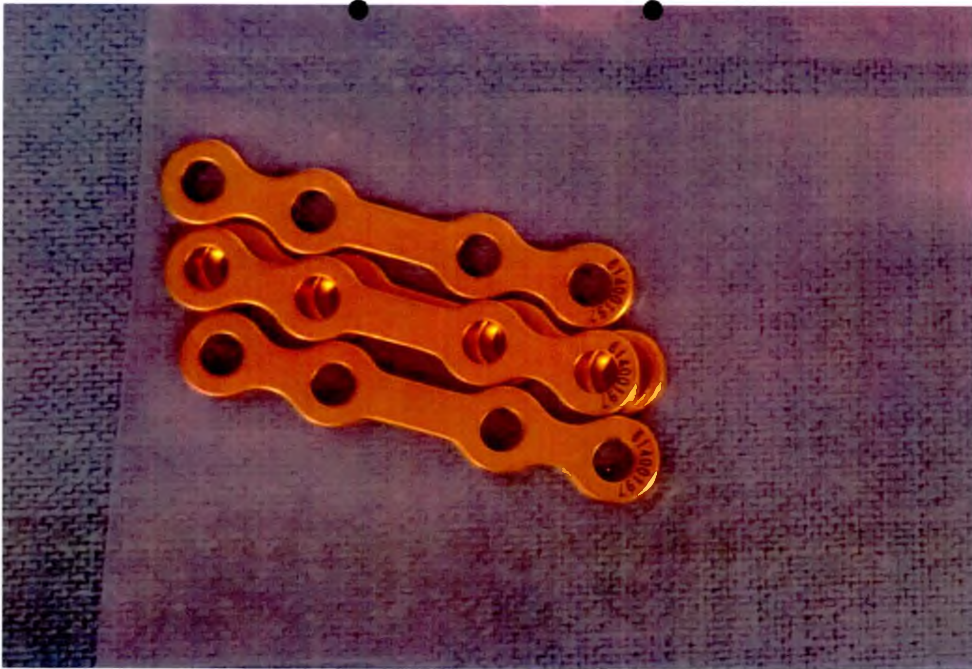
Мини-пластина прямая, 4 отверстия, планка 9 мм, 0,75 мм х 2,0 мм. Представлено 5 одинаковых изделий
