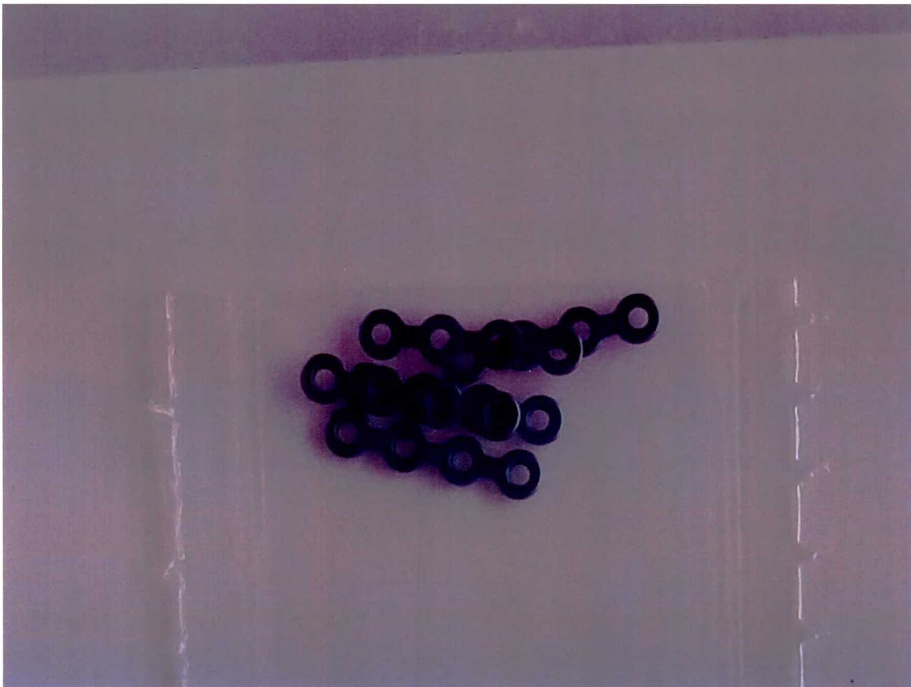
Микропластина прямая, 4 отверстия, 0,6 мм x 1,2 мм. На фотографии представлена упаковка с 5 пластинами внутри.
