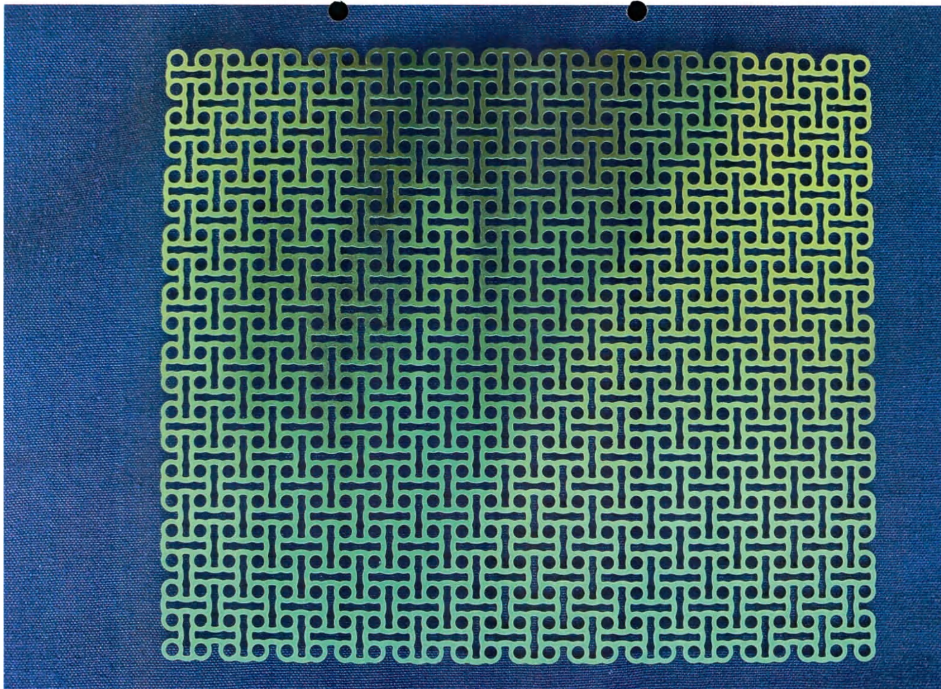
Пластина сетчатая для винтов 1.6 / 2.0, тип узора 4, 100 x 120 x 0,6 мм
