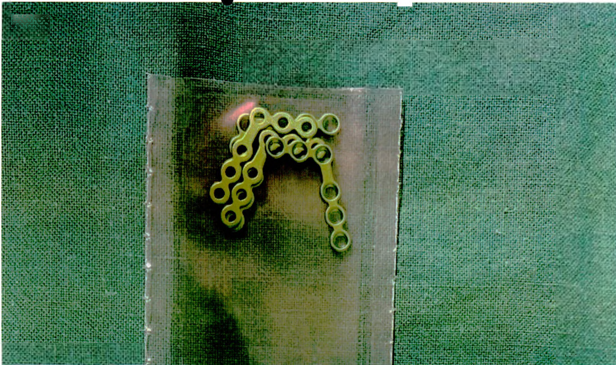
Медиум-пластина L-образная правая, под углом 110^\circ , 6 отверстий, планка 6 мм, 0,6 мм x 1,6 мм. На фотографии представлена упаковка с 5 пластинами внутри.
