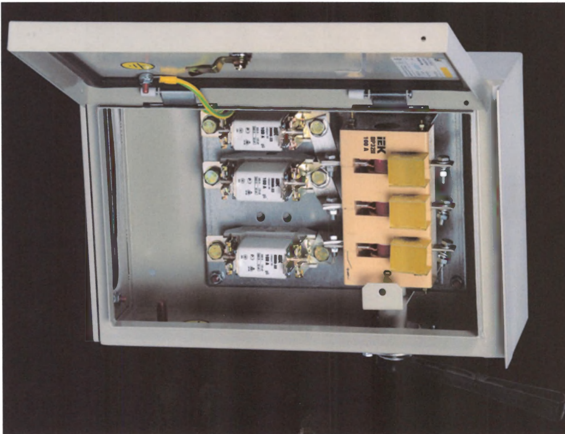
Щит распределительный
