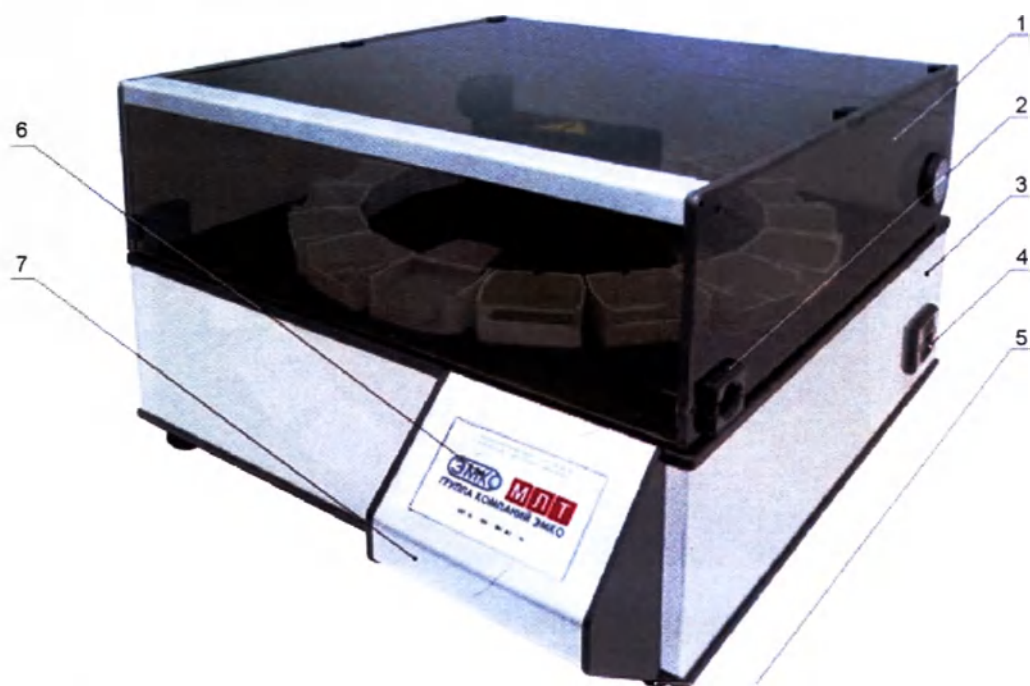
МЛБА 944330.005 -01 РЭ Рисунок 2 Общий вид прибора
