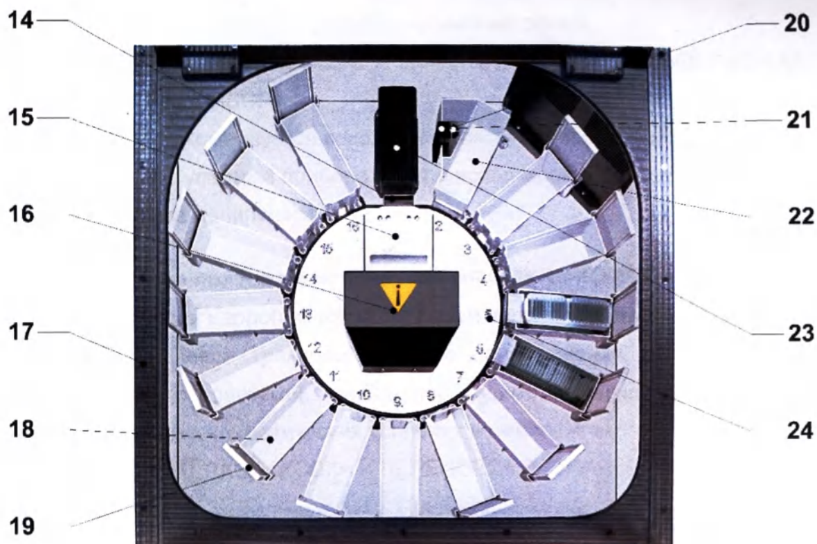
МЛБА 944330.005 -02 РЭ Рисунок 4. Внешний вид прибора, рабочая камера технологического блока, вид сверху
