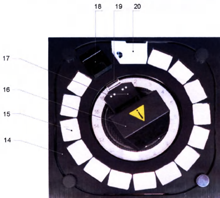
МЛБА 944330.005 -01 РЭ Рисунок 4. Внешний вид прибора, рабочая камера технологического блока, вид сверху
