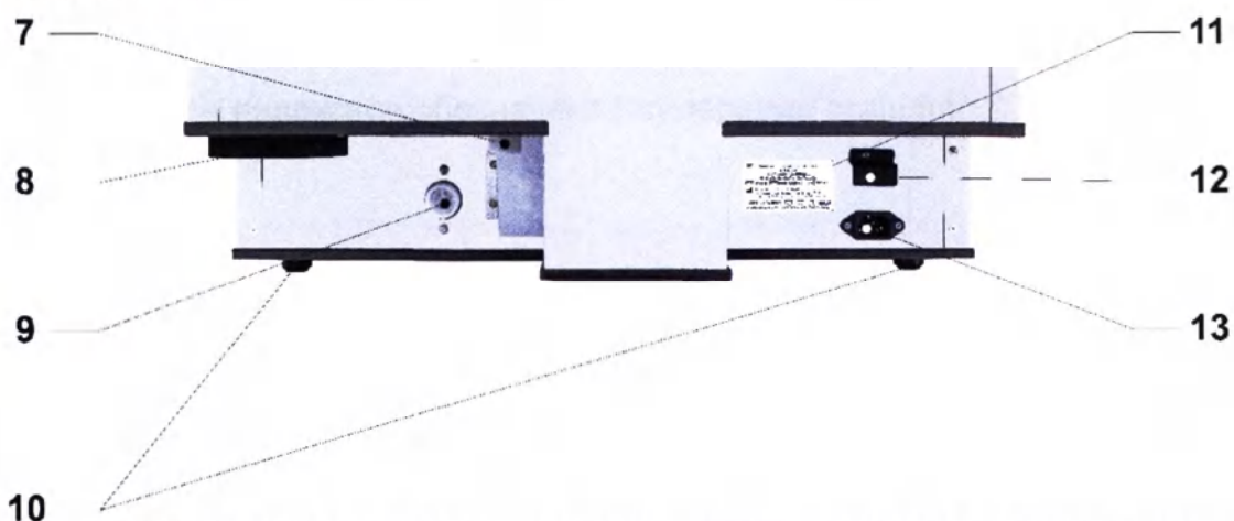
МЛБА 944330.005 -02 РЭ Рисунок 3. Внешний вид прибора, задняя панель:
