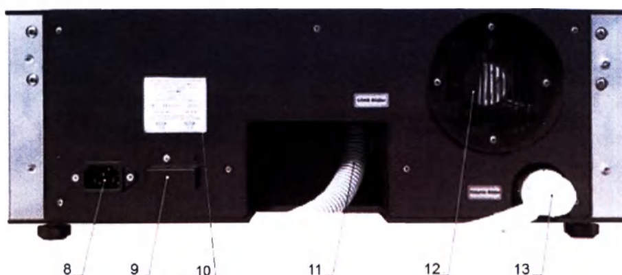
МЛБА 944330.005 -01 РЭ Рисунок 3. Внешний вид прибора, задняя панель:
