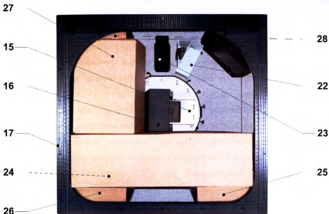
МЛБА 944330.005 -02 РЭ Рисунок 6. Распаковка прибора. Вид на рабочую камеру при открытой крышке.
