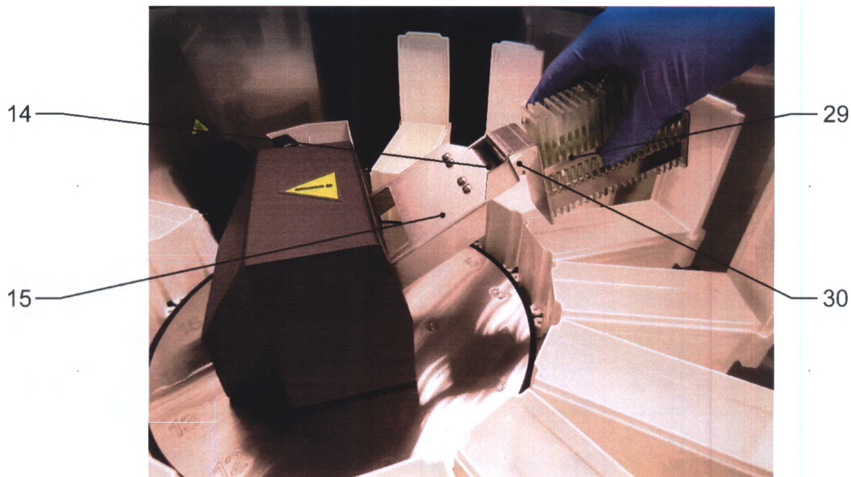
Рисунок 28. Загрузка и выгрузка штатива.
