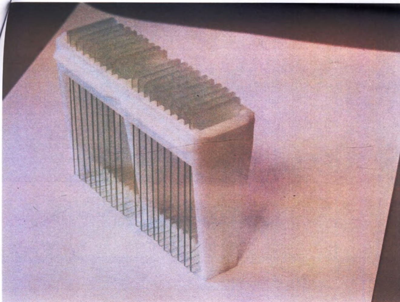
Штатив-кладыш для предметных стекол ШВВ-20 (07.00.02)
