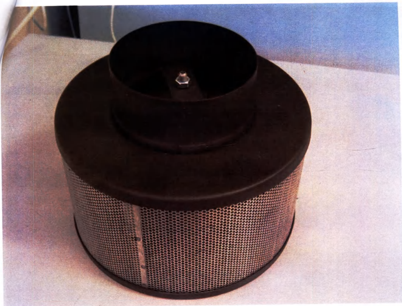
Фильтр угольный (05.04.00)
