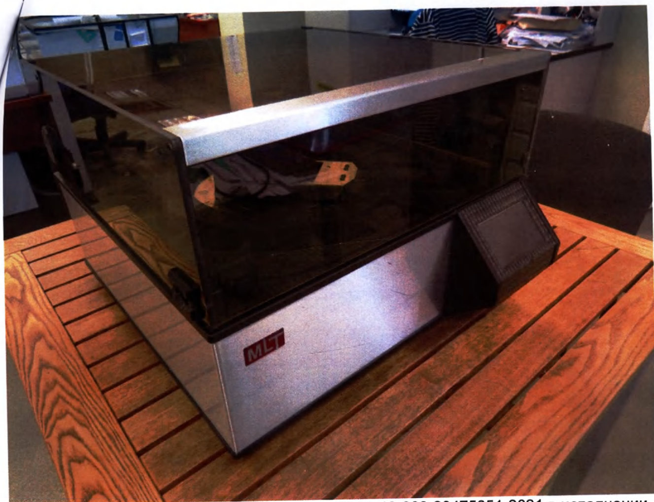
Автомат фиксации и окраски мазков по ТУ 26.60.12-003-23475651-2021 в исполнении АФОМК-16-ПРО
