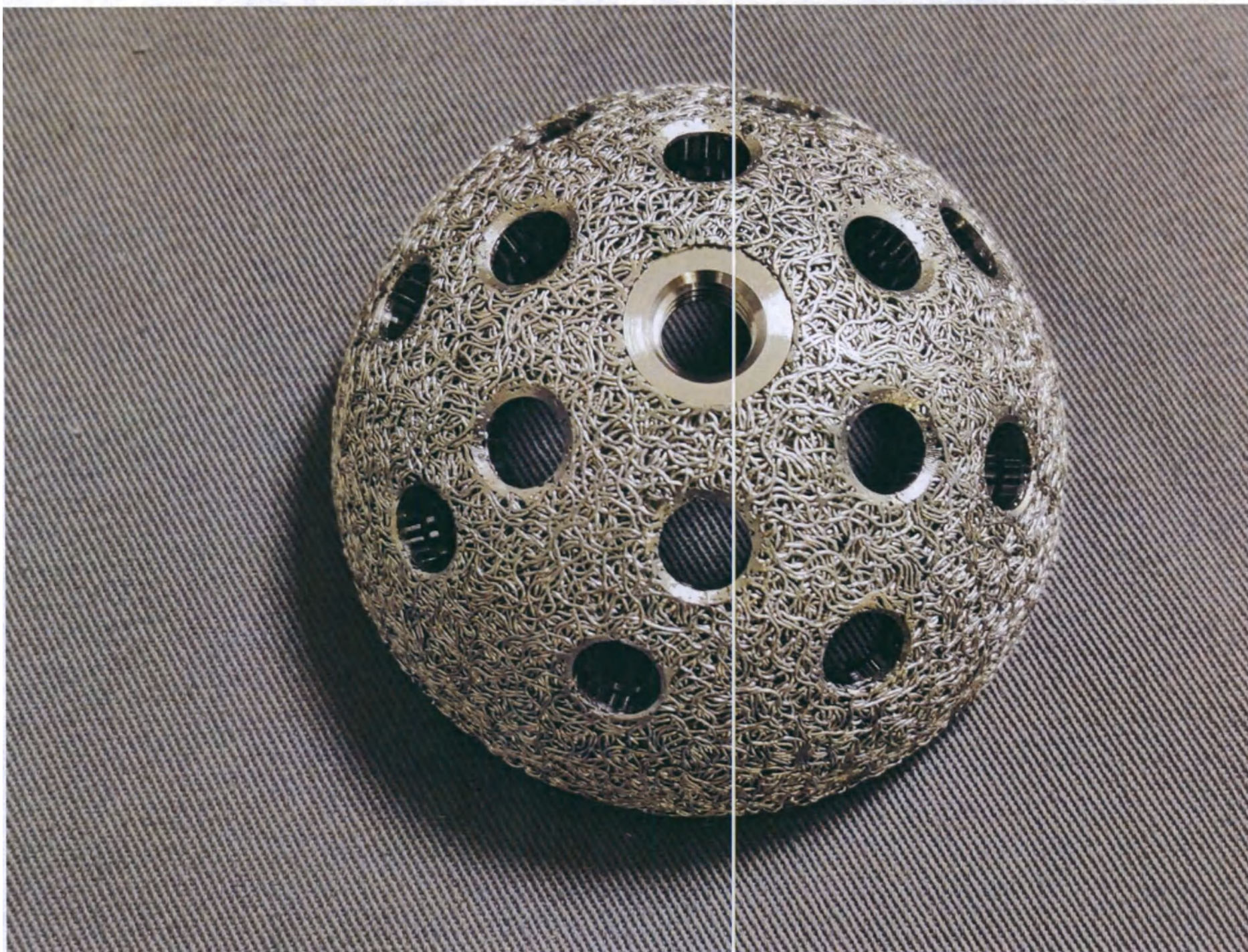
Рис. 9. Компонент вертлужный Fiber Metal многодырчатый (представлено изображение Компонент вертлужный Fiber Metal многодырчатый, размер
