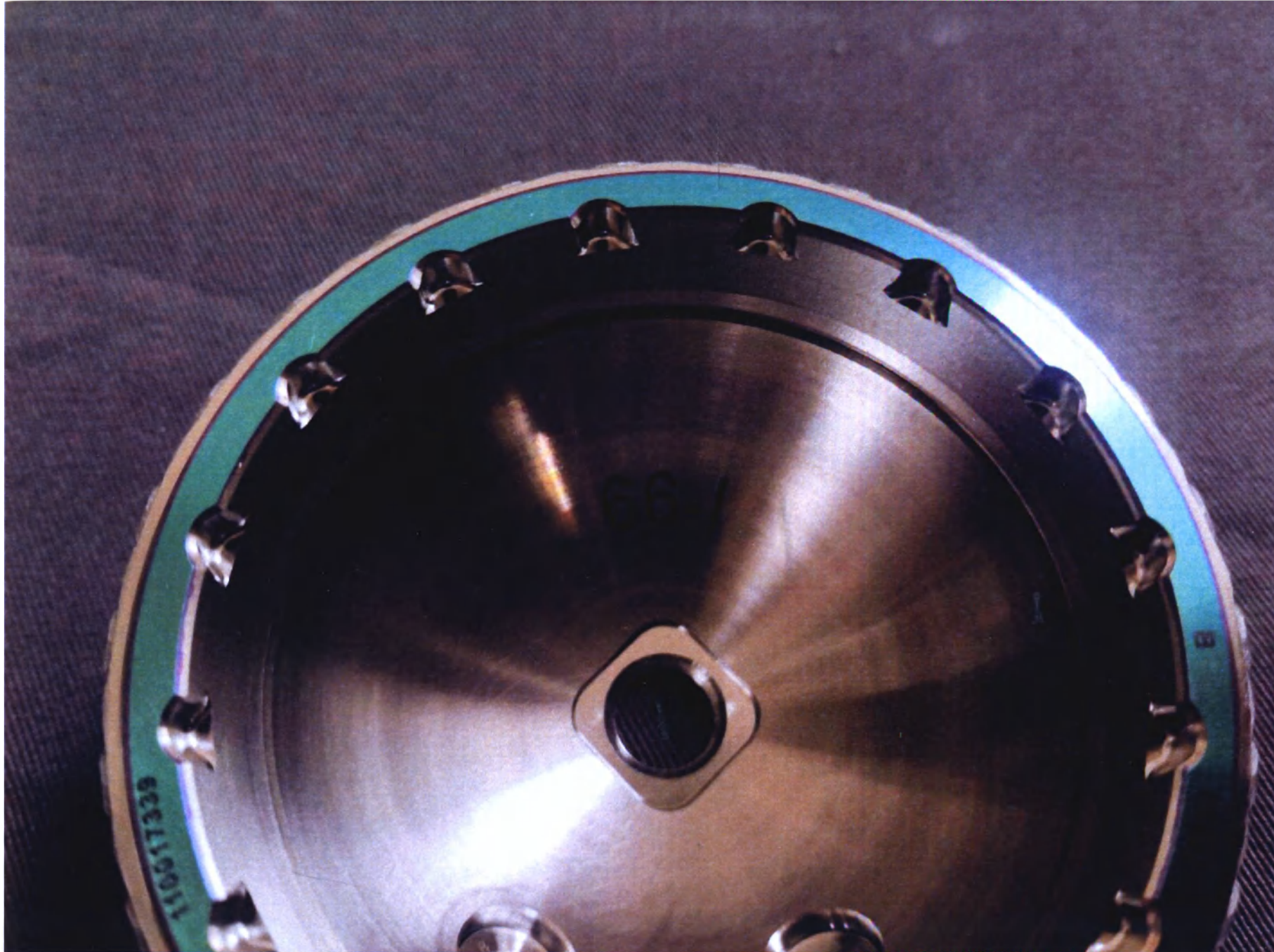
Рис. 2. Компонент вертлужный BiSpherical G7 бесцементный, 3 отверстия, размер 66 мм. I., вид снизу.
