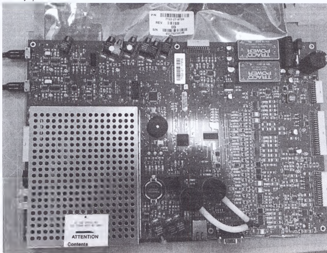
27. Плата управления.
