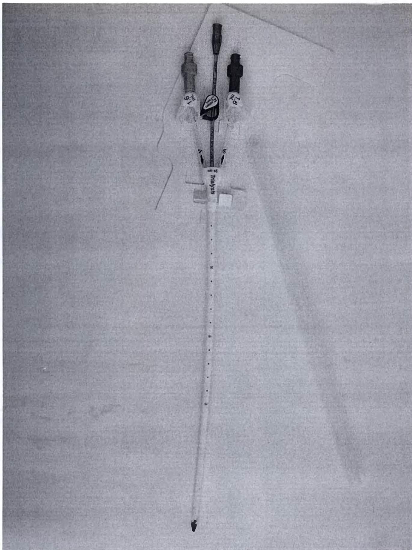
Катетер кратковременного использования для диализа прямой трехпросветный рентгеноконтрастный Power-Trialysis 13 F, длиной 15 см, или 20 см, или 24 см, или 30 см (рядом защитный колпачок)
