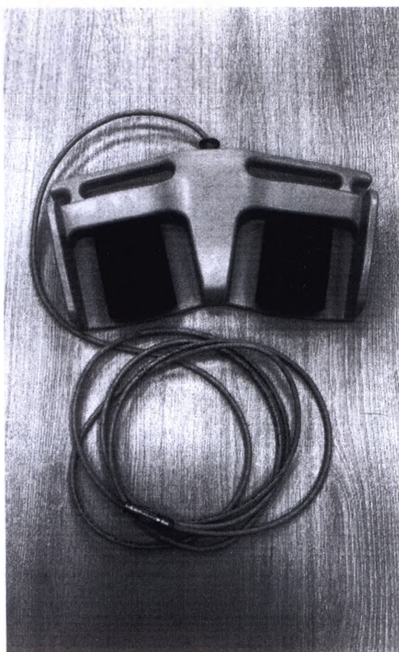
Педальный переключатель FSW01. Общий вид сверху
