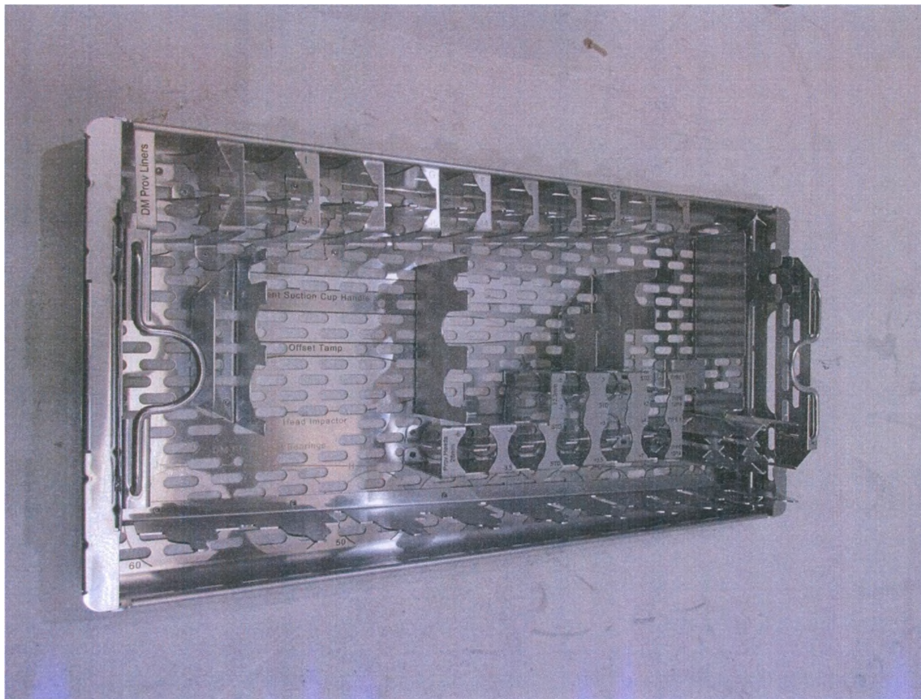
Рис. 14. Контейнер для инструментов G7 двойной мобильности.
