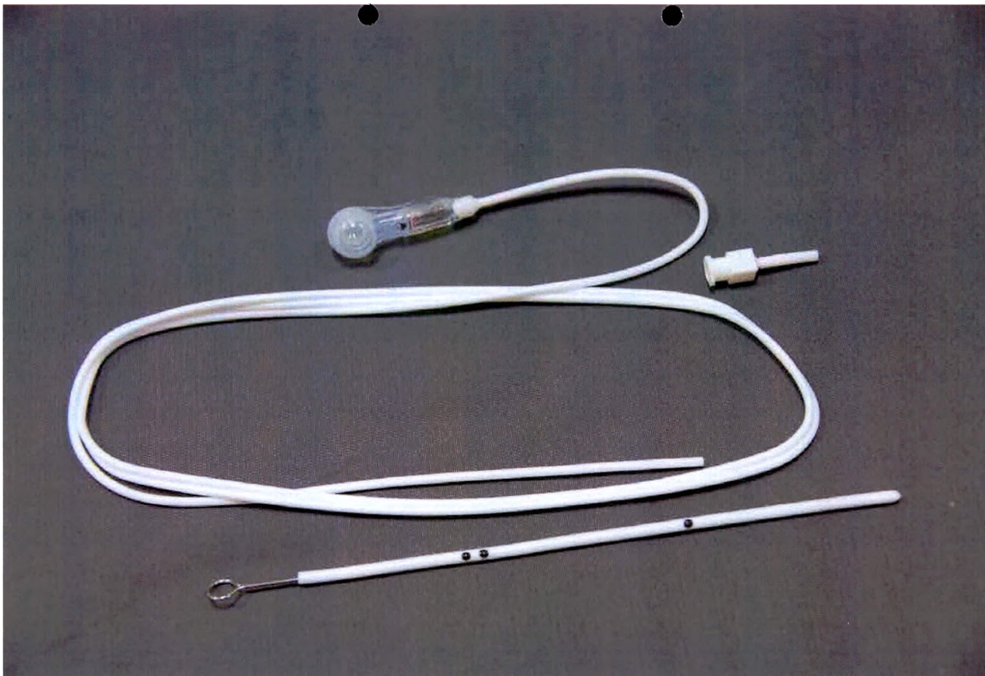
Клапан НАКИМ программируемого давления (артикул 82-3148), в составе: клапан (рабочее давление от 30 мм H 2 O до 200 мм H 2 O (294 Па - 1960 Па) с шагом 10 мм H 2 O (98 Па)) с угловым резервуаром соединенный с катетером перитонеальным (длина 120 см) – 1 шт.; катетер вентрикулярный с предустановленным стилетом (длина 14 см) – 1 шт.; адаптер для предварительного заполнения – 1 шт.
