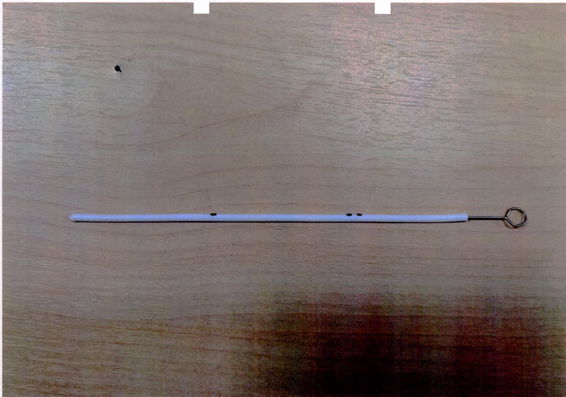
Катетер вентрикулярный с предустановленным стилетом (длина 14 см) из состава Клапана НАКИМ постоянного давления (артикул 82-3363)
