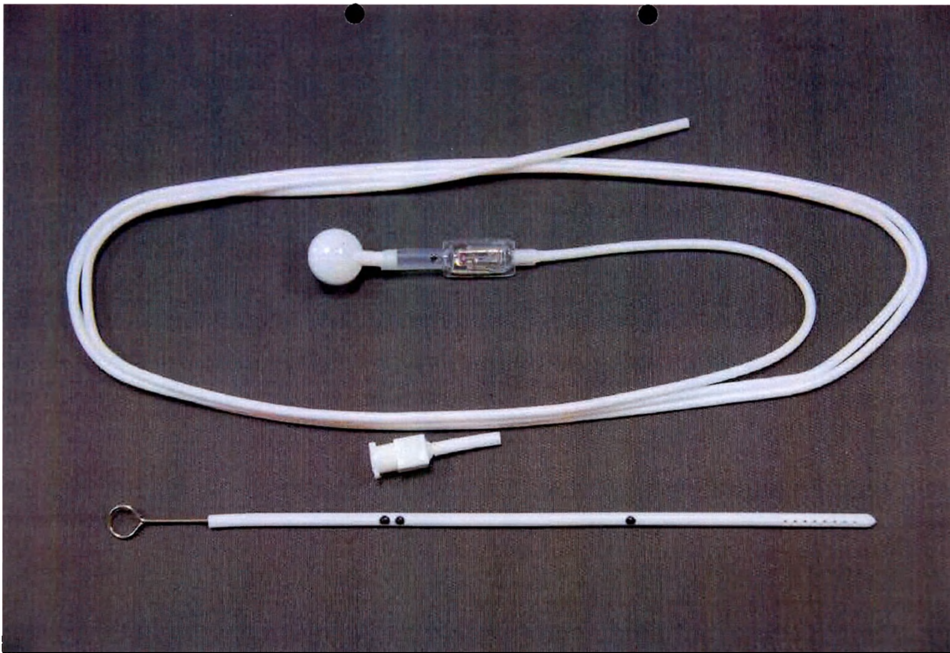
Клапан НАКИМ программируемого давления (артикул 82-3113), в составе: микроклапан (рабочее давление от 30 мм H 2 O до 200 мм H 2 O (294 Па - 1960 Па) с шагом 10 мм H 2 O (98 Па) с резервуаром RICKHAM, соединенный с катетером перитонеальным (длина 120 см) – 1 шт.; катетер вентрикулярный с предустановленным стилетом (длина 14 см) – 1 шт. ; адаптер для предварительного заполнения – 1 шт.
