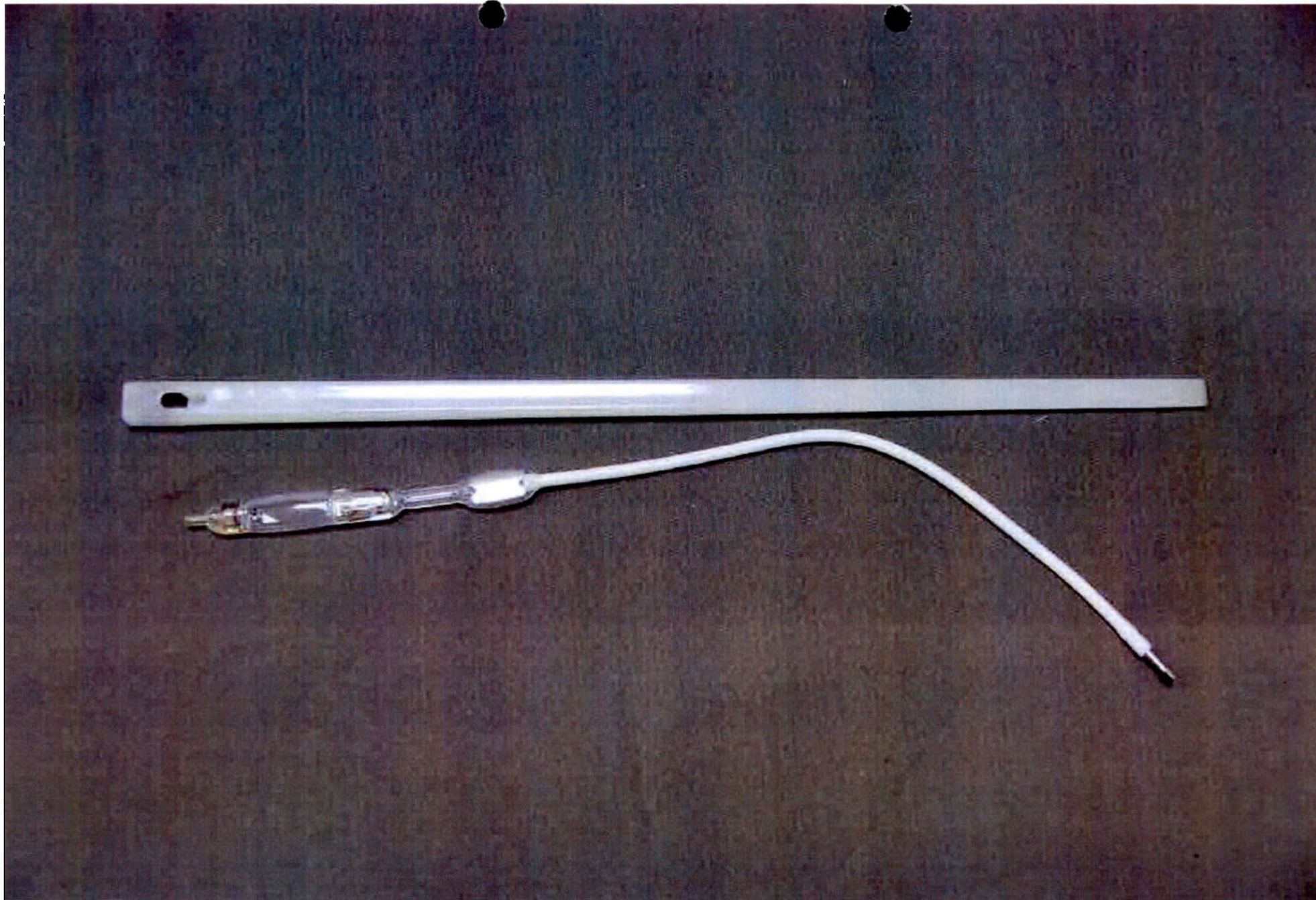
Клапан НАКТМ программируемого давления (артикул 82-3110), в составе: клапан цилиндрический с предкамерой (рабочее давление от 30 мм Н 2 О до 200 мм Н 2 О (294 Па - 1960 Па), с шагом 10 мм Н 2 О (98 Па)) – 1 шт.; интродьюсер – 1 шт.; коннектор прямой – 1 шт.
