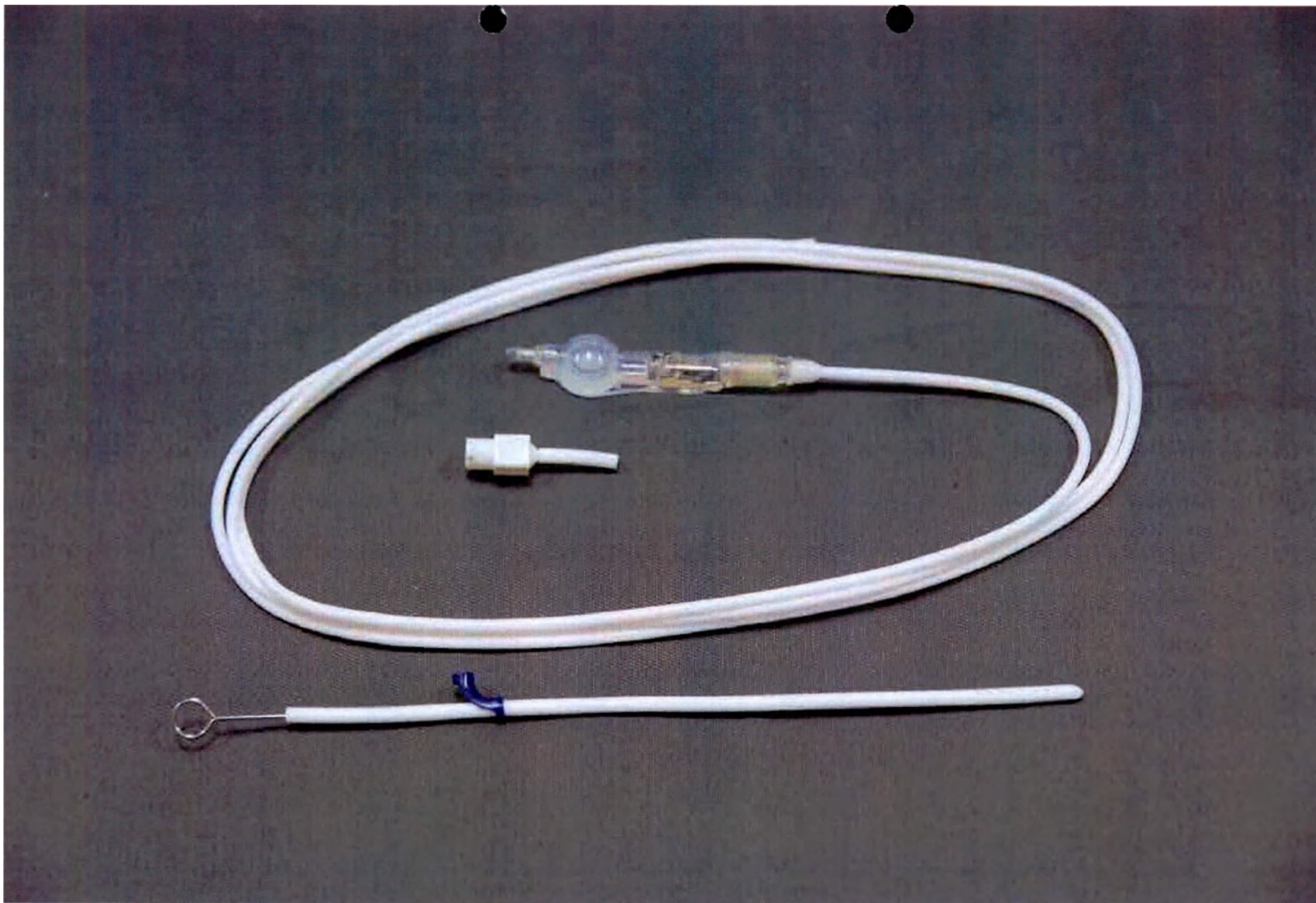
Клапан НАКИМ программируемого давления (артикул 82-3842), в составе: клапан (рабочее давление от 30 мм H 2 O до 200 мм H 2 O (294 Па - 1960 Па) с шагом 10 мм H 2 O (98 Па)) с прямоточным резервуаром и устройством SIPHONGUARD, соединенный с катетером перитонеальным (длина 120 см) – 1 шт.; катетер вентрикулярный с предустановленным стилетом (длина 14 см) – 1 шт.; адаптер для предварительного заполнения – 1 шт.; адаптер угловой – 1 шт.
