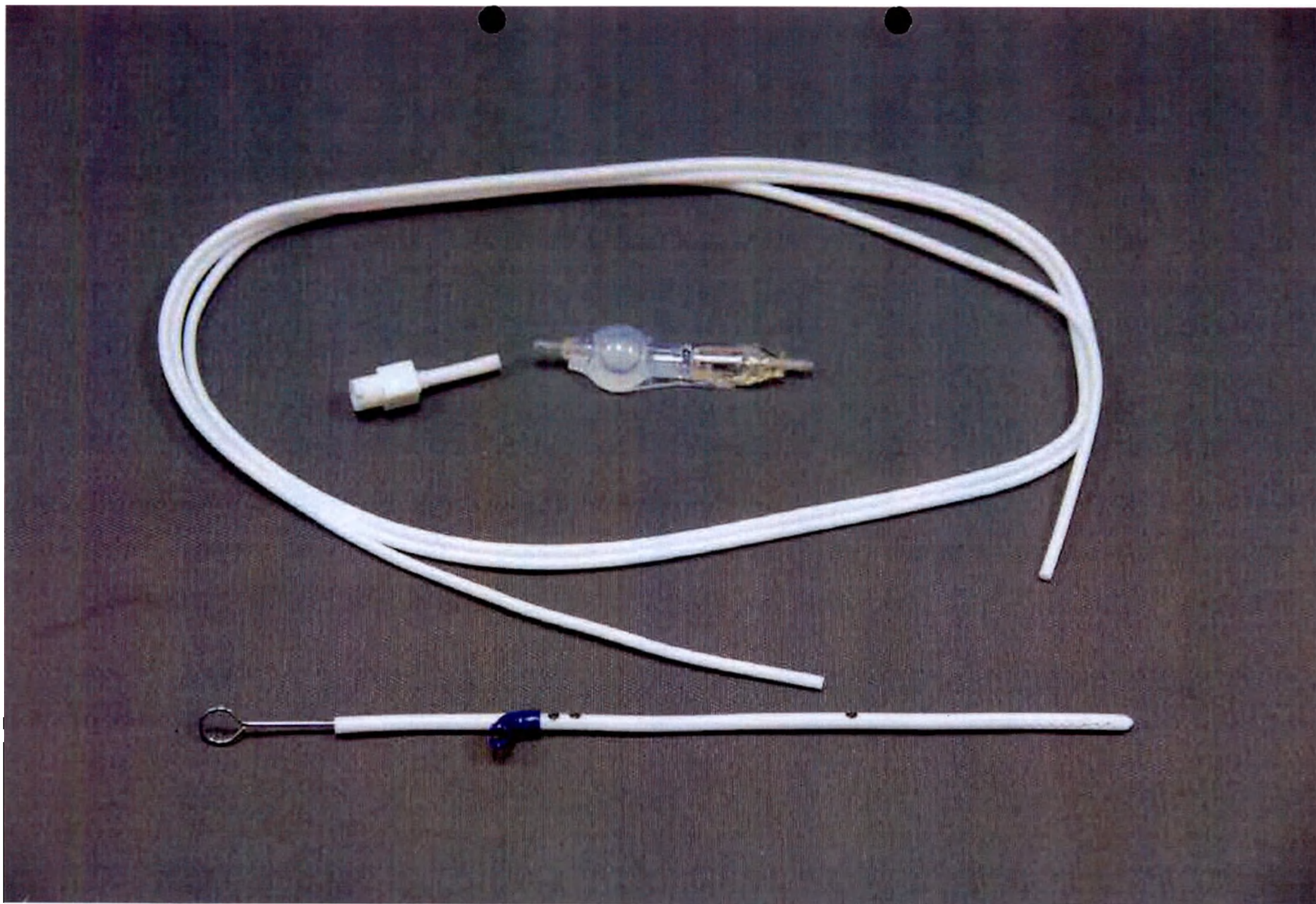
Клапан НАКІМ програмуемого давления (артикул 82-3834), в составе: клапан (рабочее давление от 30 мм H 2 O до 200 мм H 2 O (294 Па - 1960 Па) с шагом 10 мм H 2 O (98 Па)) с прямоточным резервуаром – 1 шт.; катетер перитонеальный (длина 120 см) – 1 шт.; катетер вентрикулярный с предустановленным стилетом (длина 14 см) – 1 шт.; адаптер для предварительного заполнения – 1 шт.; адаптер угловой – 1 шт.
