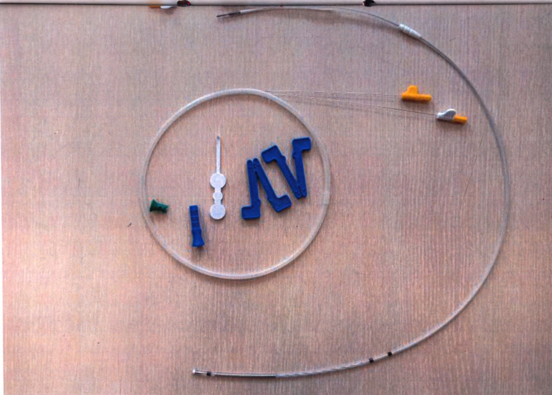
Вариант исполнения «I. Электрод дефибриллирующий эндокардиальный Plexa ProMRI S DX, модель Plexa ProMRI S DX 65/15», Вариант исполнения «II. Электрод дефибриллирующий эндокардиальный Plexa ProMRI S DX, модель Plexa ProMRI S DX 65/17» –
