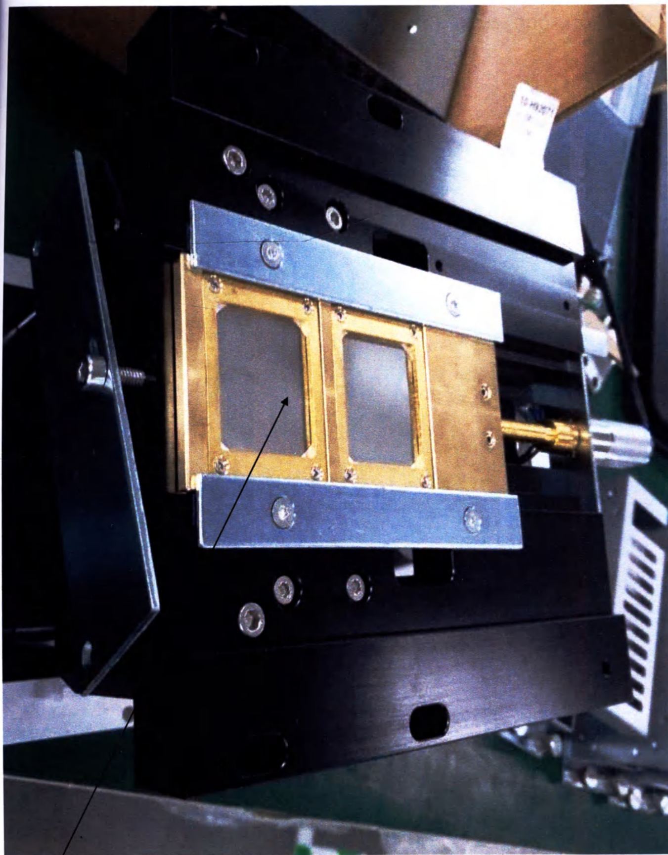
Устройство смены фильтров с электроприводом
