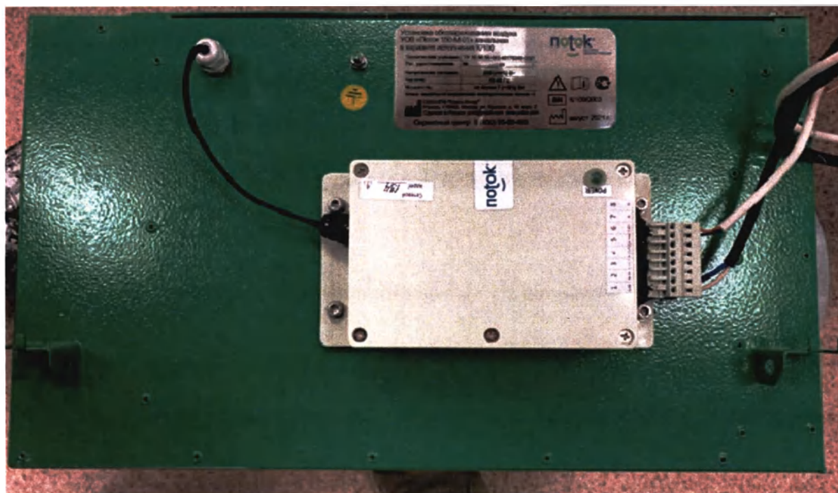
Установка обеззараживания воздуха УОВ «Поток 150-М-01» канальная (Различие вариантов исполнения только в габаритах)
