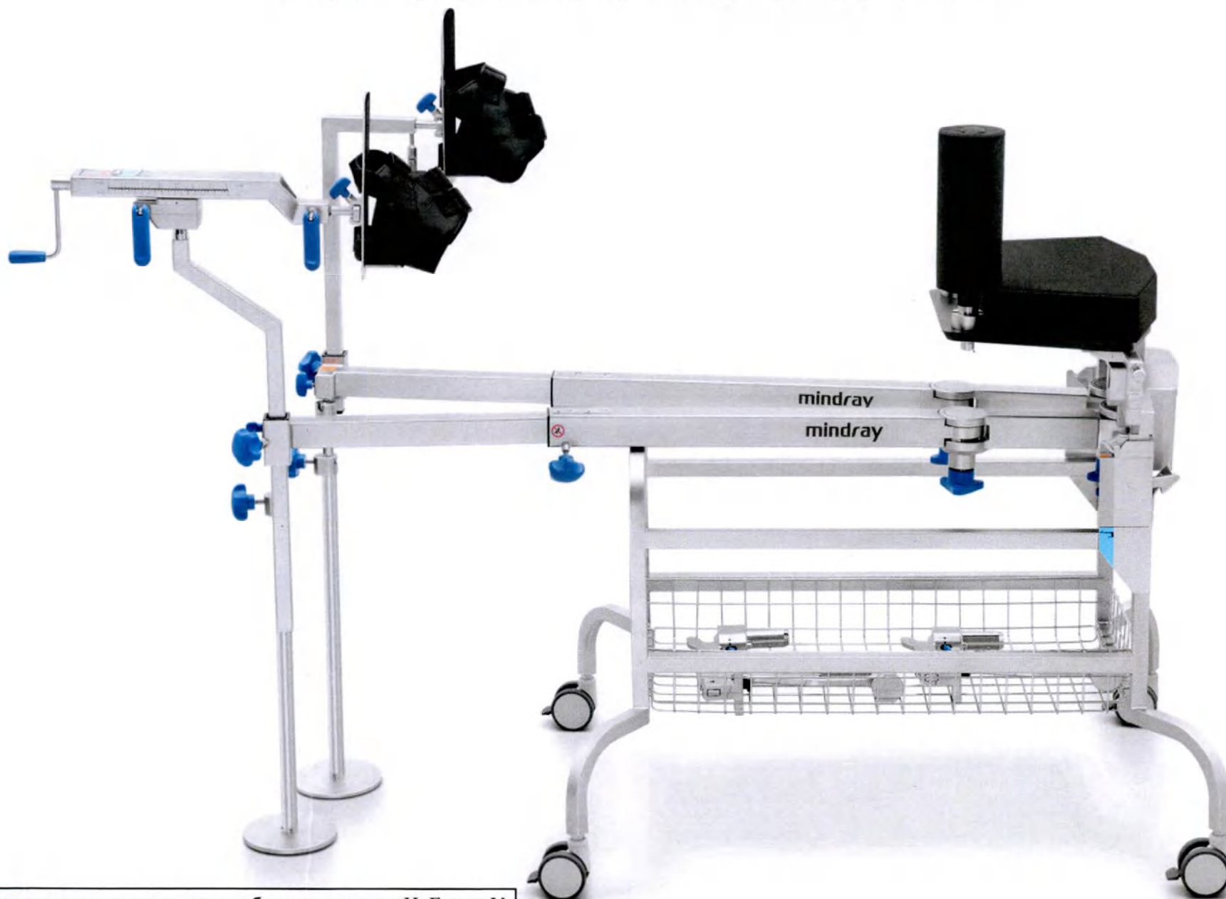
Стол операционный универсальный, электрогидравлический серии HyBase V, с принадлежностями
