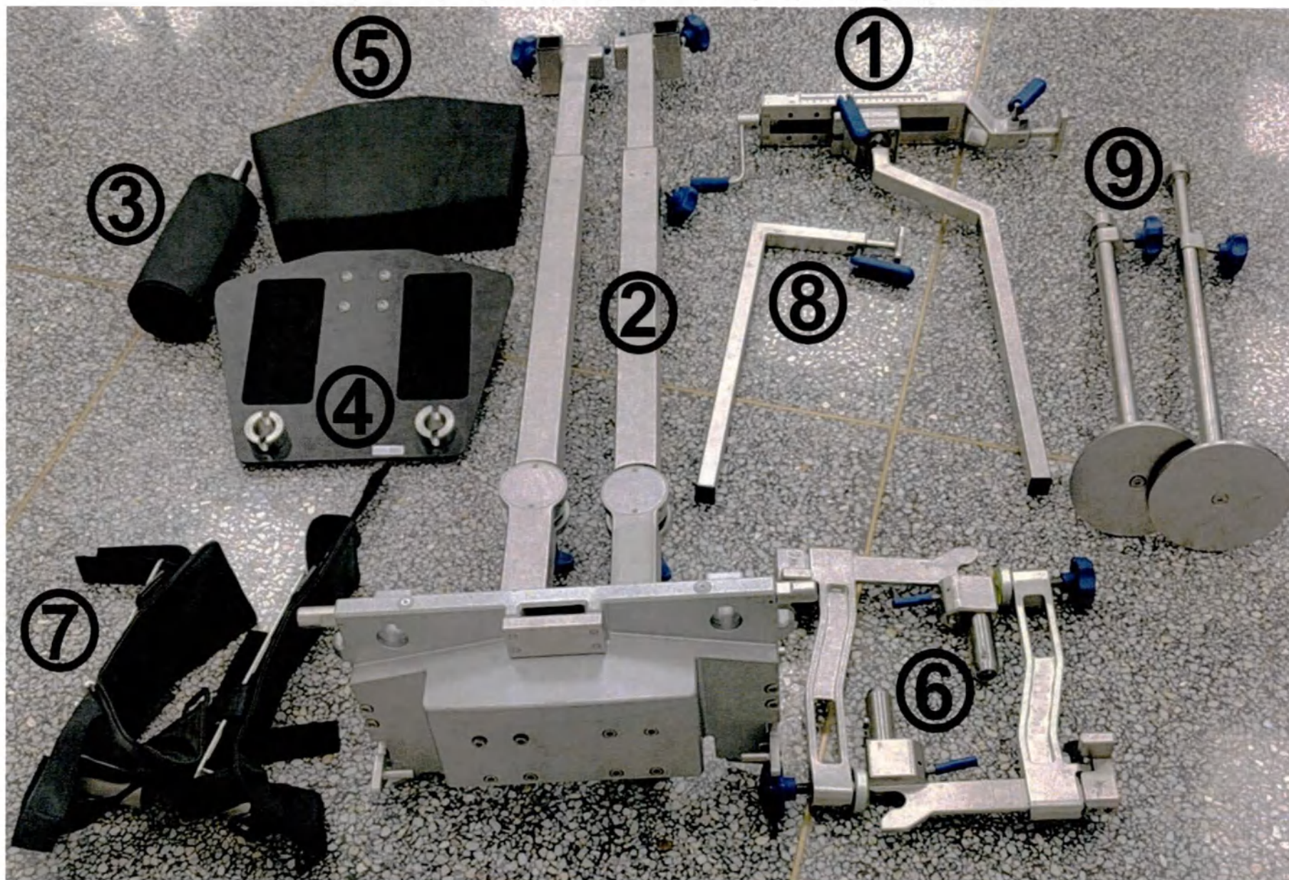
Секция вытяжения ортопедическая базовая, модель: HyExtent-V, в составе: 1. Механизм вытяжения - 1 шт., 2. Направляющая горизонтальная с шарнирным соединением - 1 шт., 3. Упор противотяговый - 1 шт., 4. Секция тазовая - 1 шт., 5. Матрас для секции тазовой - 1 шт., 6. Адаптер - 2 шт., 7. Ботинок базовый - 2 шт., 8. Опора поддерживающая для ботинка - 1 шт., 9. Стойка вертикальная поддерживающая - 2 шт. Для Стол операционный универсальный, электрогидравлический, в вариантах исполнения HyBase V8, HyBase V80, HyBase V8 Classic, HyBase V80 Classic.
