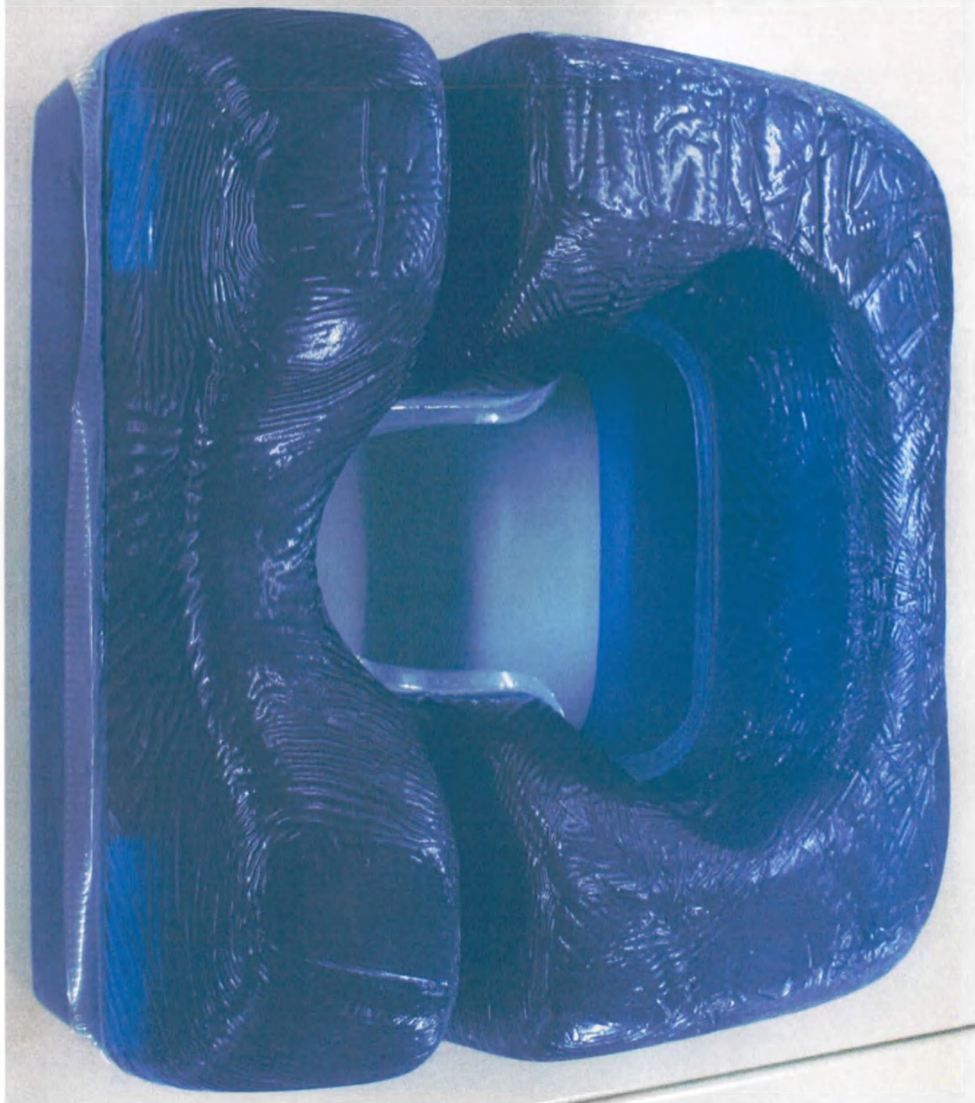
Стол операционный универсальный, электрогидравлический серии HyBase V, с принадлежностями
