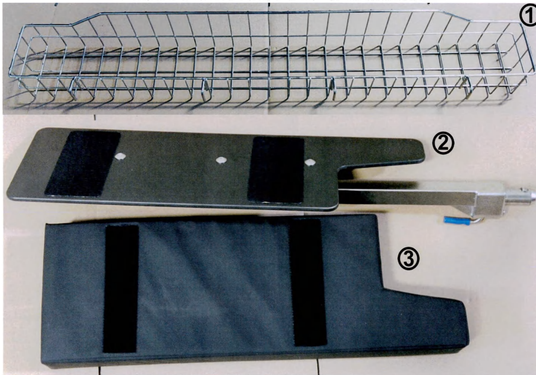
1. Корзина проволочная боковая (одна штука). 2. Секция ножная, вспомогательная, правая. 3. Матрас для секции ножной, вспомогательной, правой. Для Секция ножная, вспомогательная, для секции вытяжения ортопедической HyExtent-V, модель: A88XX. Для Стол операционный универсальный, электрогидравлический, в вариантах исполнения HyBase V8, HyBase V80, HyBase V8 Classic, HyBase V80 Classic.
