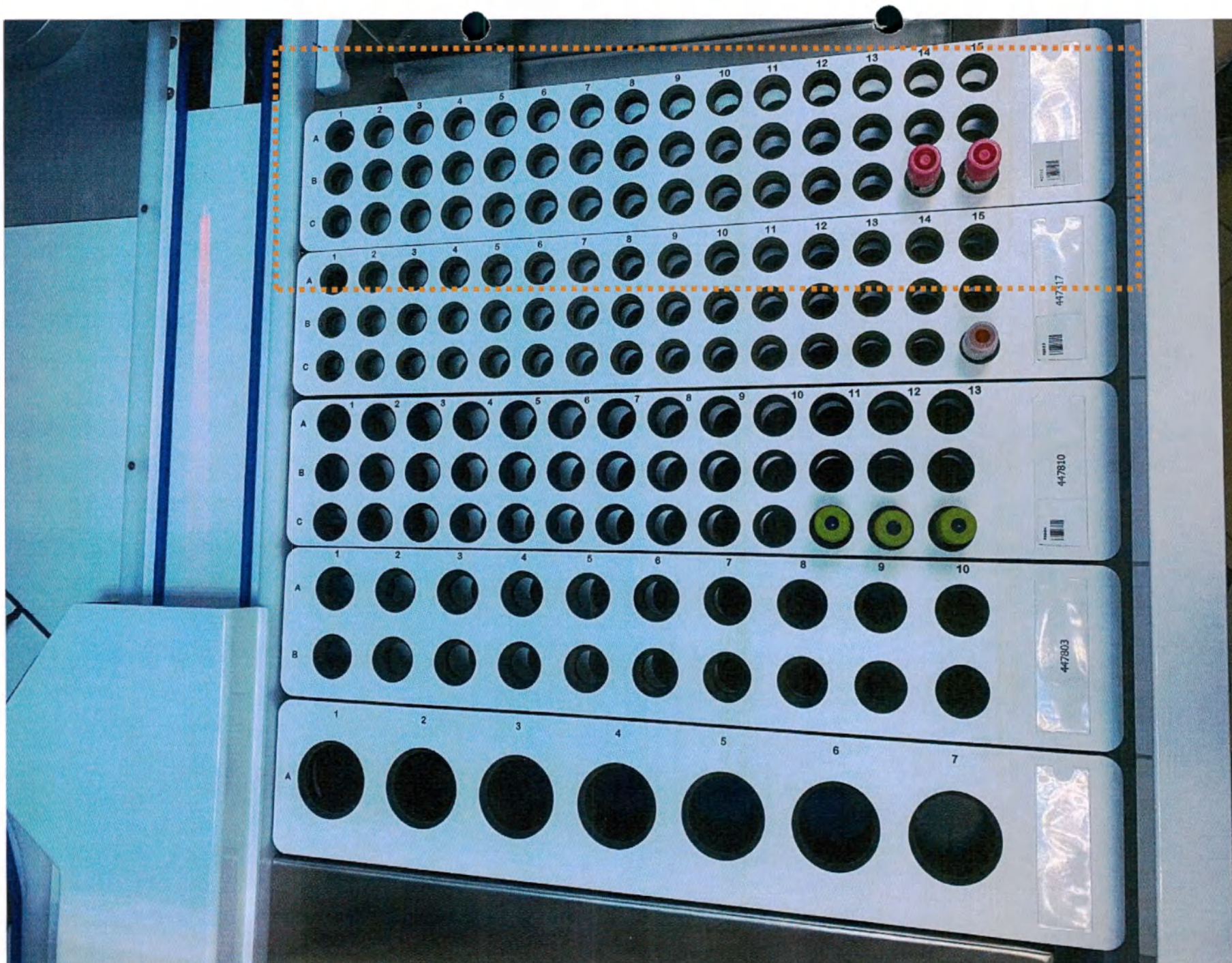
Штатив для контейнеров с образцами и пробирок с бульоном на 45 ячеек, тип 1 (верхний на представленном изображении)
