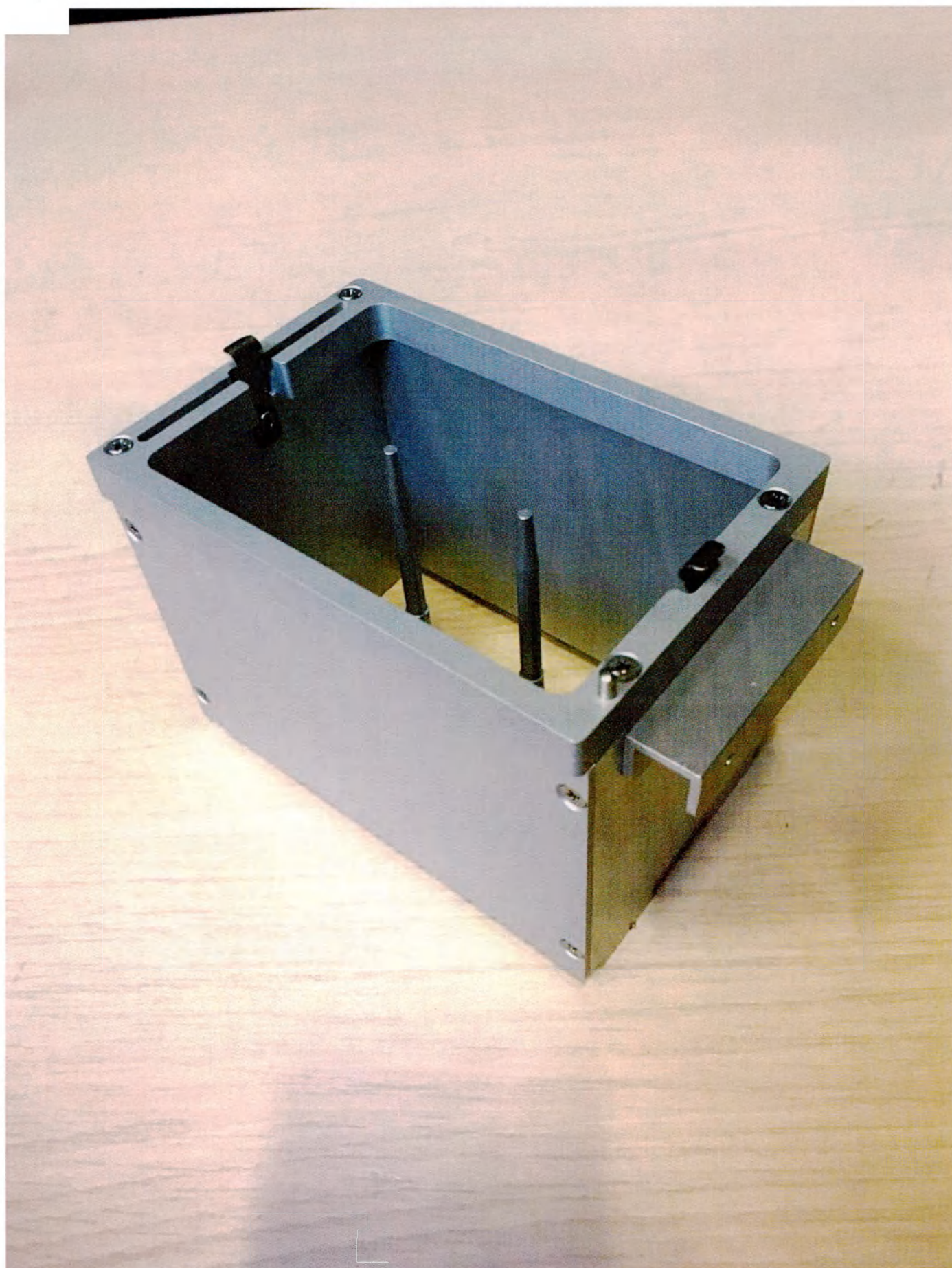
Держатель штативов для наконечников пипеток
