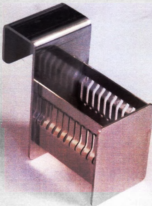
Штатив для праметных стекол ШВ-10 (06.08.00)
