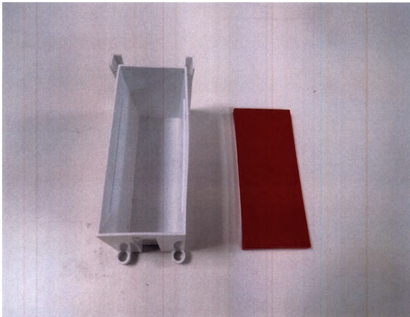
Ванна для реагентов ВВ-25 ПП с крышкой
