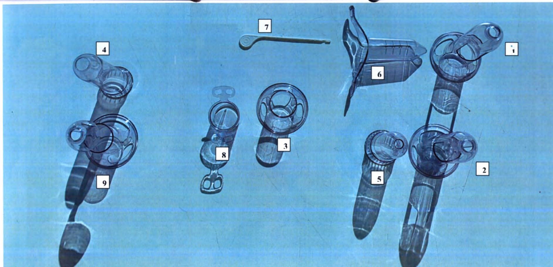
Фото 2 – Внешний вид комплектующих степлера циркулярного геморроидального, с головкой диаметром 33 мм (TST33-S180) где:
