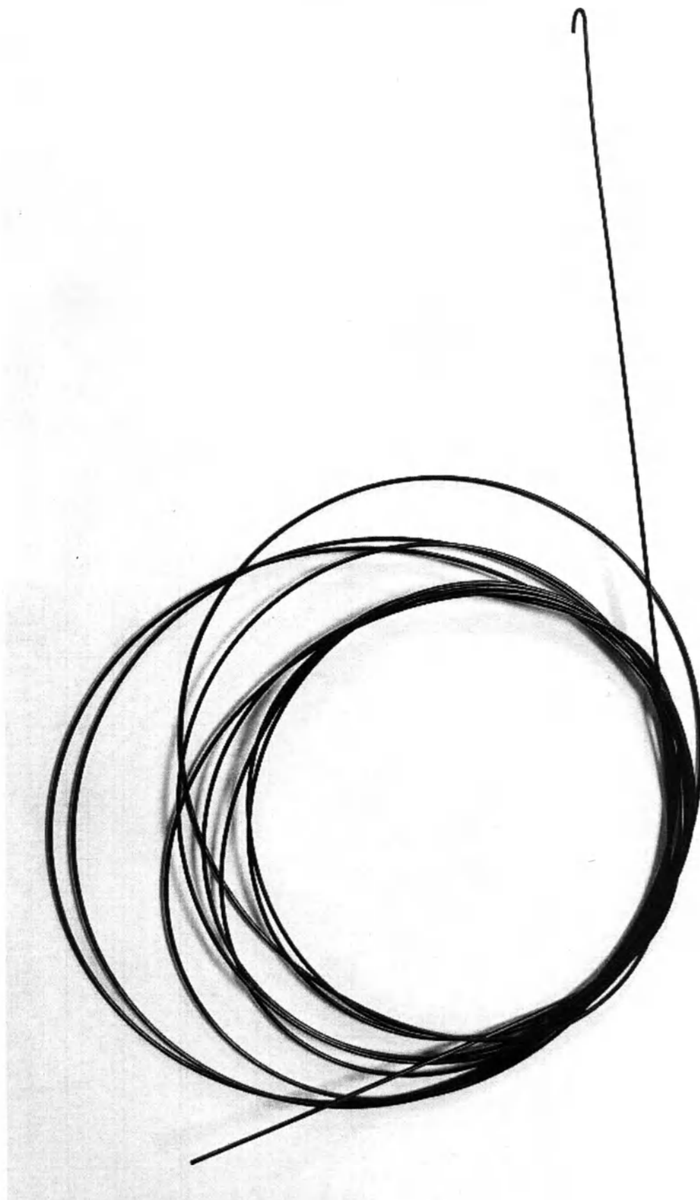
Рис. 6 – Проводник RADIFOCUS® GUIDE WIRE для сосудистых вмешательств, вариант исполнения Проводник RADIFOCUS® GUIDE WIRE M (вне защитной оболочки)
