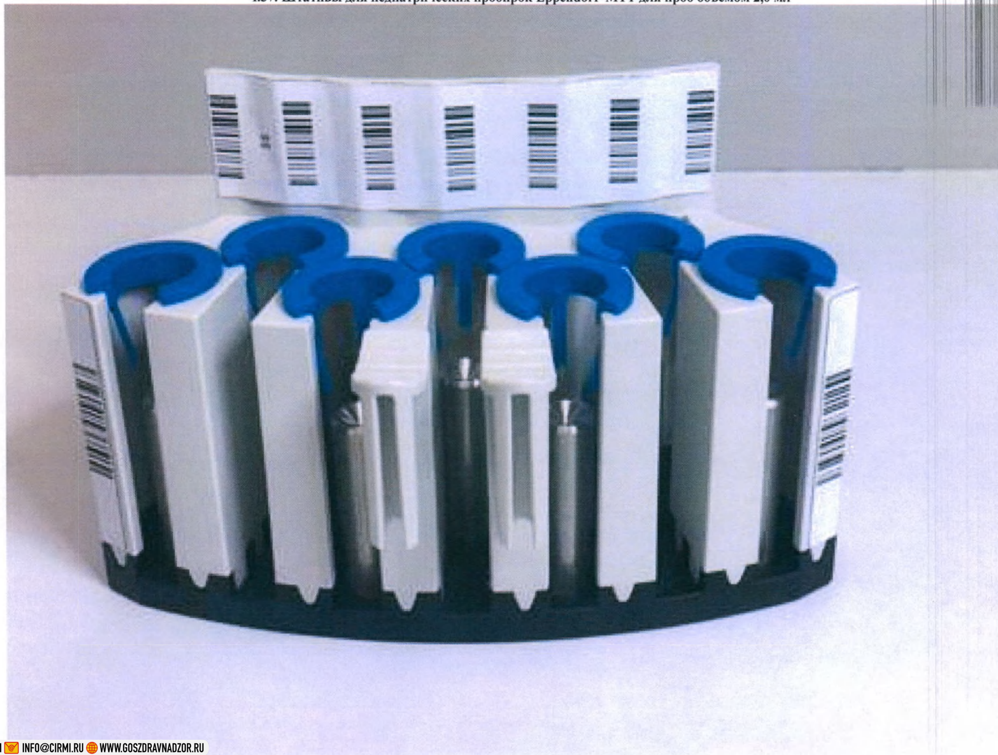
1.37. Штативы для педиатрических пробирок Eppendorf MTT для проб объемом 2,0 мл
