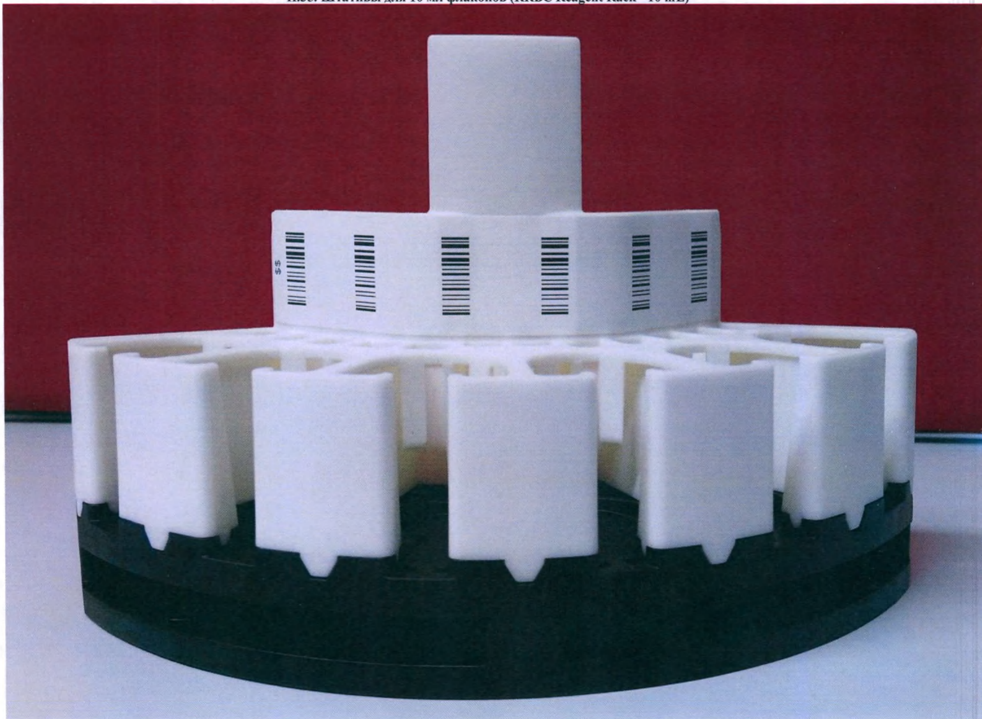
II.35. Штативы для 10 мл флаконов (RRBC Reagent Rack - 10 mL)
