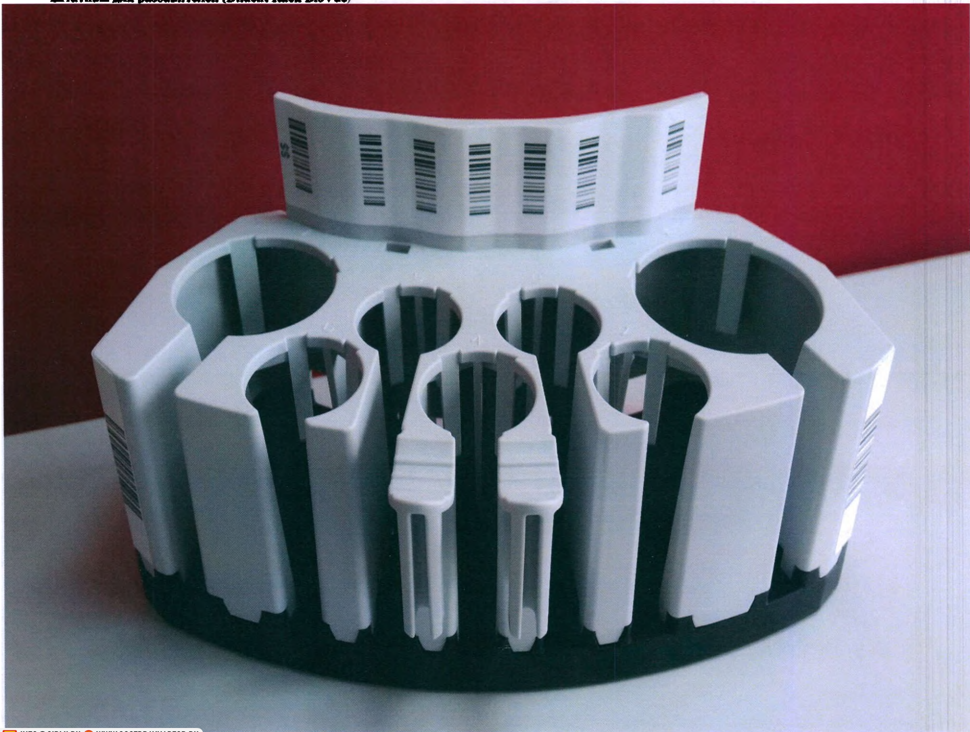
1.56. Штативы для разбавителей (Diluent Rack BioVue)
